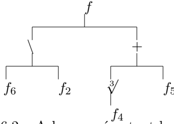
FIGURE 6.2 – Arbre représentant le terme g
