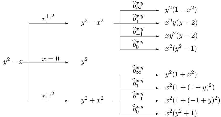
FIGURE 2.1 – Arbre de normalisation
