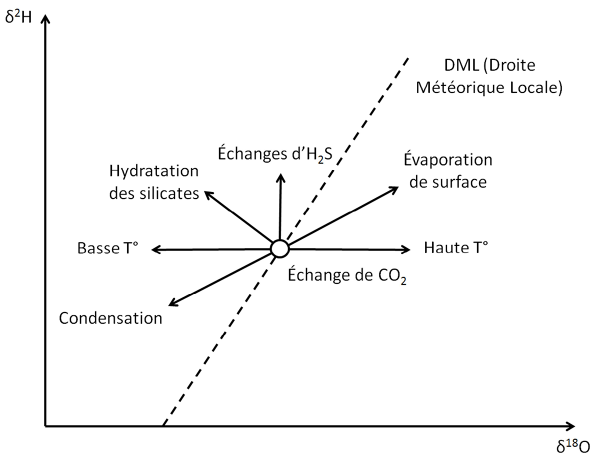
Figure 30 - Processus naturels pouvant influencer sur le fractionnement en ^2\text{H} et ^{18}\text{O} (d'après Clark et Fritz [1997]).
