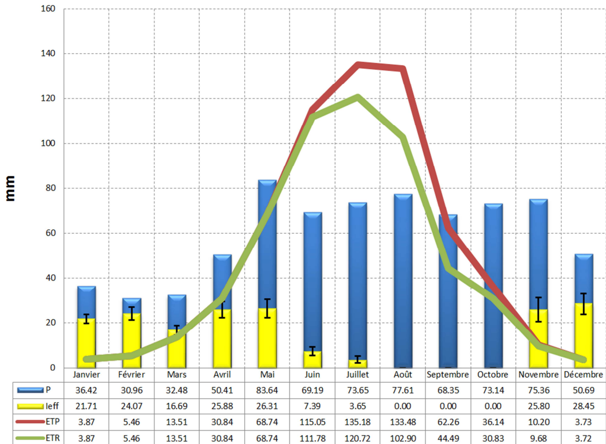
Figure 38 - Bilan hydrique mensuel moyen (moyenne sur 1995-2011) pour un sol dont la RU est de 200 mm de type Chalaïn. Les courbes de couleur rouge et verte correspondent respectivement à l'évapotranspiration potentielle (ETP) moyenne mensuelle et l'évapotranspiration réelle (ETR) moyenne mensuelle. Les histogrammes de couleur bleue et jaune correspondent respectivement à la pluie (P) moyenne mensuelle et l'infiltration efficace (Ieff) moyenne mensuelle. Les barres d'erreur correspondent à l'écart type des valeurs d'infiltration efficace pour les 7 années de considérées.
