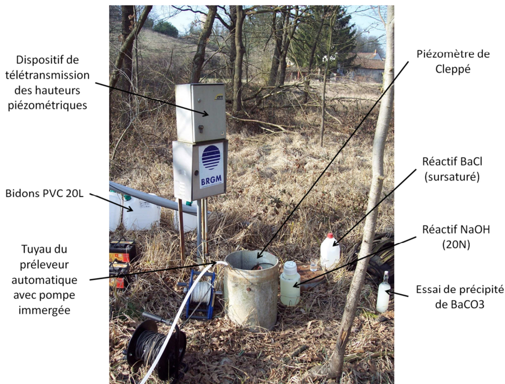
Photo - Dispositif de prélèvement pour l'analyse ^{13}\text{C} et ^{14}\text{C} .
