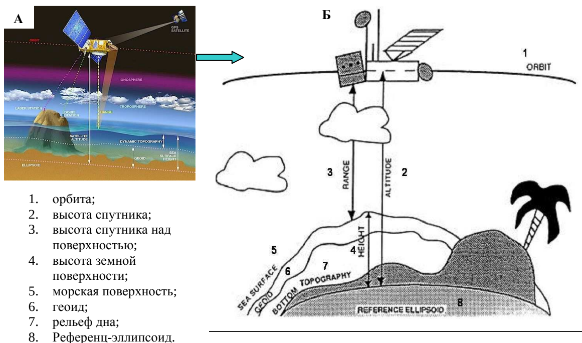
Рисунок 11 – Схема альтиметрических измерений ( www.aviso.oceanobs.com ; Aviso User handbook, 1996); А – общий вид; Б – детально
