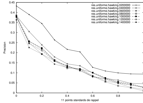
FIG. 4.6 – Rappel/précision pour les 7 sous-collections uniformes de WT10G - modèle de Hawking
