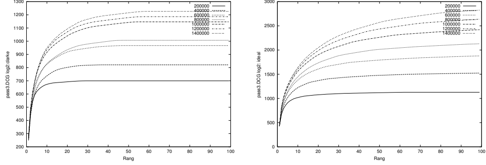
FIG. 5.29 – DCG avec 1/\log_2(\text{rang}) , par taille de collection (modèle de Clarke et cas idéal) jusqu'au rang 100 Schéma (0, 5, 10).
