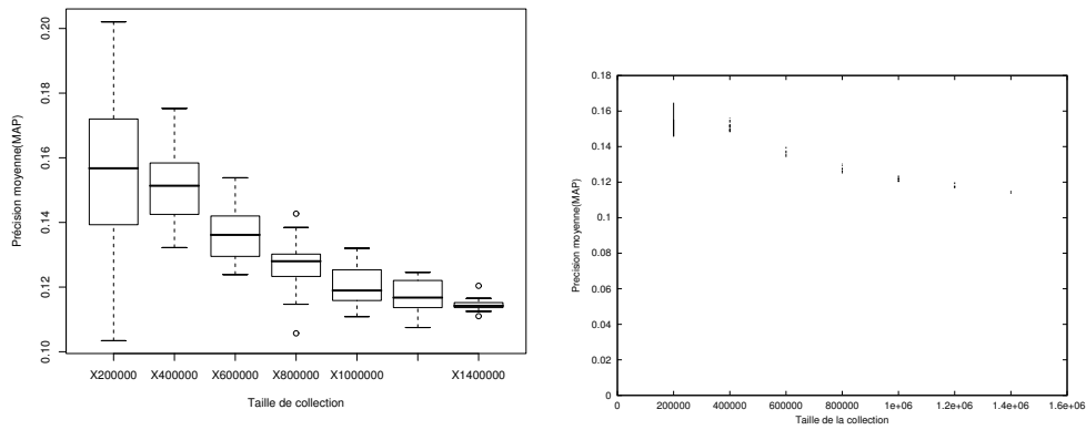
FIG. 4.41 – Box-plot et intervalle de confiance sur MAP : construit à base des 30 sous-collections de chaque taille - Modèle de Hawking
