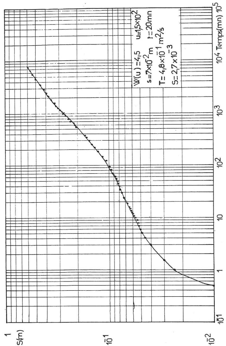
Figure IV 10 : Essai de pompage de Niangon.
