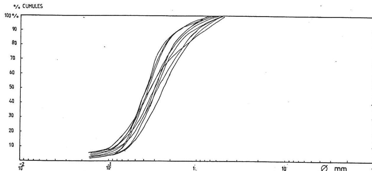
Figure III 23 : Enveloppe granulométrique du niveau 3 du forage IV Sodeci Riviera Centre (continental terminal)
