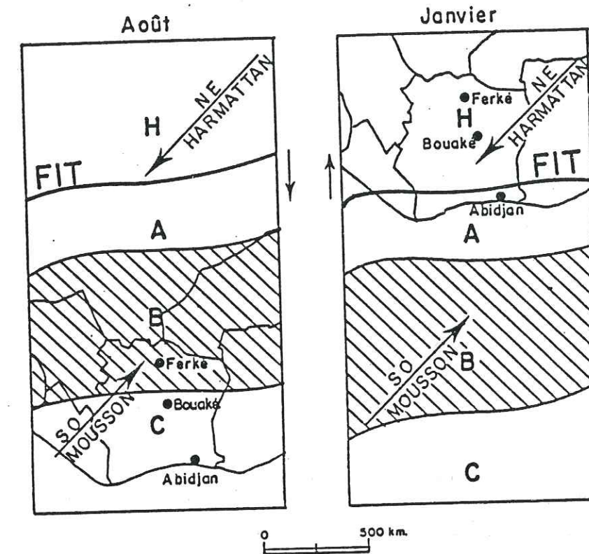
Fig. I 3 : Schéma du Mécanisme des variations climatiques saisonnières
