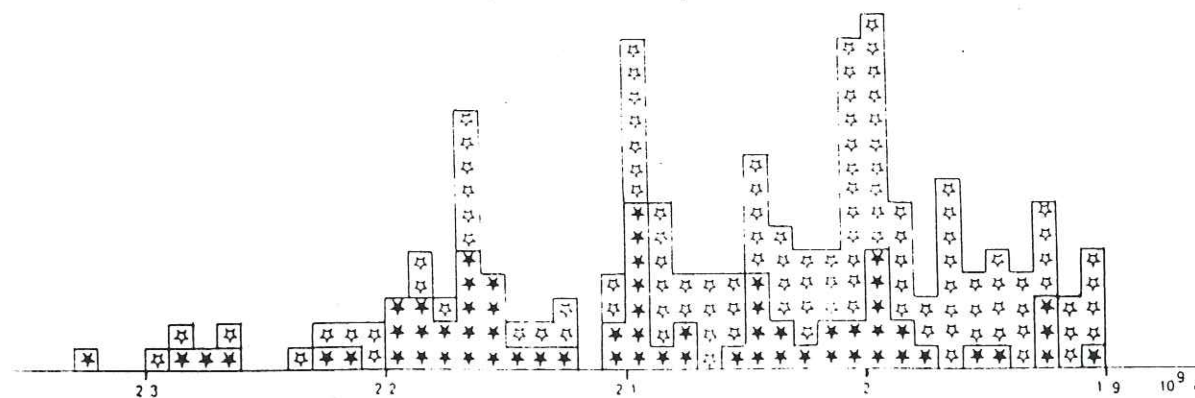
Fig I 9 Histogramme des âges pour la Côte d'Ivoire et le Burkina Faso. Etoiles pleines : âges sur zircons (U/Pb) et par isochrone Rb/Sr sur roches totales ; Etoiles vides : âges Rb/Sr sur minéraux. Tempier, 1986)
