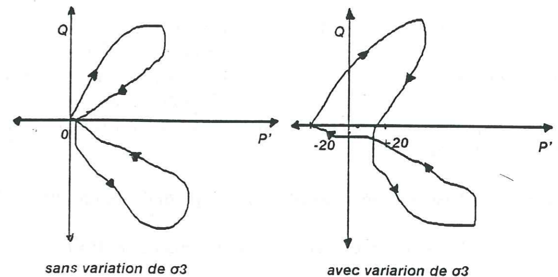
Schéma (V-1): variation des contraintes effectives moyennes au moment de la liquéfaction
