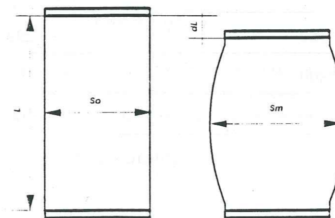
Schéma (IV-2) : Déformation de l'échantillon en forme de tonneau
