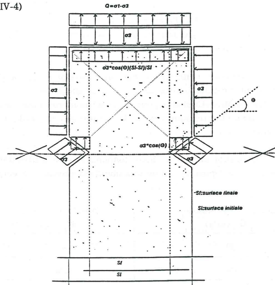
Schéma (IV-4) : effet de la striction sur la contrainte déviatoire (Q)
