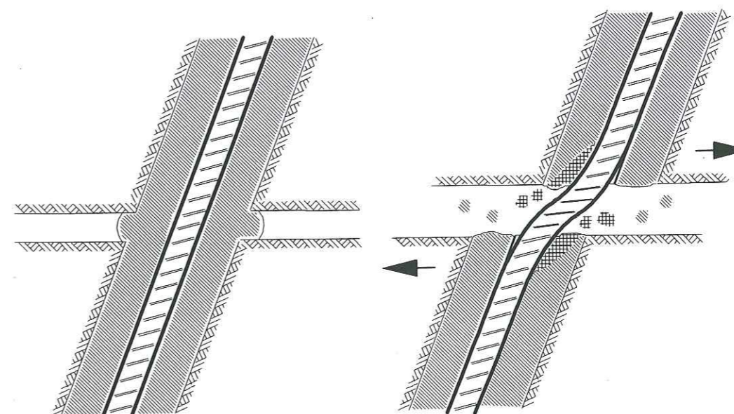
Fig. 5: ancrage passif soumis à un cisaillement du joint
