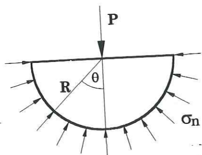
Fig. 6: contraintes au contact de l'armature
