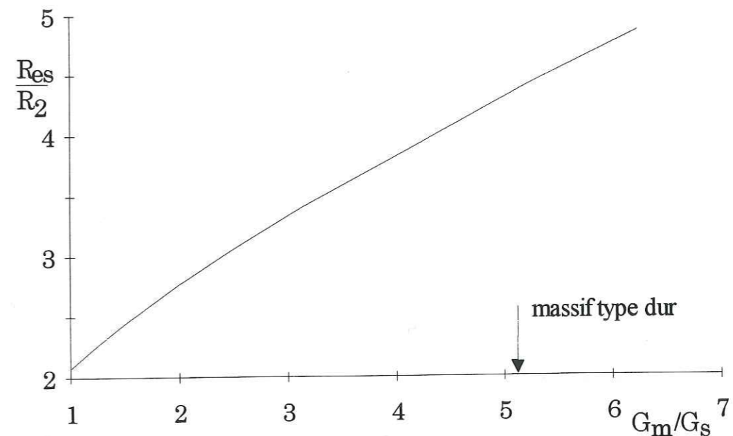
Fig. 14: rayon intérieur du cylindre élastique du scellement, nécessaire pour une stabilité après le début de la rupture du massif
