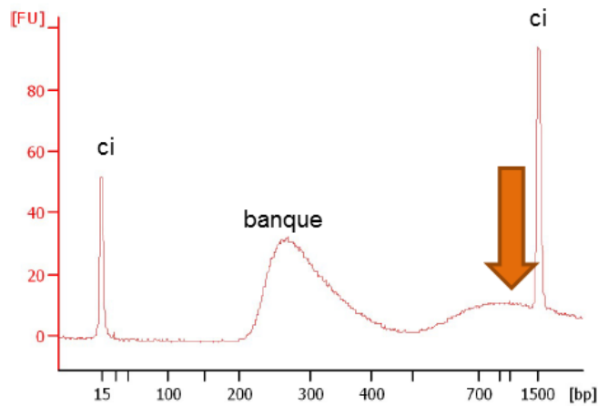
Figure 38 : Analyse sur une puce DNA 1000 de la qualité d'une banque obtenue à partir de 6 µg d'ARN totaux.
