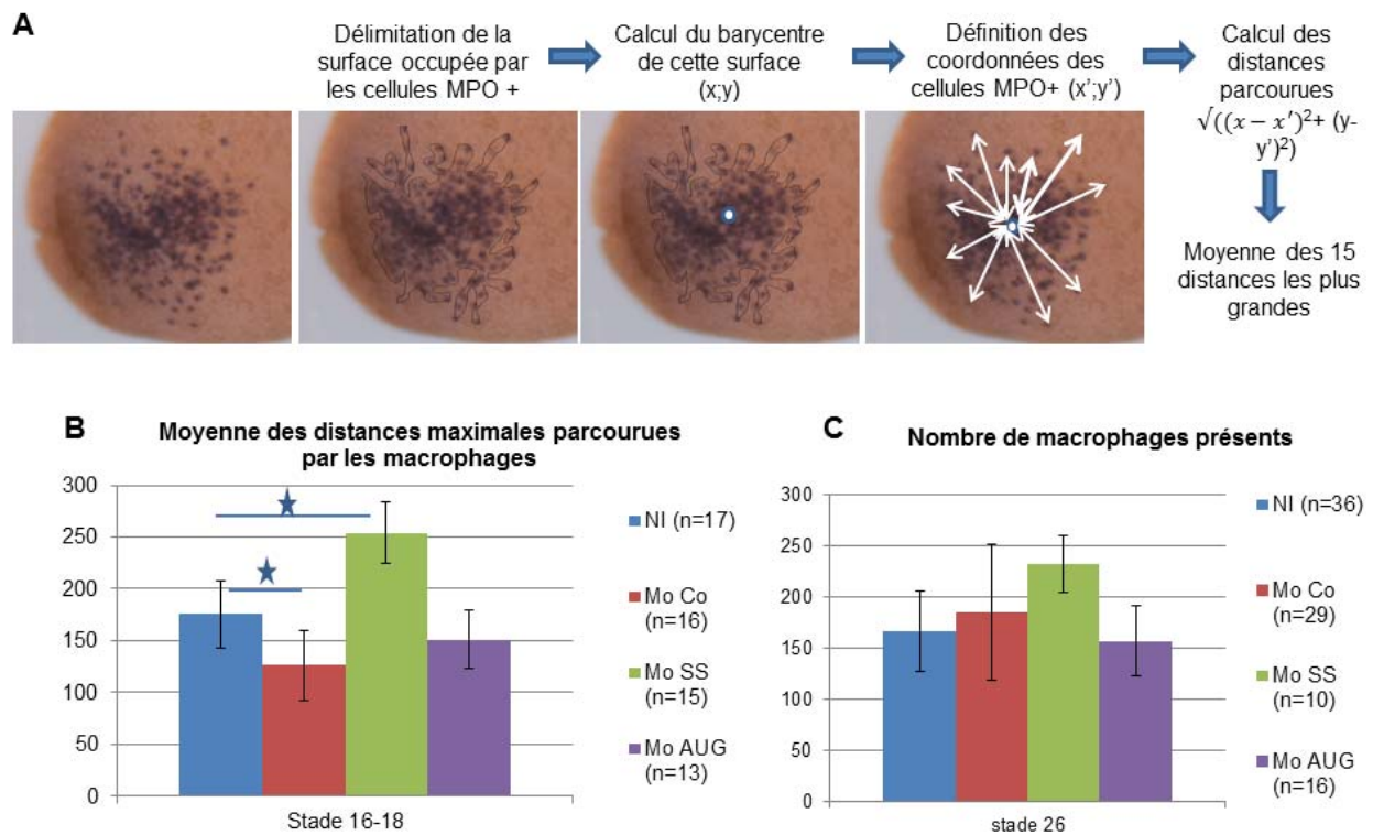
Figure 24 : Phénotype des morphants TTP.
