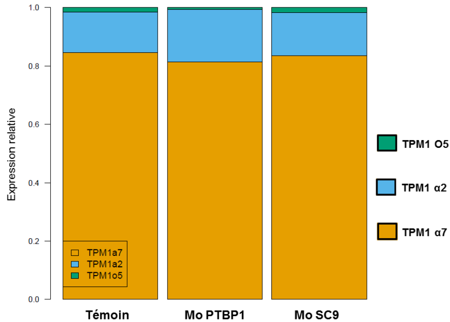
Figure 44 : Expression relative des différents ARNm de la tropomyosine \alpha dans les embryons témoins et les morphants PTBP1 (Mo PTBP1) et EXOSC9 (Mo SC9).
