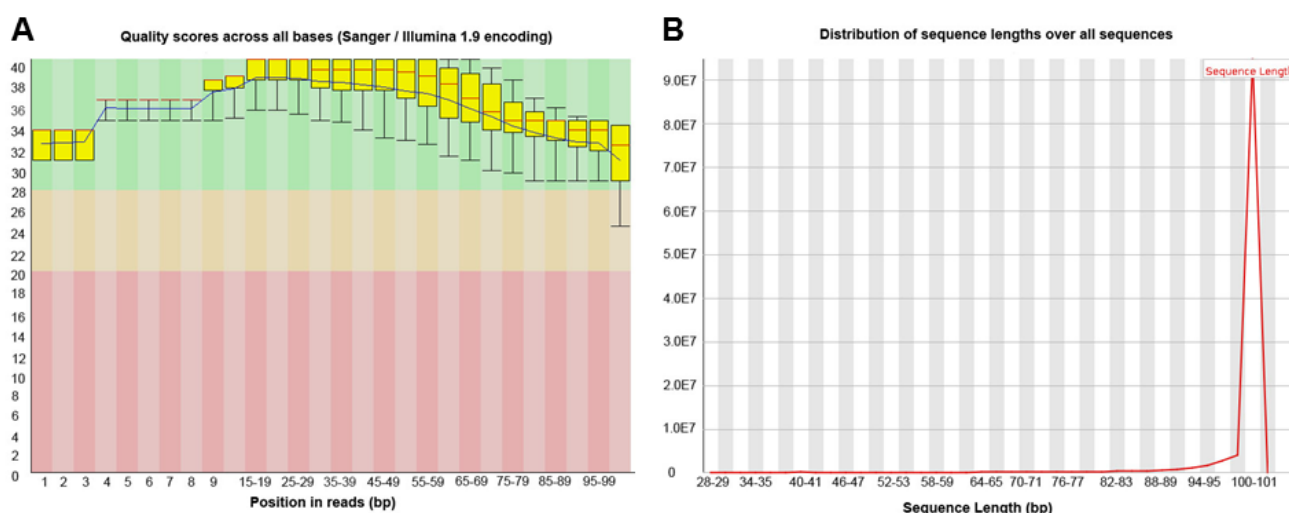
Figure 42 : Analyse de la qualité du séquençage des banques avec le programme FastQC.
