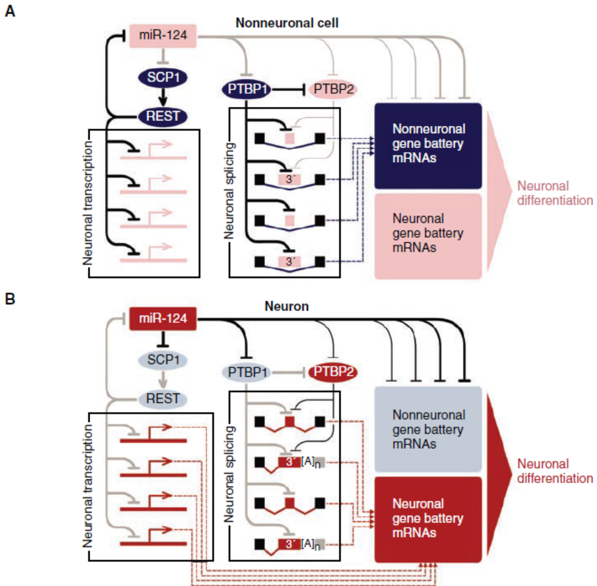
Figure 11 : MiR-124 contrôle un réseau régulateur de gènes
