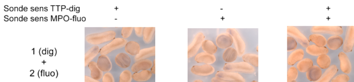
Figure 21 : Co-localisation des cellules exprimant TTP avec les cellules exprimant MPO.
