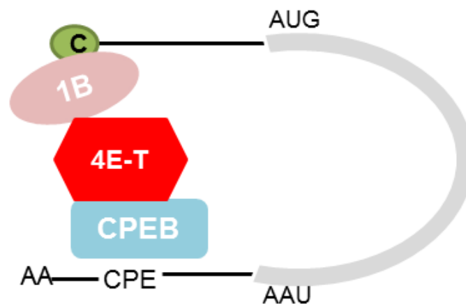
Figure 9 : Modèle de répression de la traduction de l'ARNm Cycline B1 par CPEB dans les ovocytes de xénope.
