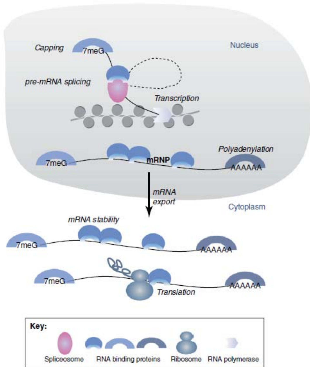
Figure 1 : Les RNA-BP associées aux ARN forment des ribonucléoparticules impliquées dans toutes les étapes de régulations post-transcriptionnelles.
