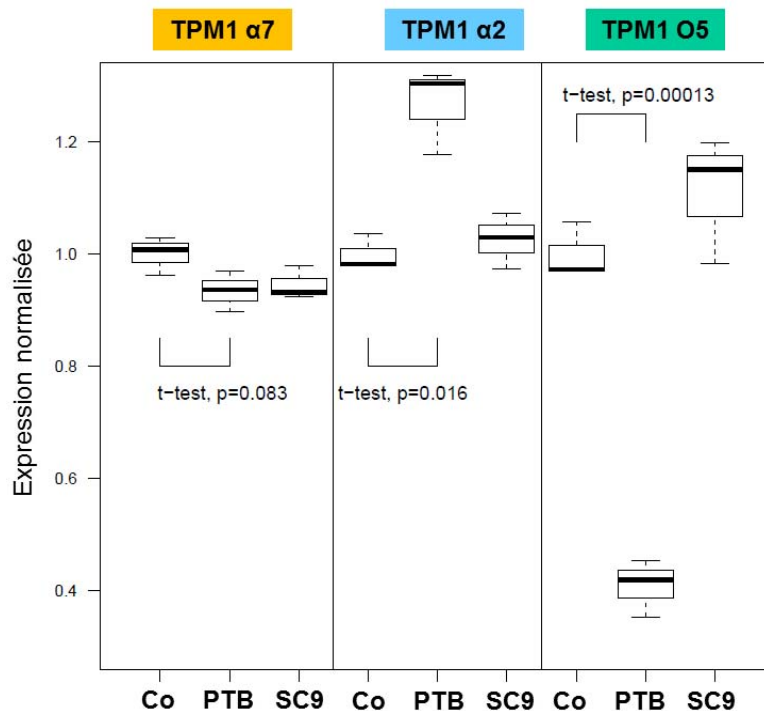
Figure 45 : Expression normalisée des différents ARNm de la tropomyosine \alpha dans les embryons témoins (Co) ou injectés par les morpholinos PTBP1 (PTB) ou EXOSC9 (SC9).
