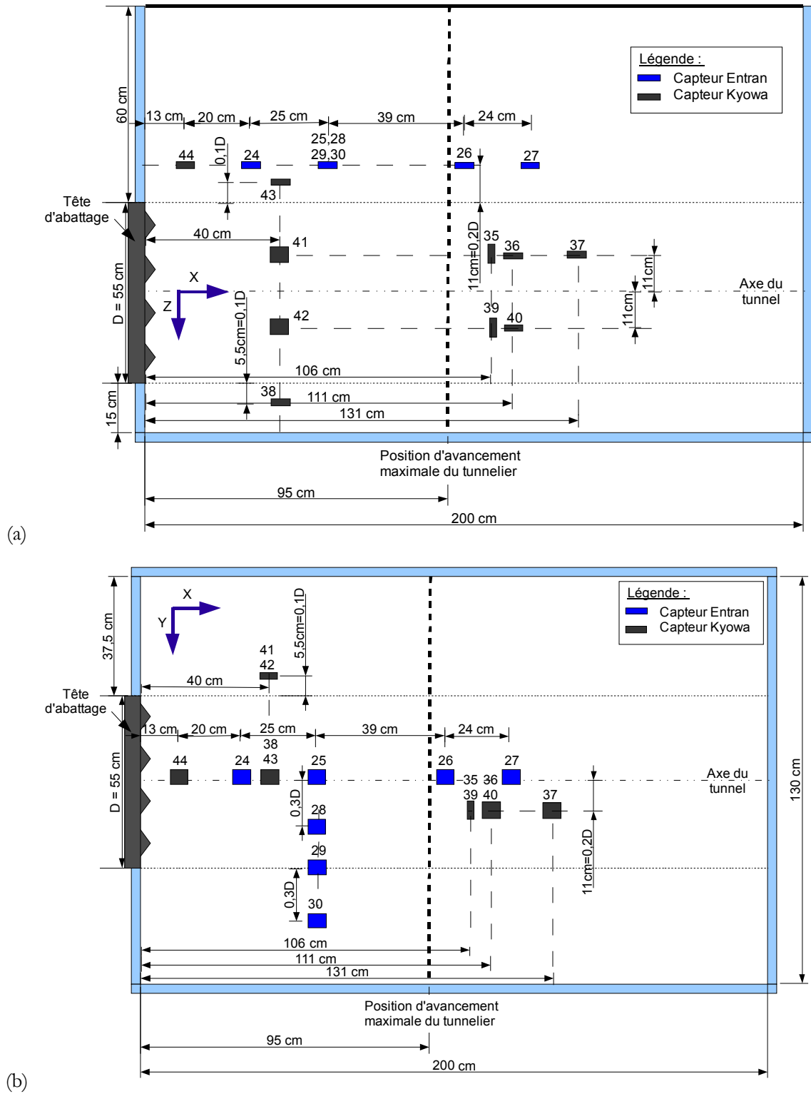
Figure Annexes 10 : Positions des capteurs de contraintes lors des essais MS2 et MS3 (vue de côté (a) et vue de dessus (b) du caisson).
