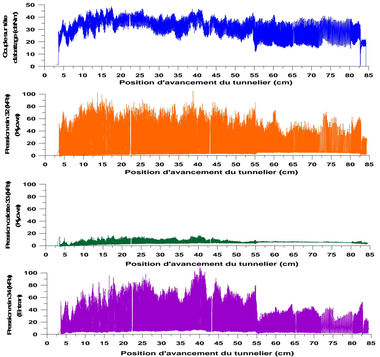
Figure Annexes 15 : Evolutions du couple sur la roue de coupe et des pressions dans la chambre d'abattage au cours de l'essai MC8.
