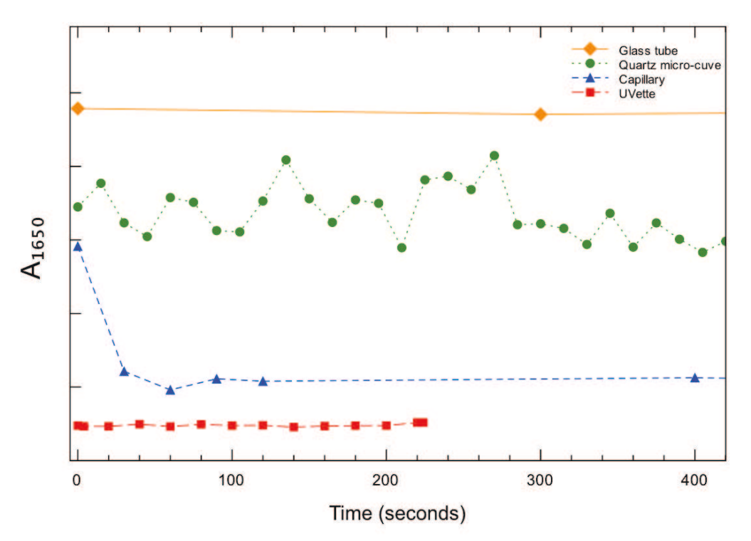
Figure II-8 : Stabilité au cours du temps du signal SERRS d'un échantillon de Rup(R6G) 3 en concentration 8,7 \times 10^{-7} \text{ M} dans différents contenants.
