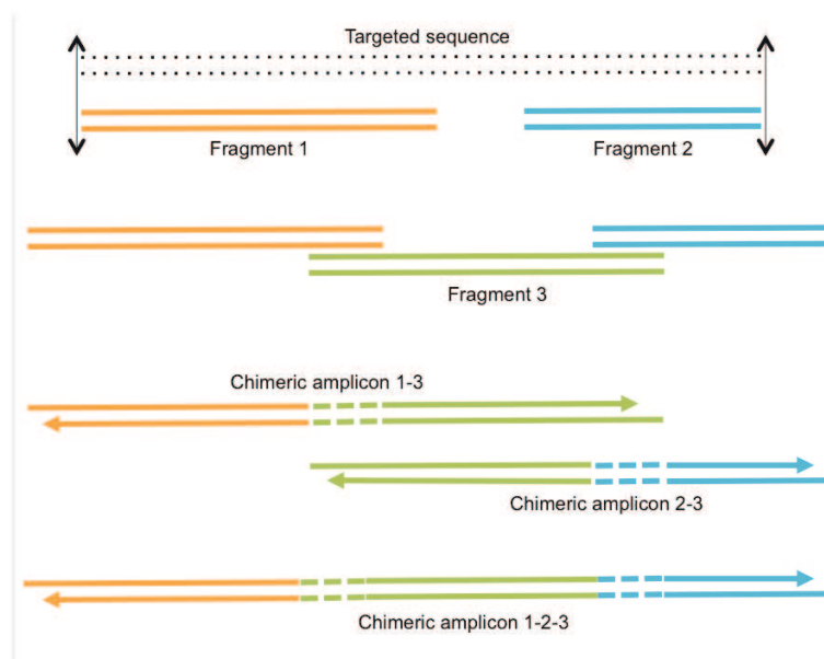
Figure I-7 : Jumping PCR, artéfact d'amplification fréquent dans l'étude d'ADN ancien (d'après Pääbo et al., 1990 et Orlando et Hänni, 2000). Le fragment ciblé n'est pas forcément présent dans l'échantillon. L'ADN polymérase va donc créer des molécules chimères en combinant plusieurs fragments qui se recoupent. Le résultat d'amplification peut par conséquent être plus long que la séquence ciblée.
