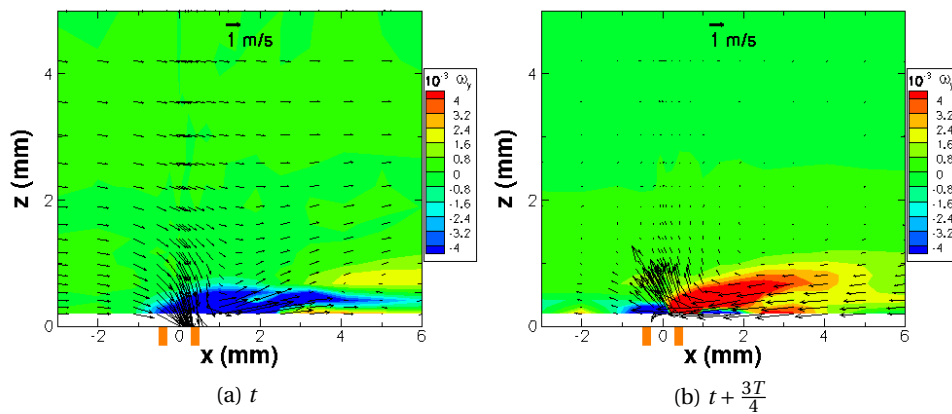
FIGURE I.9 – Champs de vitesse acoustique (flèches) et de vorticit  (couleurs) au-dessus d'un r sonateur. T est la p riode acoustique. LDV, 1592 Hz, excitation 140.5 dB, M_b = 0.1 (source : [121]).
