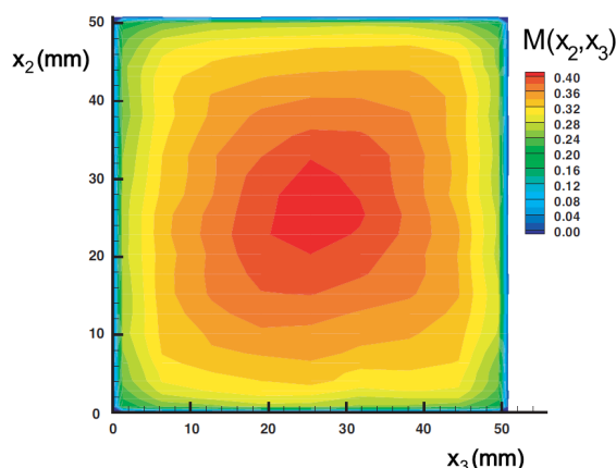
FIGURE I.14 – Vitesse d'écoulement mesurée par sondes Pitot dans le NASA GIT (d'après Jones et al. [66])
