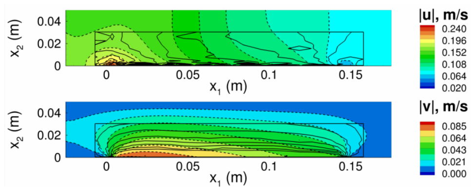
FIGURE V.21 – Comparaison de l'amplitude de vitesse acoustique longitudinale (haut) et transversale (bas) mesurée par LDV (banc B2A traité par matériau microperforé) et reconstruite avec le solveur GD à partir des paramètres identifiés, à f = 1992 Hz. Les mesures LDV (contours pleins) sont superposées aux résultats numériques (couleurs et contours pointillés) dans la zone de mesure représentée par le rectangle noir.
