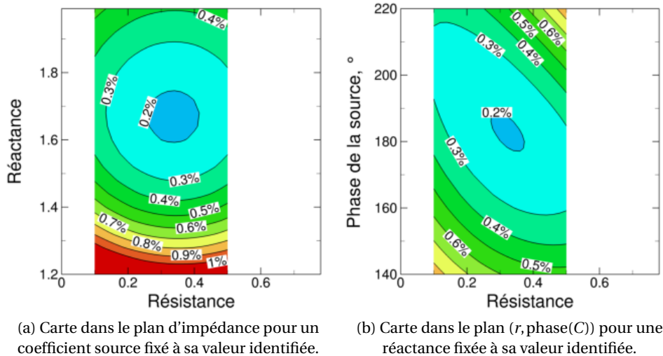
FIGURE V.6 – Cartes de fonction objectif adimensionnée \mathcal{J}_{\text{red}} à f = 2488 Hz.
