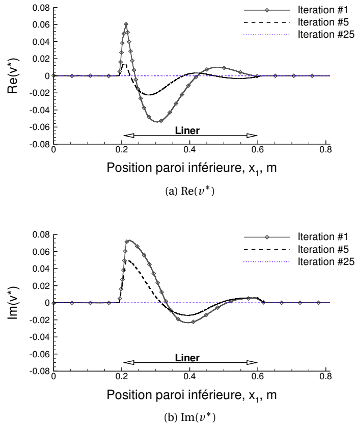
FIGURE VII.11 – (a) Partie réelle et (b) partie imaginaire de la vitesse adjointe transversale sur la paroi inférieure (parties rigides et partie traitée)
