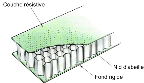
FIGURE I.2 – Liner à un degré de liberté (SDOF)
