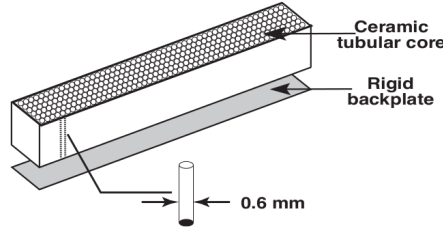
FIGURE IV.4 – Matériau tubulaire céramique CT57
