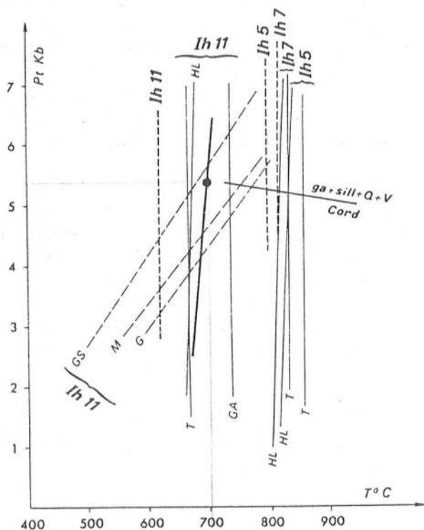
Fig. 2. Estimation P , T des assemblages minéralogiques des gneiss à cordiérite et grenat à partir des géothermomètres. Traits fins: couple grenat-biotite; tirets fins: couple grenat-plagioclase; tirets épais: couple cordiérite-grenat; ligne épaisse: assemblage à sept phases, point: position du gneiss rubané Ih 11 sur cette ligne; grenat + sillimanite + quartz + vapeur \rightleftharpoons cordiérite pour X_{\text{Fe}} \text{ cordiérite} = 0,25 et PH_2O = 0,4 P_T (Lee et Holdaway, 1977); voir Tableau III pour les références des données thermodynamiques. Fig. 2. P , T field for assemblages from cordierite and garnet gneisses using the geothermobarometers. Thin lines: garnet-biotite; thin dashed lines: garnet-plagioclase; heavy dashed lines: cordierite-garnet; heavy line and spot: univariant seven-phase assemblage and position of the banded gneiss Ih 11; garnet + sillimanite + quartz + vapor \rightleftharpoons cordierite with X_{\text{Fe}} \text{ cordierite} = 0.25 and PH_2O = 0.4 P_T (Lee and Holdaway, 1977). References on thermodynamic data are given in Table III.
