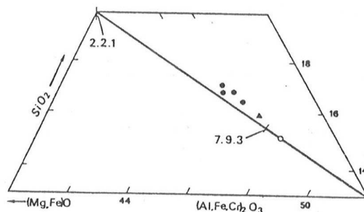
FIG. 7. — Position des saphirines des amphibolites d'Anavoha (o), de Marolinta (A) et de l'anorthosite (o) dans une portion du système ternaire (Mg, Fe)O-(Al, Fe, Cr) 2 O 3 -SiO 2 (Higgins et al. , 1979).
