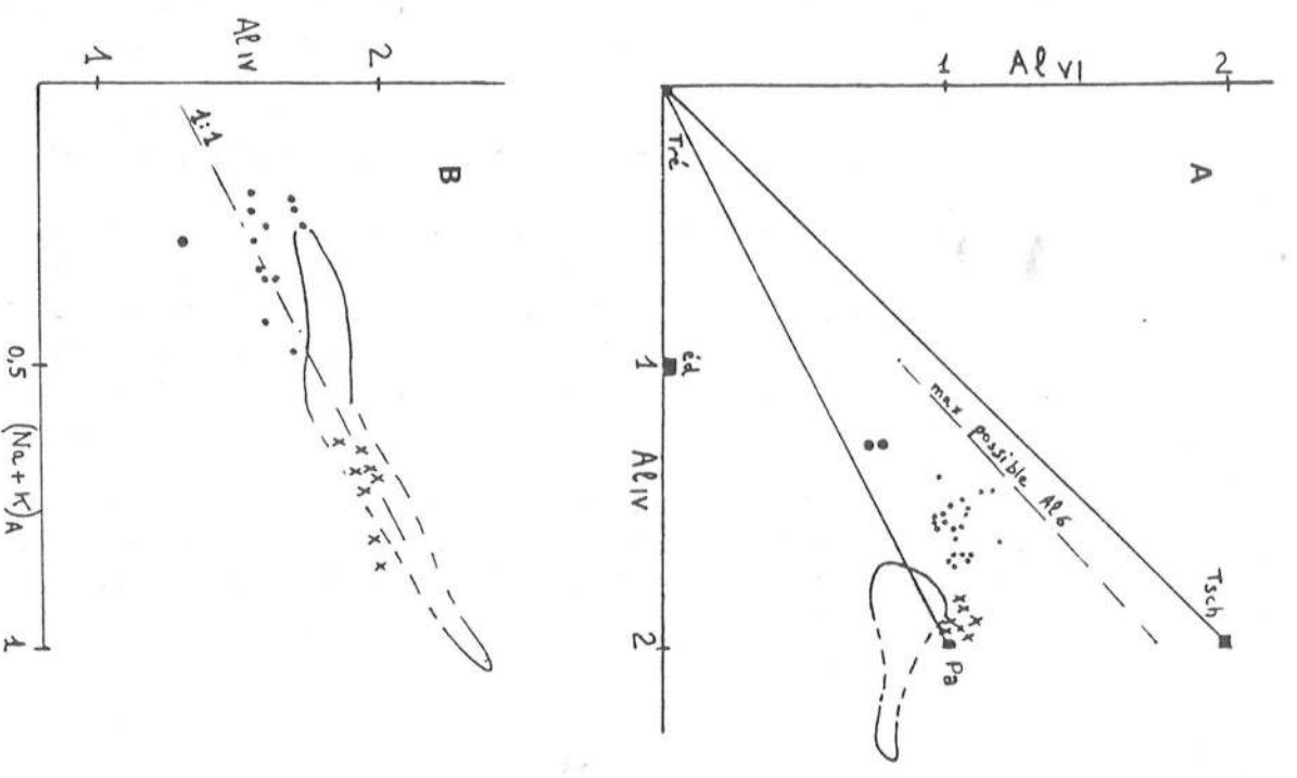
Figure 13 - Diagrammes AlVI en fonction de AlIV (A) et AlIV en fonction de la somme des alcalins en site A (B) des pargasites des métatrocloites (x) et des hornblendes des amphibolites à Sa-Co (.) (gros points : amphibolite biminérale A 14). Le domaine des amphibolites à Sa-Co du Haut Allier (Brand, 1981) est également indiqué. Limite du maximum possible d'Al 6 : Leake (1971).
