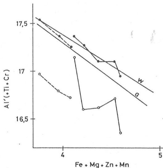
FIG. 9. — Al' (=Al+Si-8) ( \circ ) et Al'+Ti+Cr ( \bullet ) versus Mg+Fe+Mn+Zn pour les staurotides de l'anorthosite d'Anavoha (ligne pleine) et pour les staurotides chromifères de Fiordland (ligne pointillée; Ward, 1984). "Lignes de probabilité maximale" de Griffen et al. , 1982 : (G) et de Ward, 1984, calculée par Grew et Sandiford, 1985 : (W).
