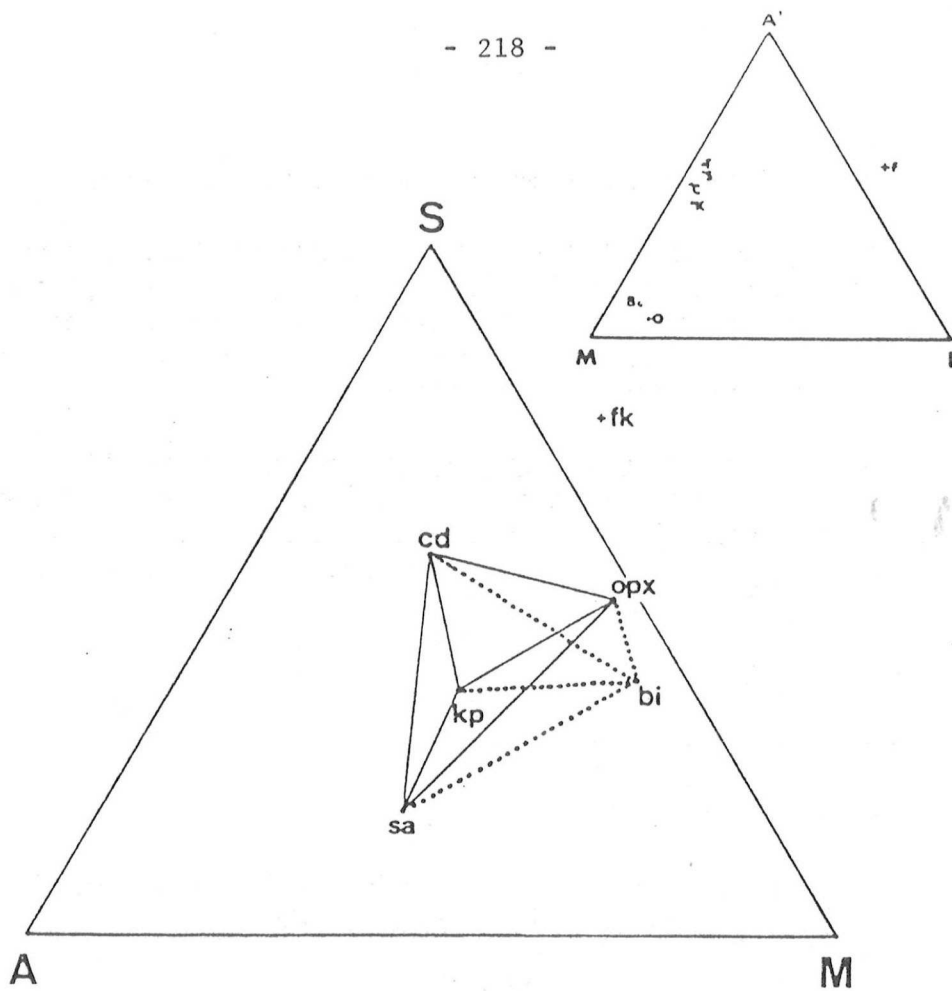
Figure 5 - Représentation des minéraux des gneiss biotitiques à kornéropine dans un diagramme \text{SiO}_2\text{-Al}_2\text{O}_3\text{-Mg(Fe)O-K}_2\text{O} (- \text{B}_2\text{O}_3 et \text{H}_2\text{O} en excès) ; projection à partir du feldspath potassique. Les lignes jointives pleines sont sur la base SAM du tétraèdre, tandis que les lignes pointillées sont projetées. Le triangle A'FM (projection à partir du Fk) met en évidence les faibles variations du rapport XMg des différents minéraux.
