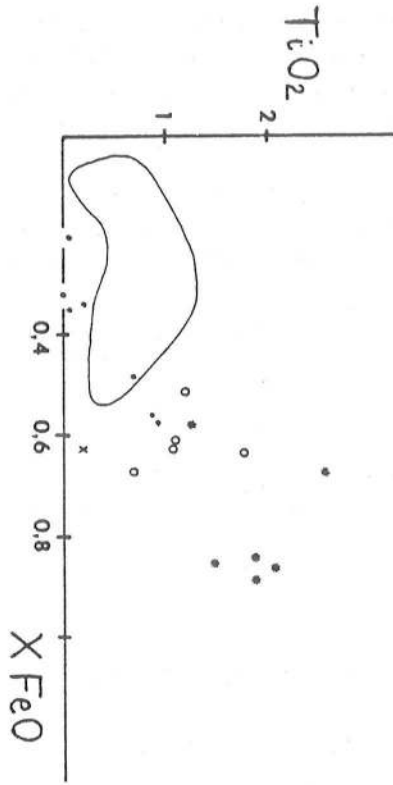
Fig. 6 - Diagramme TiO_2 versus X FeO des roches ultrabasiques et basiques avec (*) ou sans (.) grenat (x : notrite) et des granulites à Opx et Oamph-Cord (o) de la formation d'Andriamena. Le domaine représenté inclut les pelites magnésiciennes à Oamph-Cord de Queensland (Reinhardt, 1987).
