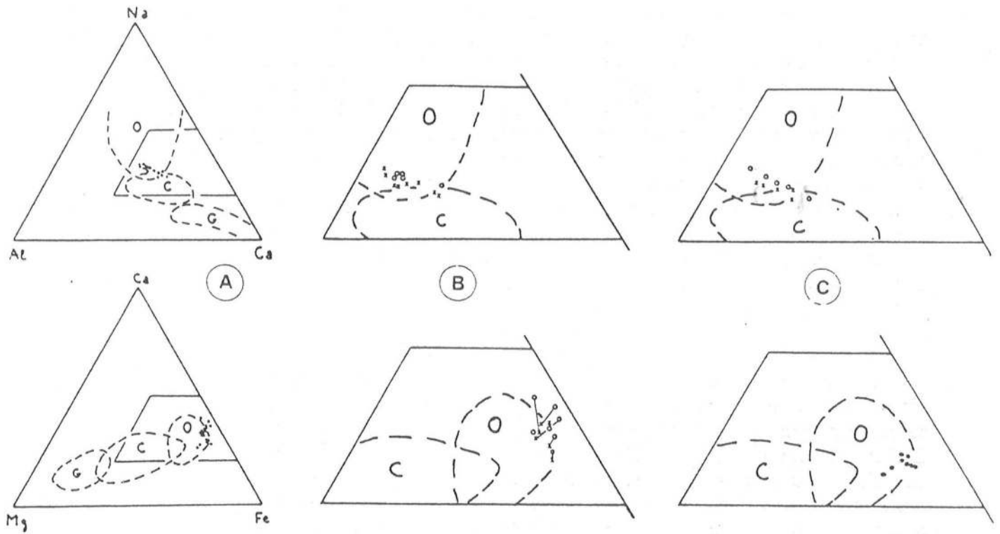
Fig. 1 - A : Compositions des clinopyroxènes de l'éclogite de Faratsiho dans un diagramme Na-Al-Ca. Champs des clinopyroxènes des différents types d'éclogites de Smulikowski (1972) : G : clinopyroxènes des Griquaites ; C : clinopyroxènes des éclogites des formations gneissiques et migmatiques (= HT) ; O : clinopyroxènes des éclogites "ophiolitiques" ou "de type alpin" (= HP-BT) ; I-B : agrandissement du trapèze de la Fig. 1-A pour les cristaux de la zone granoblastique : coeurs (o) et bordures (x) des cristaux ; I-C : même chose pour les omphacites de la fissure centrale (x) et pour les inclusions (o) dans les gros grenats.
