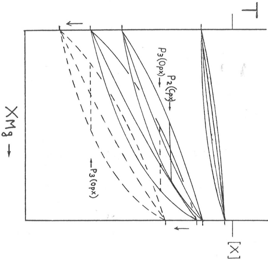
Figure A5 - Diagramme T-XMg polyphare, dessiné à partir de la fig. 9, permettant d'estimer les rapports XMg des minéraux des réactions univariantes stables dans cette figure. P2 (Cpx) : compositions des minéraux de la réaction [Cpx] à la pression P2. La loupe en tiret illustre le déplacement de la réaction [Opx] lors d'une diminution de PH 2 O et, par voie de conséquence, les variations de la T°C et de la composition des minéraux à P3 (Opx) constante. Même échelle de T°C sur tous les diagrammes T-X et P-T.
