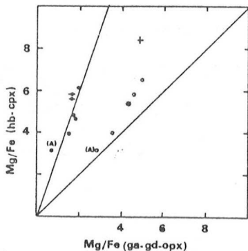
FIG. 6. — Répartition magnésium-fer des couples : opx-cpx (+) et opx-hb (*) dans les métatroctolites, hb-gd (o) dans les amphibolites à corindon et dans l'anorthosite d'Anavoha (A), hb-ga dans les métatroctolites (o) et dans les amphibolites et anorthosite d'Anavoha (o) ; lignes : Kd=1 et 3.
