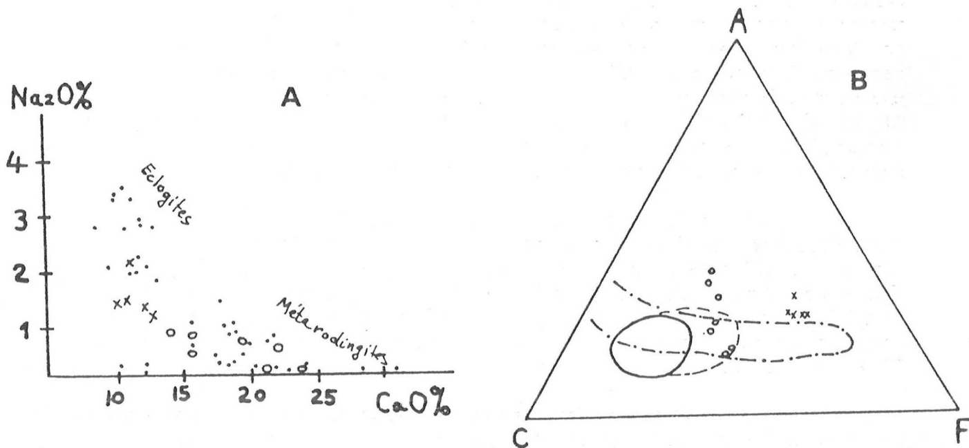
Fig. 3 A - Corrélation inverse entre Na 2 O et CaO dans les amphibolites à Sa-Co (et métatroctolite coronitique : x) et les clinopyroxénites (o) comparée à celle des écloğites et métarodingites de la Cima de Gagnone (., Evans et al, 1979).
