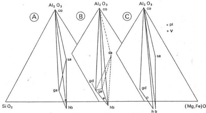
FIG. 10. — Projection à partir de l'anorthite sur le plan SiO_2-Al_2O_3-(Mg,Fe)O du système SiO_2-Al_2O_3-(Mg,Fe)O-CaO-(H_2O) . Anavoïa : A) Echantillon 52 (minéraux et roche totale : ●) ; B) Echantillons 54b (minéraux) et métatroctolite AI (roche totale : ■) ; lignes pointillées : assemblage relictuel (?) Marolinta : C) Echantillons 50a (minéraux) et 50b (minéraux et roche totale : o).
