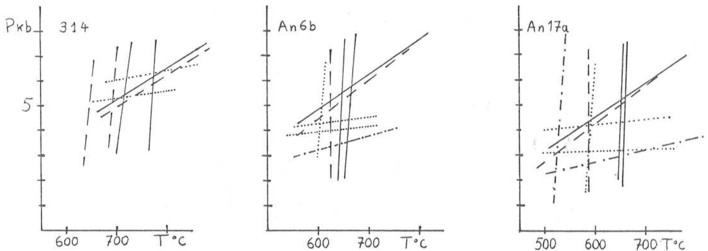
Fig. 2 - Estimations des conditions thermodynamiques d'équilibre d'une granulite ferrugineuse de Farafangana (éch. 314) et de deux métabasites à grenat de la formation d'Andriamena (éch. An 6b et An 17a).
