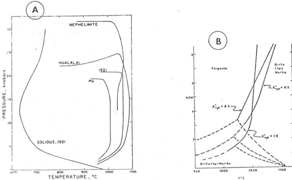
Fig. 22 - A : Limite de stabilité de l'amphibole dans les magmas basiques avec \text{PH}_2\text{O} = \text{PT} et dans les conditions de fugacité de l'oxygène des tampons FMQ et NNO ; B : même chose pour la pargasite pour différentes fractions molaires de l'eau dans un fluide \text{H}_2\text{O} - \text{CO}_2 ( in Veblen et Ribbe, 1982).
