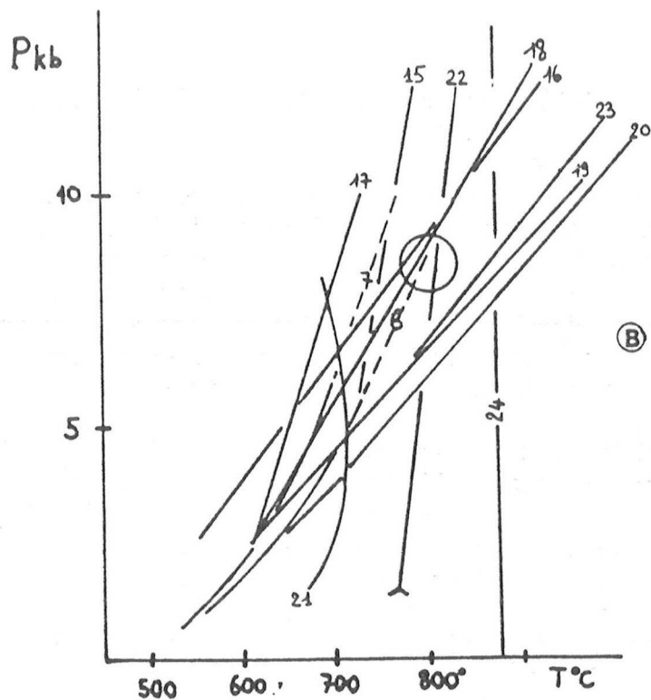
Fig. 2 B - Evaluation Pression-Température de formation des clinopyroxénites à Ga ou Zo (cercle : estimation moyenne) PH 2 O = Pt, sauf pour les réactions (6) et (7). Le membre droit des réactions suivantes est stable à haute température.
