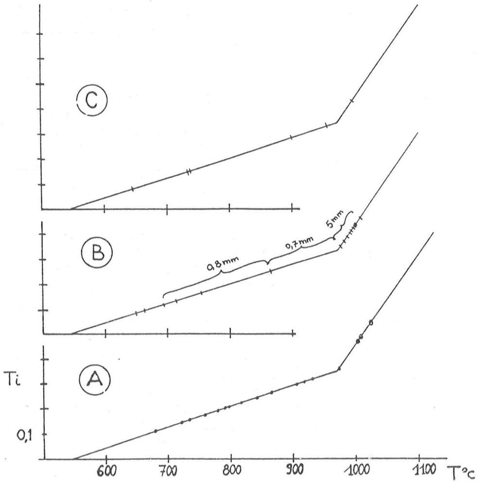
Fig. 14 - Géothermomètre Ti dans l'amphibole (Oren, 1984). A : granulites ( ) et métatucociolites d'Anabohitsy (o) ; B : amphibole zonée de la métatucociolite d'Anatafisa (éch. 250) ; C : amphibole zonée du leucogabbro d'Anabohitsy (éch. 172 l).
