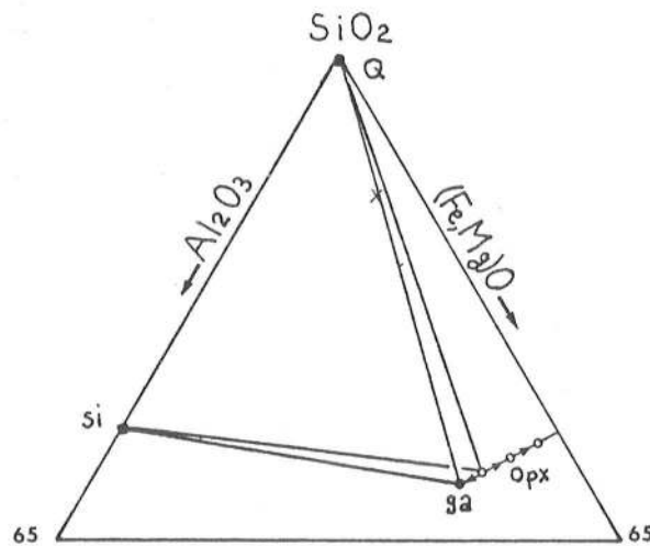
Fig. 3 - Diagramme SiO 2 - Al 2 O 3 - (Mg, Fe)O montrant l'évolution de l'orthopyroxène alumineux le long d'une ligne reliant le grenat au point représentatif du pyroxène sans alumine sur la ligne SiO 2 - (Mg, Fe)O au cours de la réaction Al Opx = Opx + Ga. Les lignes jointives relient les minéraux de la paragenèse initiale à Al Opx - Ga - Q ± Sill (celles-ci se coupent car MgO et FeO sont des constituants indépendants). Minéraux (• : Ga, Sill, Q ; o : Opx) et roche totale (x) de l'échantillon An4c.
