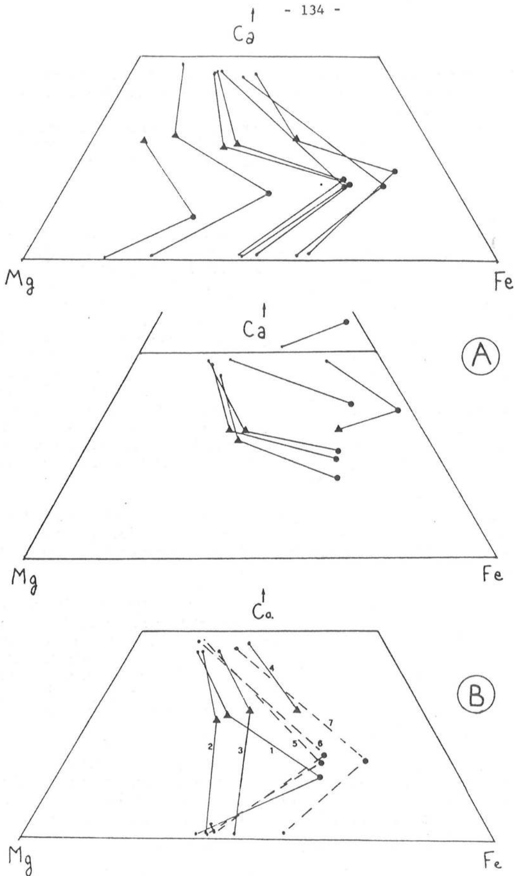
Fig. 6 - Compositions des minéraux ferromagnésiens dans le triangle Ca - Mg - Fe ++ (pourcentages atomiques).
