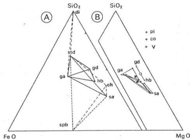
FIG. 11. — Projection à partir de l'anorthite sur le plan SiO_2-FeO-MgO dans le système SiO_2-Al_2O_3-MgO-FeO-CaO-(H_2O) . Al_2O_3 et H_2O sont en excès. A) Anorthosite d'Anavoïa ; lignes pointillées : réactions possibles d'apparition et de disparition de la staurolite ; B) Amphibolites (minéraux : Anavoïa : 54b, A7, A9 ; Marolinta : 50a, 50b ; roches : voir figure 10).
