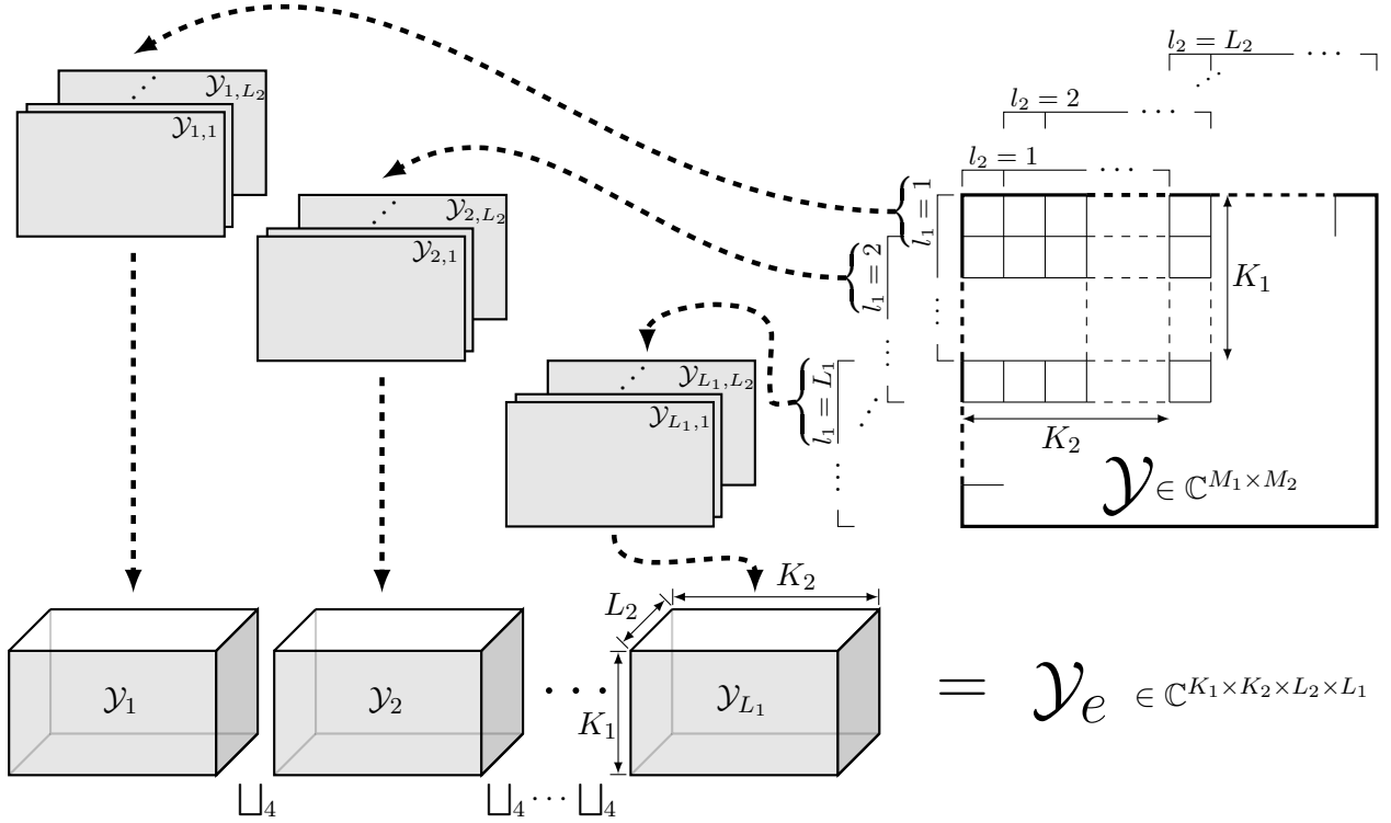
FIGURE 2.4 – Construction du tenseur d'ordre augmenté pour un signal bi-dimensionnel \mathcal{Y} de dimension M_1 \times M_2 .
