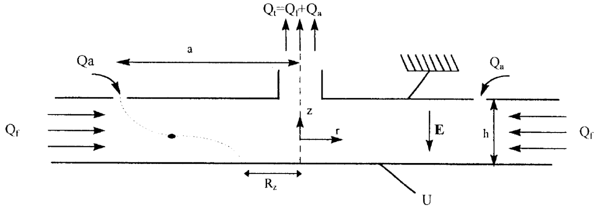
Figure 2.1 : Le SMEC à dépôt (Mesbah, 1993).
