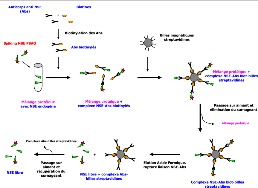
Fig. 3.2 Stratégie d'immuno-capture de la protéine NSE [58].
