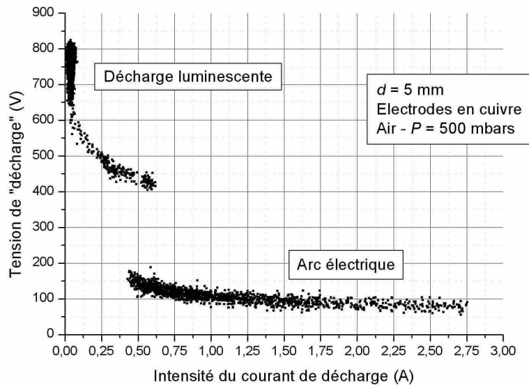
Figure 3.10 : Caractéristique U/I pour P = 500 mbar, d = 5 mm
