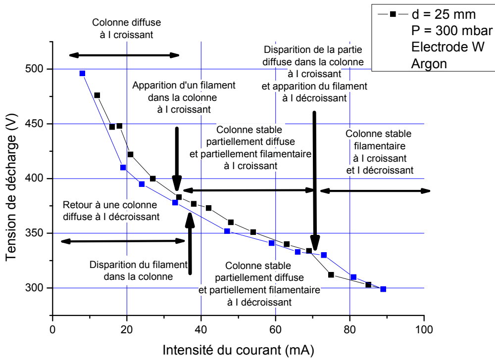
Figure 3.29: Exemple de caractéristique U/I zoomée autour de la zone de contraction de la colonne pour P = 300 mbar, d = 25 mm. Points noirs : I croissant ; points bleus : I décroissant.
