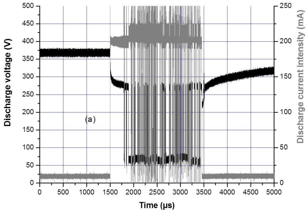
Figure 3.15 : Évolution au cours du temps de la tension de décharge et de l'intensité de décharge lors de l'application d'un pulse d'intensité environ égale à 200 mA ( P = 100 mbar et d = 25 mm)
