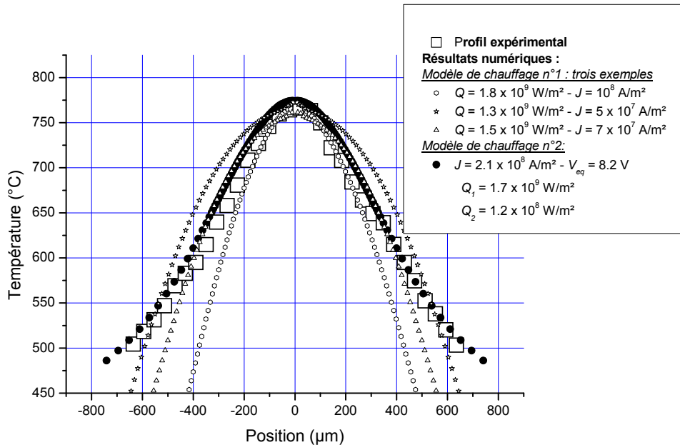
Figure 6.16: Rappel des résultats expérimentaux et des résultats numériques obtenus avec le modèle de chauffage n°1. (présentés figure 6.7). Comparaison avec les résultats numériques obtenus dans le cas d'un chauffage dû à un flux supplémentaire (modèle de chauffage n°2).
