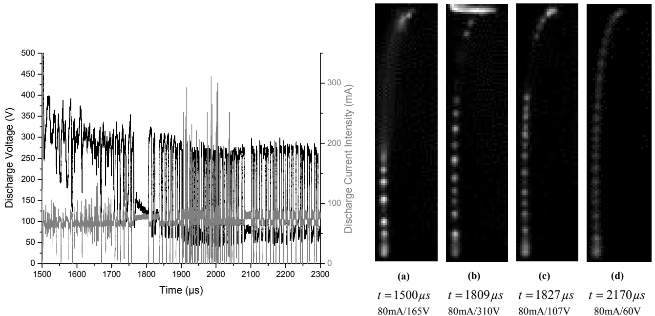
Figure 3.34 : Partie de gauche : Évolution en fonction du temps de la tension entre les électrodes et de l'intensité de la décharge. P = 100 mbar ; d = 25 mm.
