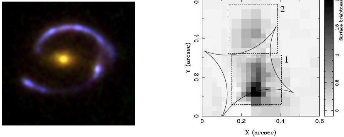
FIGURE 2.2 – A gauche, image à haute résolution de l’œil cosmique obtenue par le télescope Hubble en combinant les filtres visible (caméras ACS et WFPC2) et proche-infrarouge (caméra NICMOS). A droite, reconstruction de la source d’origine en corrigeant de l’effet de lentille (Dye et al., 2007) : on distingue deux composantes (marquées par 1 et 2) avec une amplification différente.
