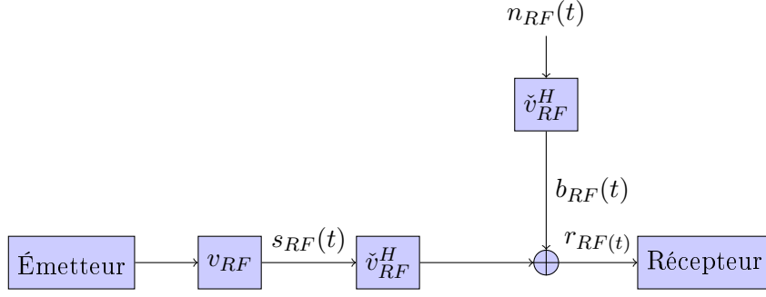
(b) Filtrage passe-bande en émission et bande équivalente de bruit.
