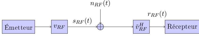
(a) Filtrage passe-bande en émission-réception.
