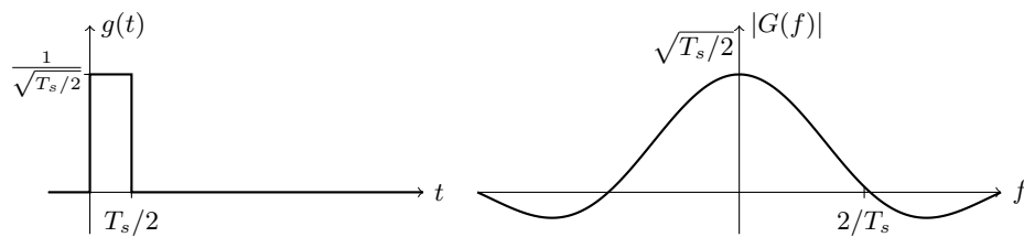
FIGURE 1.7 – Fonction prototype RZ.
