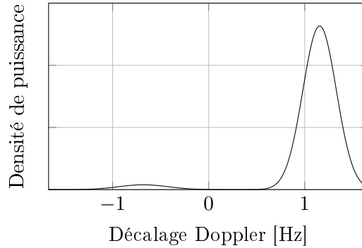
(c) Spectre Doppler des trajets 5 et 6.
