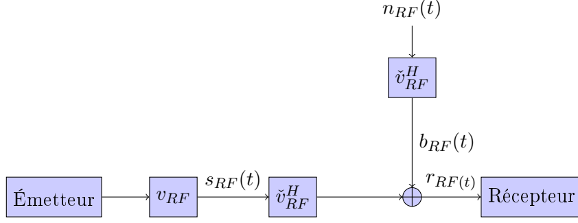
(b) Fitrage passe-bande en émission et bande équivalente de bruit.
