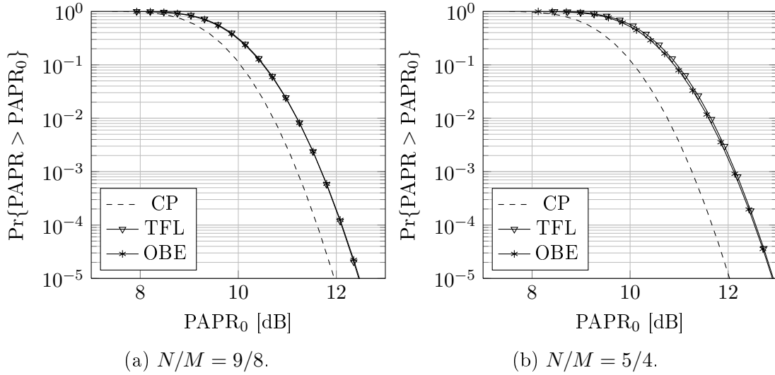
FIGURE 4.15 – Estimation de la fonction de répartition complémentaire du PAPR pour différents prototypes avec M = 1024 .
