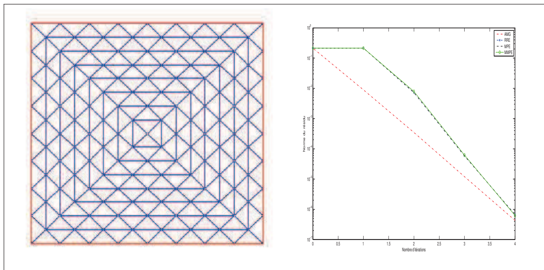
FIGURE 5.5 – Cas d'un maillage uniforme ( N = 145 )
