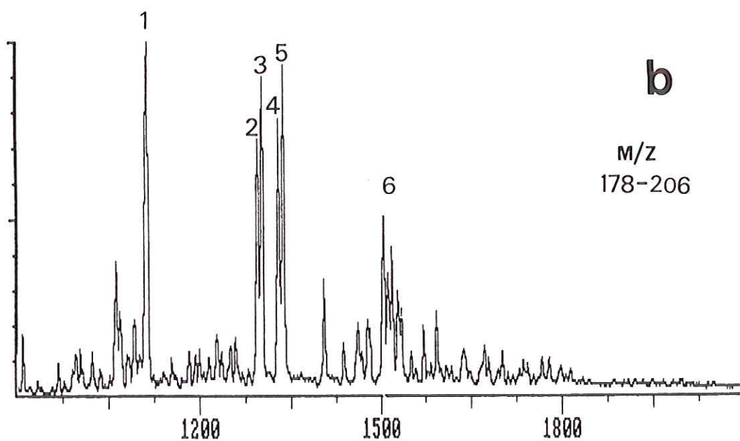
Fig. 50 : Exemples de distribution des composés de la famille de phénanthrènes trouvés à Anou-Ararène (a) et Sékiret (b).
