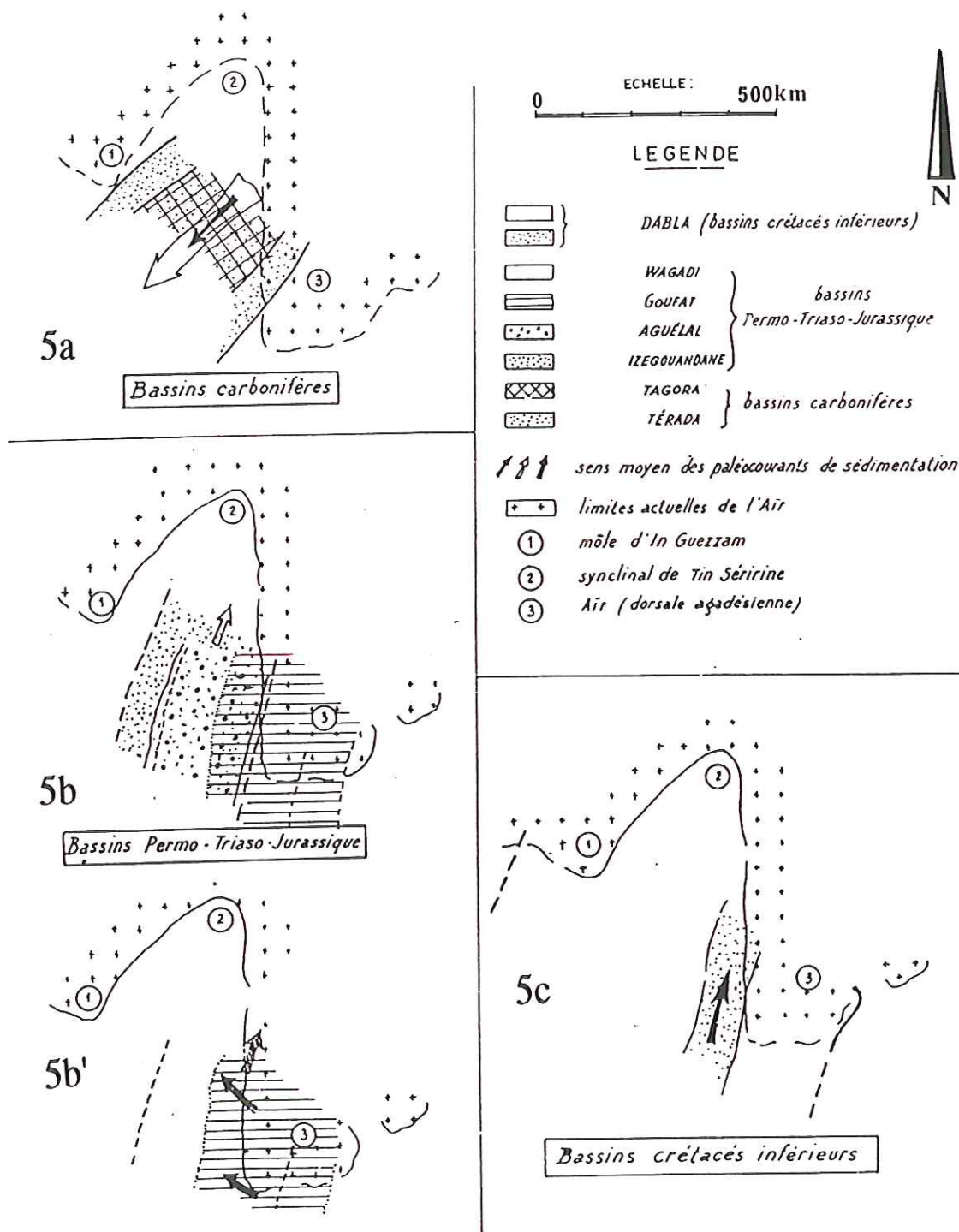
Fig. 5 - Schémas paléogéographique dans la région septentrionale du bassin des Iullemden (bassin de Tim Merso1) (d'après Valsardieu, 1970).
