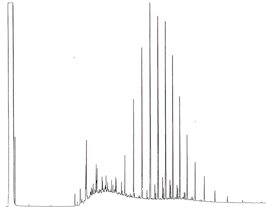
Fig.57 - Chromatogrammes d'hydrocarbures saturés représentant les principales distributions des n-alcane dans les échantillons de Taza et d'Akouta.
