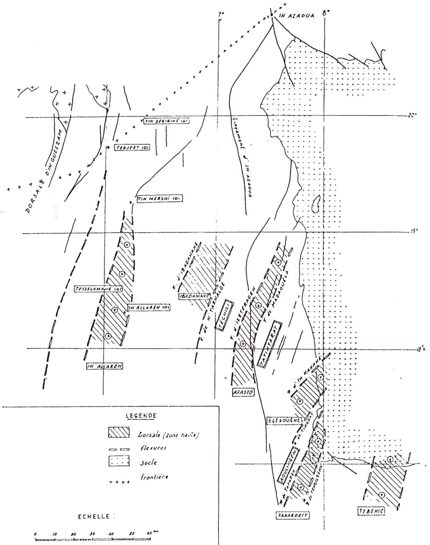
Fig. 16 - Les grandes cassures et les structures associées (d'après Valsardieu, 1970).
