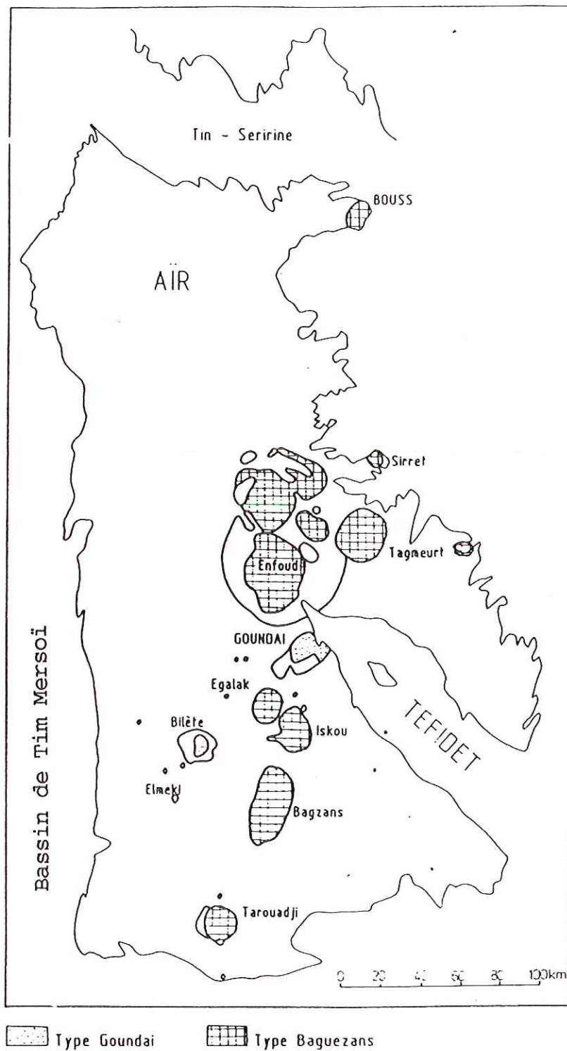
Fig.66 - Volcanisme paléozoïque dans l'Air (d'après Moreau, 1982; Ahmed, 1989).
