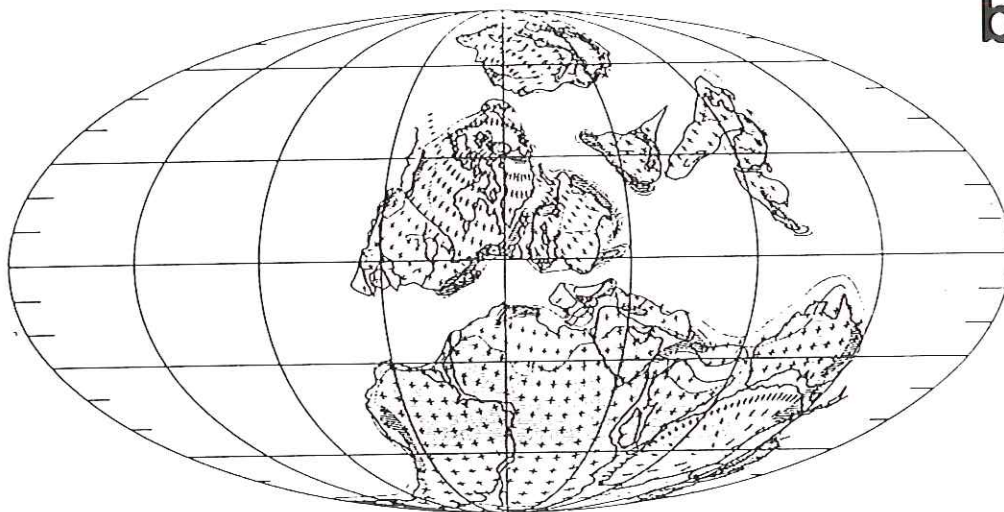
Fig.29- Position du continent africain au Paléozoïque (d'après Scotese et al., 1979).
