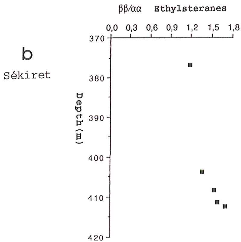
Fig. 37 - Ethyl cholestanes \beta\beta/\alpha (20R et 20S) en fonction de la profondeur.
