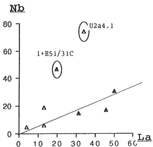
Fig.69 a - Correlation entre éléments incompatibles dans les faciès gréseux.
