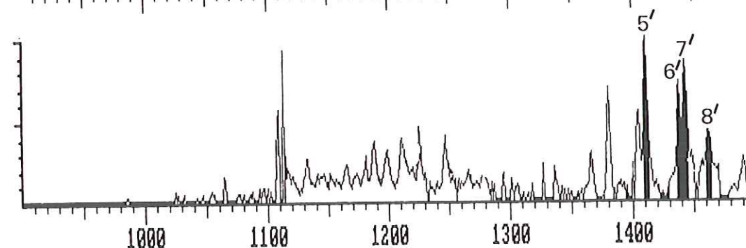
Fig.54 : Exemple de répartition des composés de la famille du dibenzothiofène à sékiret; comparaison avec celle du groupe des phénanthrènes.
