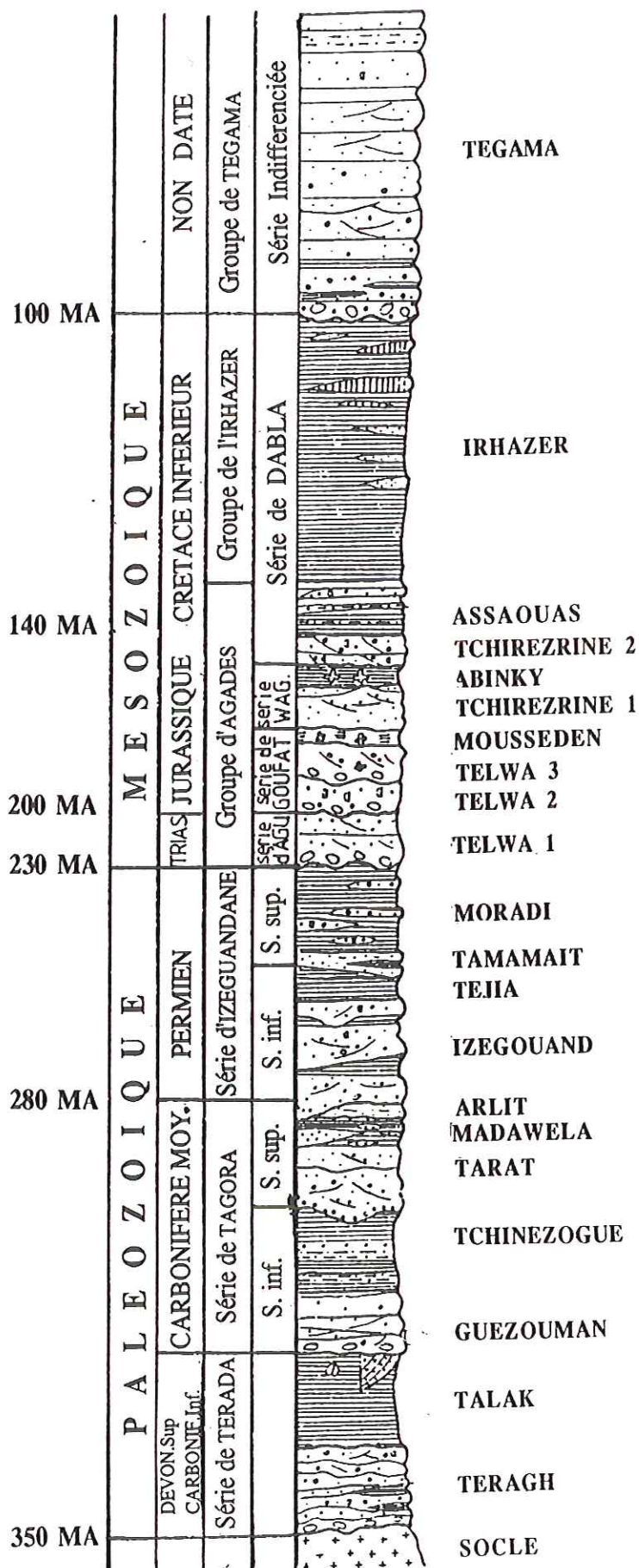
Fig. 3 - Coupe stratigraphique schématique du bassin de Tim Mersoi (empunté à Elhamet, 1983; d'après COGEMA).
