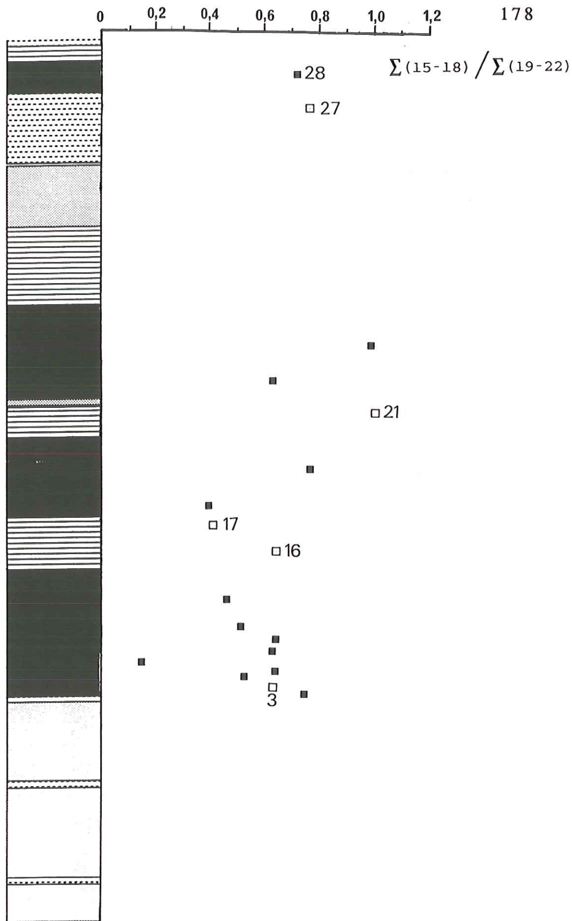
Fig.48 : Mise en évidence des variations d'intensité du phénomène de lessivage au sein de la série étudiée, à Sékiret, d'après l'altération des signatures en n-alcanes (explications dans le texte).
