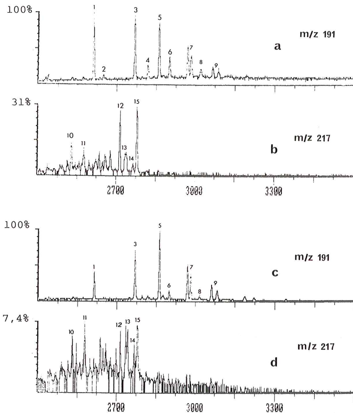
Fig.24- Proportion des stérans (b,d) par rapport aux hopanes (a,c) dans les échantillons d'Anou-Ararène (a et b) et de Sékiret (c et d).
