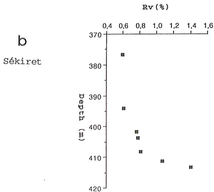
Fig. 38 - Réflectance de la vitrinite (%) en fonction de la profondeur.
