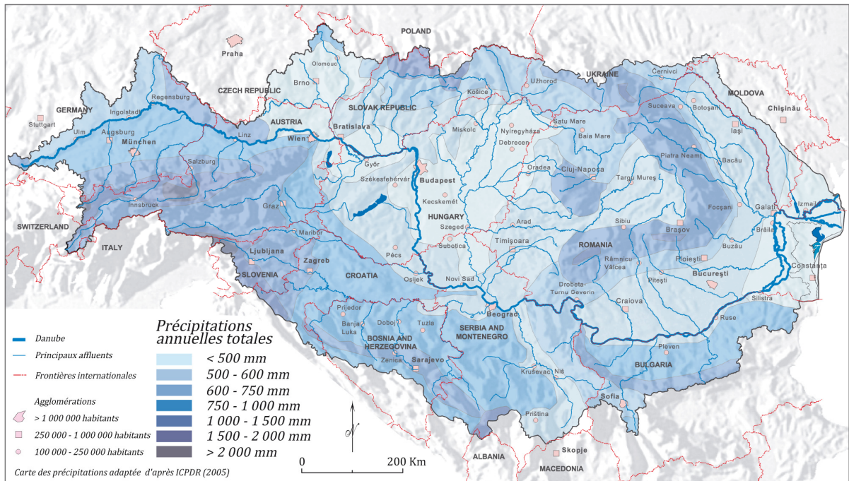
Figure 4 : Principaux éléments du relief du bassin versant du Danube (en haut) et distribution spatiale des précipitations cumulées sur l'année (en bas). Les altitudes sont issues de données SRTM (Shuttle Radar Topography Mission) et la carte des précipitations a été adaptée d'après ICPDR (2005).
