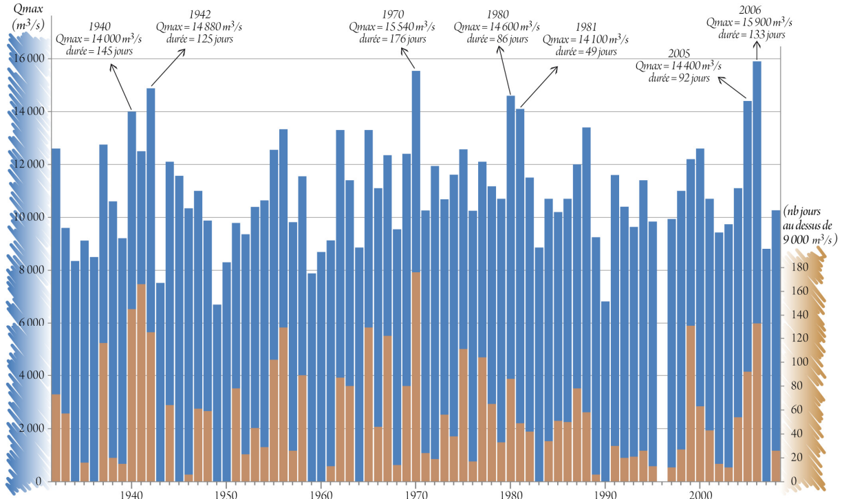
Figure 8 : Débits de pointe (moyenne journalière) des principales crues du Danube à Ceatal Izmail (1932 – 2008). La durée de la crue (colonnes en orange) correspond au nombre de jours consécutifs avec des débits supérieurs à 9 000 m 3 /s, celle-ci pouvant être associée à la durée d'inondation sur le delta du Danube.
