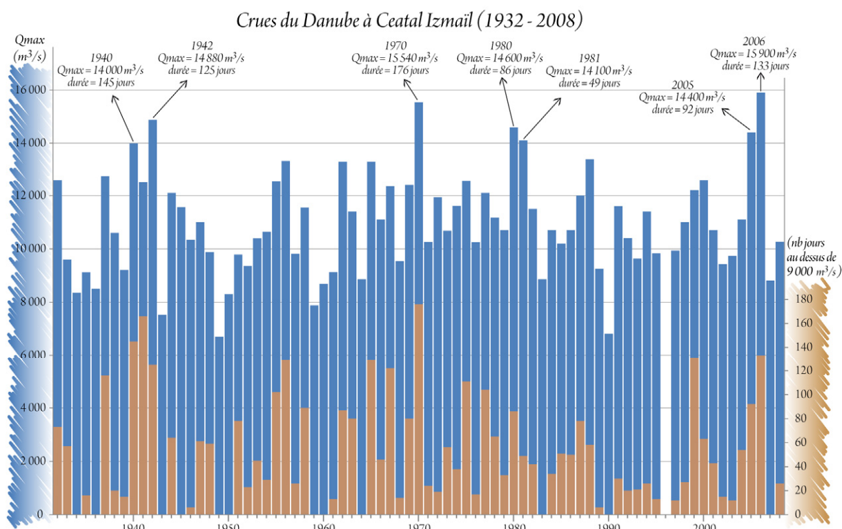
Figure 8 : Débits de pointe (moyenne journalière) des principales crués du Danube à Ceatal Izmail (1932 – 2008). La durée de la crue (colonnes en orange) correspond au nombre de jours consécutifs avec des débits supérieurs à 9 000 m 3 /s, celle-ci pouvant être associée à la durée d’inondation sur le delta du Danube.
