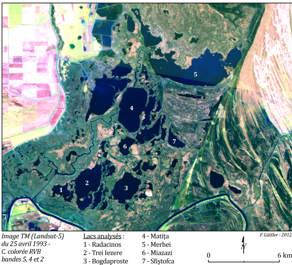
Figure 91 : Localisation des lacs analysés au sein de la sous-unité hydrologique de Matîța-Merhei.
