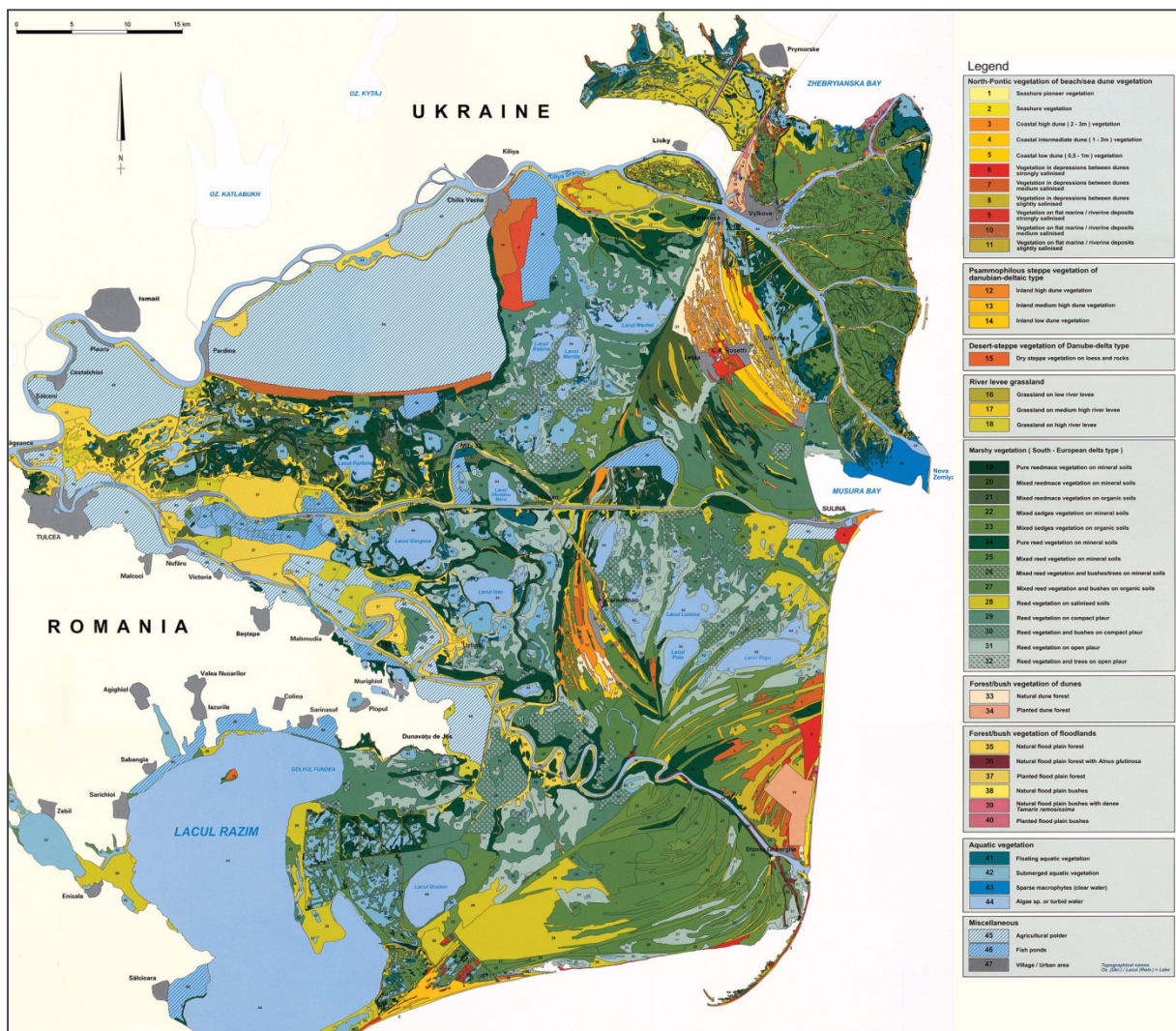
Figure 46 : Carte de la végétation du delta du Danube avec 44 types de végétation regroupés en 8 catégories (cf. légende à droite). Carte extraite de Hanganu et al. (2002).
