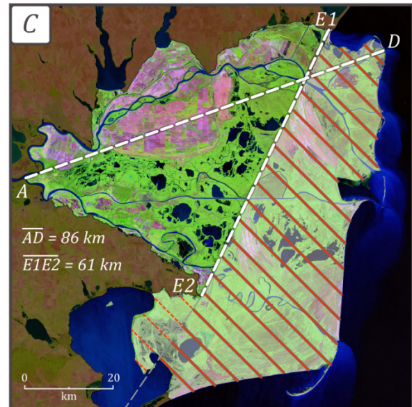
Figure 24 : A - Caractérisation générale du delta du Danube et délimitation de la plaine deltaïque. B - Limites du front deltaïque et du prodelta, lignes retracées d'après Panin (2003). C - Éléments de la géomorphométrie plane.
