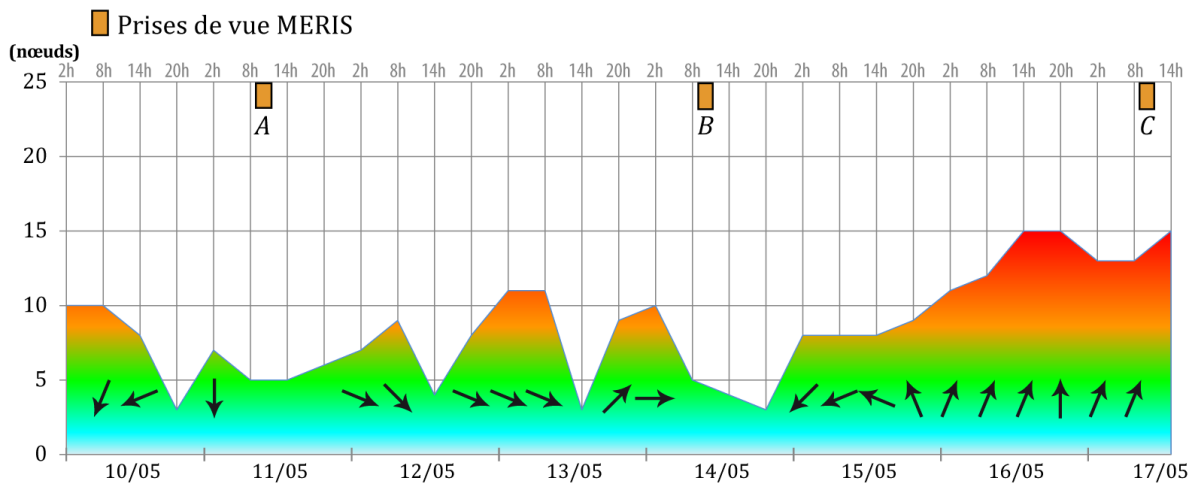
Figure 106 : L'effet du vent sur la forme et l'orientation des panaches sédimentaires au large du delta du Danube.
