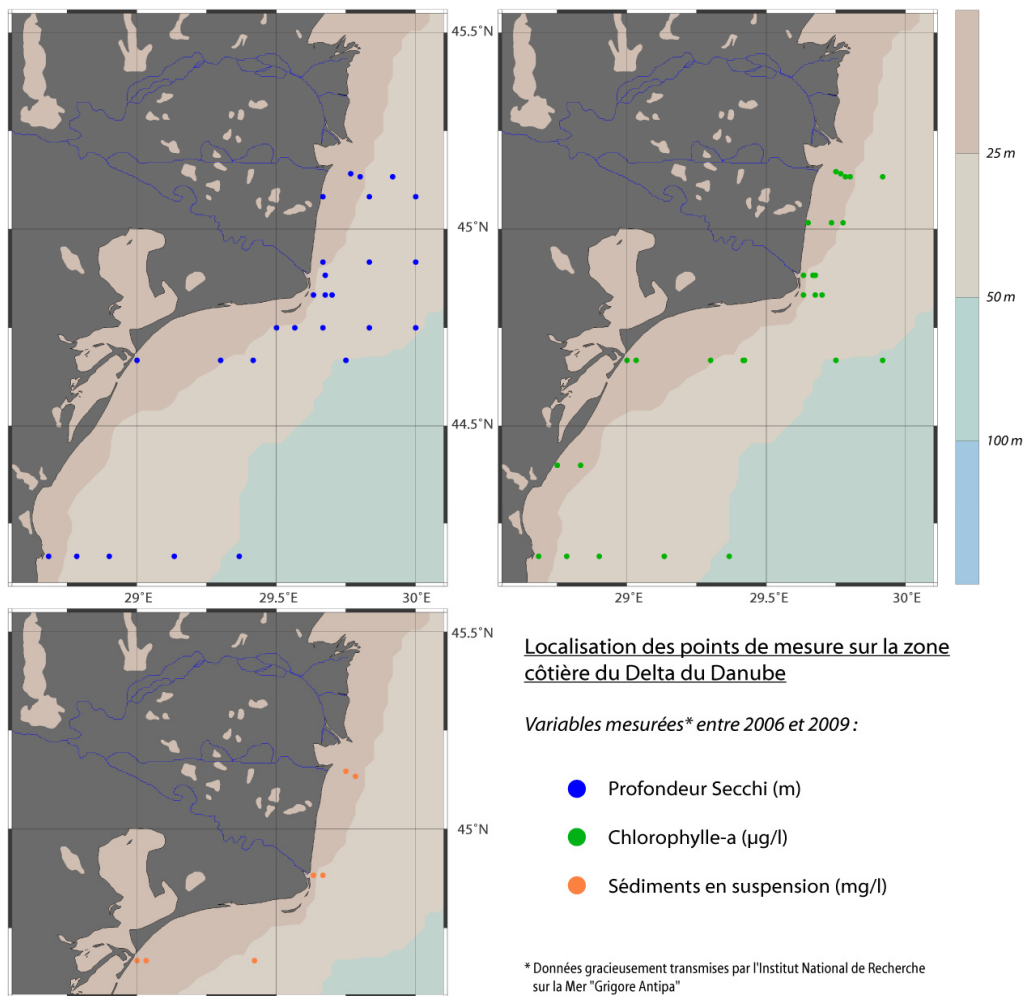
Figure 65 : Localisation des points de mesure in situ sur la zone côtière du delta du Danube selon les variables sélectionnées. La présence d'un point indique qu'au moins une mesure a été réalisée entre 2006 et 2009.
