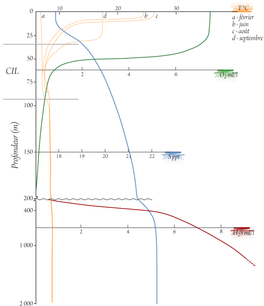
Figure 17 : Structure verticale approximative de la mer Noire en fonction de la température (T), de la salinité (S) et des concentrations en oxygène dissous (O 2 ) et en sulfure d'hydrogène (H 2 S). Graphique redessiné d'après Tolmazin (1985).
