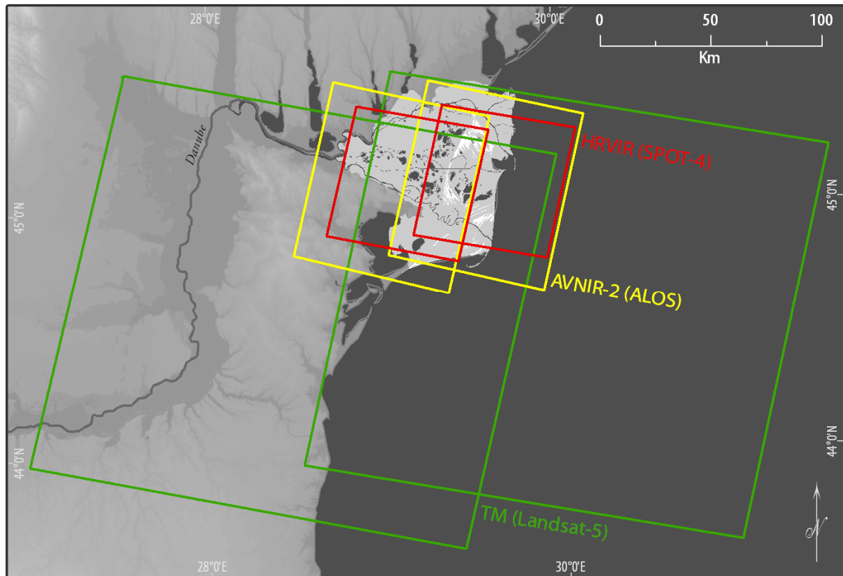
Figure 61 : Emprise au sol des scènes à haute résolution spatiale selon l'orbite du satellite sur la plaine du delta du Danube. Pour chacun des capteurs, il est possible de considérer deux orbites, une occidentale et une orientale (cette appellation s'applique également aux scènes respectives).
