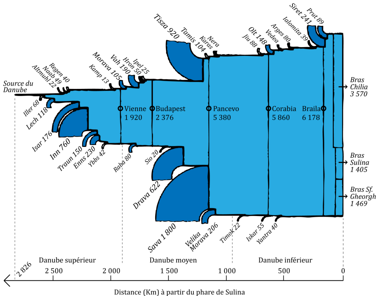
Figure 5 : Secteurs et réseau hydrographique du bassin du Danube. La contribution liquide (moyennes annuelles en m^3/s ) des principaux affluents est indiquée sur le schéma en-dessous de la carte. Les valeurs de débit sont issues de Sommerwerk et al. (2009), sauf pour les trois bras à l'embouchure du fleuve (calculés par ailleurs). La conception du schéma inférieur a été inspirée par l'illustration originale (orientée verticalement) de Liepolt (1967), reprise par Sommerwerk et al. (2009).
