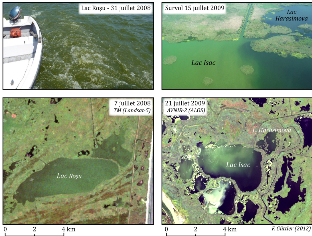
Figure 110 : Exemples de blooms de phytoplancton observés sur le terrain en juillet 2008 et juillet 2009 (en haut). Les images satellitaires (en bas) sont présentées en "vraies couleurs". Clichés : F. Güttler
