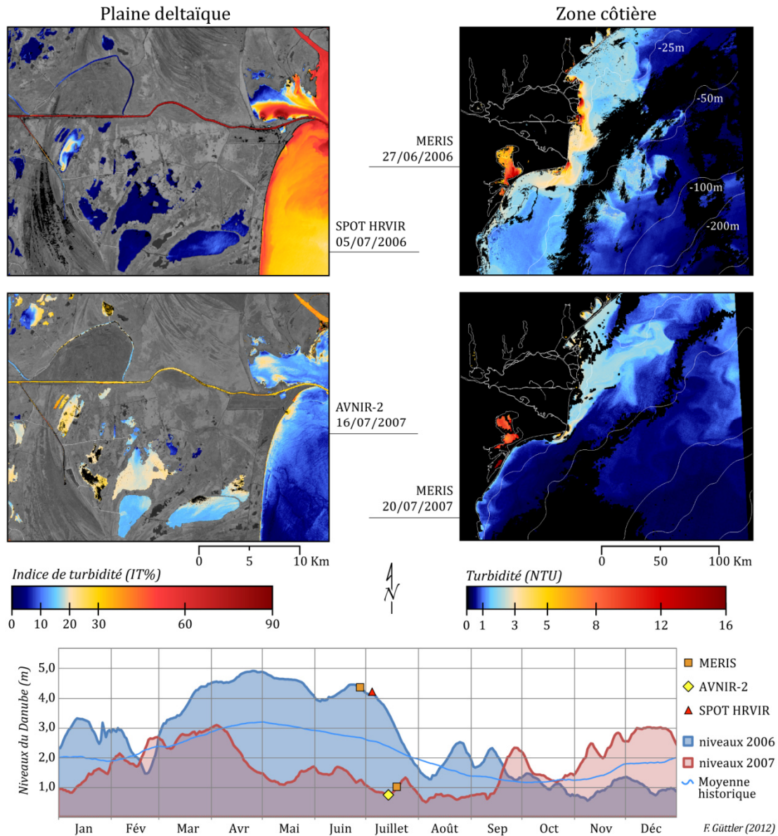
Figure 108 : Evolutions opposées de la turbidité entre la plaine deltaïque et la zone côtière. Les images en haut de la figure illustrent la situation lors de l'été 2006, tandis que celles du milieu se réfèrent à l'été 2007. Le graphique permet de comparer les niveaux du Danube entre les deux années et au moment des prises de vue.
