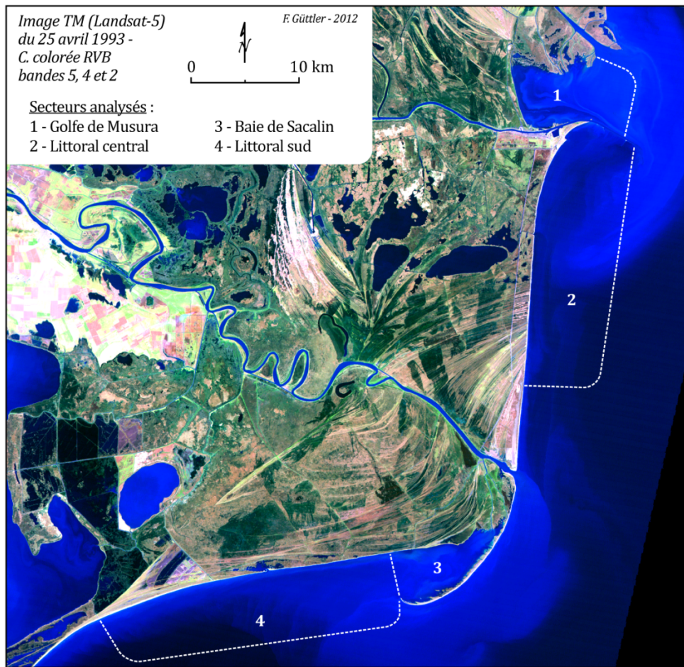
Figure 95 : Secteurs sélectionnés au sein de la zone côtière.
