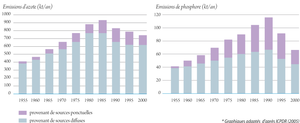
Figure 15 : Évolution des émissions de nutriments sur le bassin du Danube selon le modèle MONERIS (DaNUbs). Adapté d'après (ICPDR, 2005).
