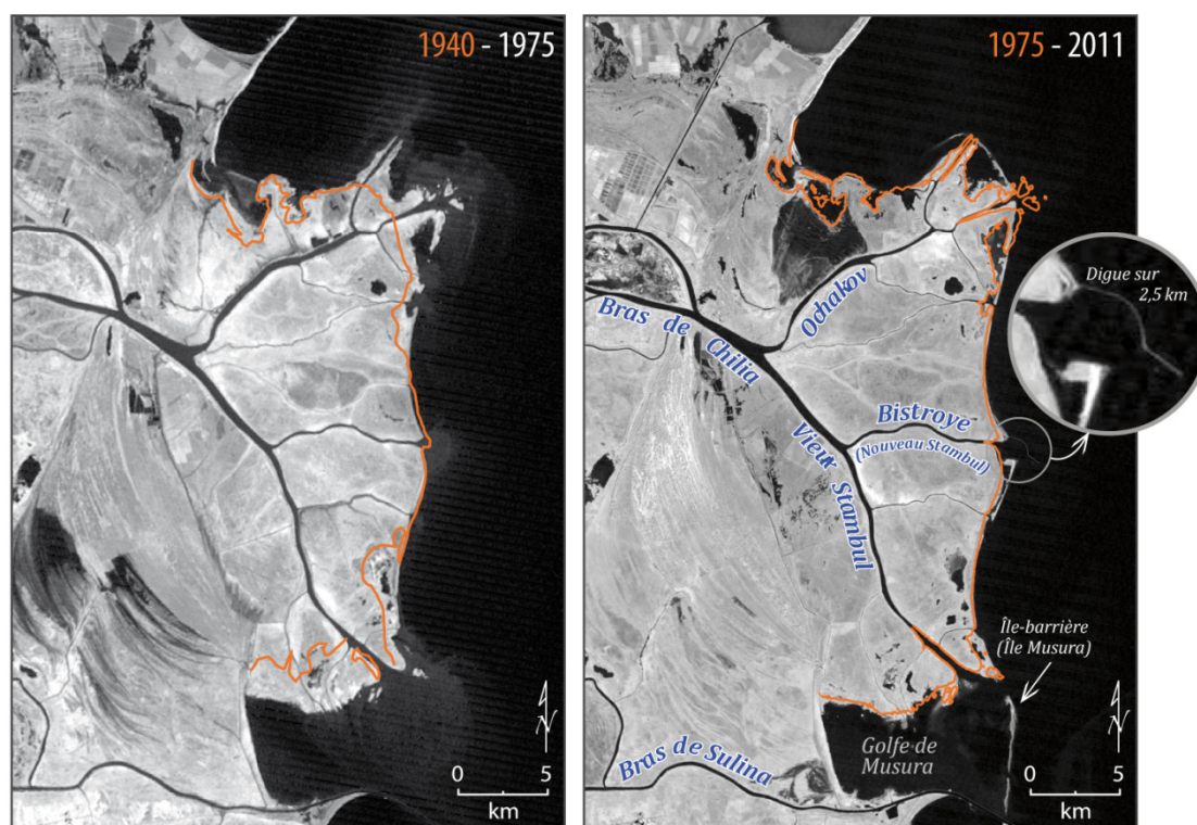
Figure 28 : Restitution graphique du trait de côte sur le secteur de l'embouchure du bras de Chilia. Les contours entre 1856 et 1940 sont issus de Giosan et al. (2005) – les zones en gris correspondent à la progradation observée entre deux dates, tandis que celles en noir indiquent un retrait. Le trait de côte de 1975 a été extrait à partir du traitement numérique de l'image MSS (Landsat-2), à gauche, alors que celle de 1975 a été acquise par le capteur TM (Landsat-5) en octobre 2011.
