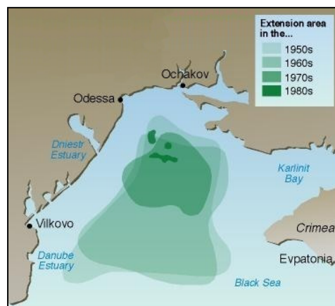
Figure 21 : Réduction du champ de Phyllophora (Champ de Zernov) durant la deuxième moitié du XX e siècle. Source : Zaitsev et Mamaev (1997) - graphisme par P. Rekeawicz (UNEP/GRID-Arendal, 2006).
