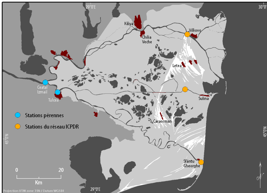
Figure 64 : Localisation des stations hydrologiques sur la plaine du delta du Danube.
