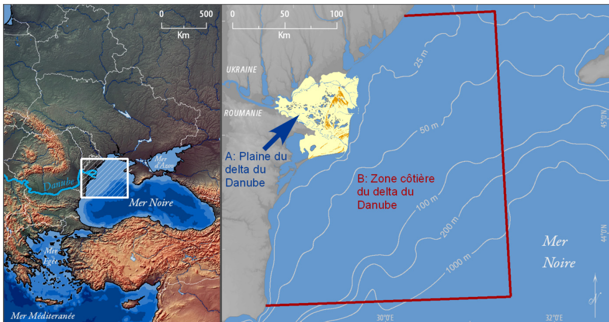
Figure 55 : Localisation des deux sous-zones d'étude (A et B) dans le contexte de la portion nord-ouest de la mer Noire.
