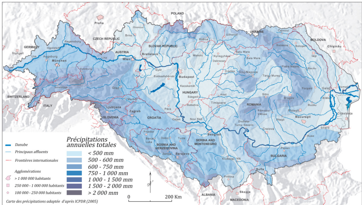
Figure 4 : Principaux éléments du relief du bassin versant du Danube (en haut) et distribution spatiale des précipitations cumulées sur l'année (en bas). Les altitudes sont issues de données SRTM ( Shuttle Radar Topography Mission ) et la carte des précipitations a été adaptée d'après ICPDR (2005).
