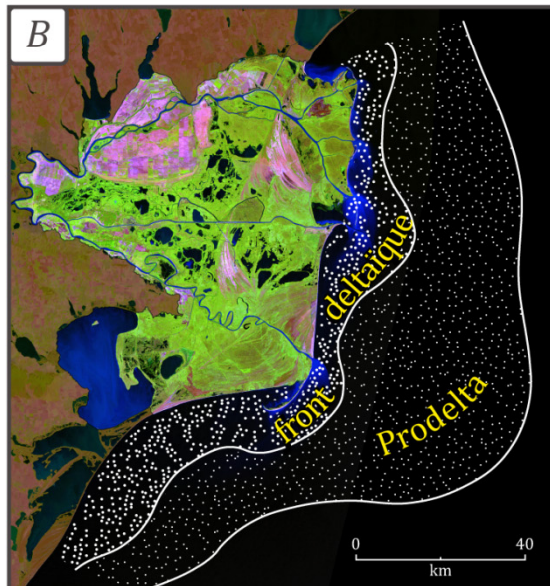
Figure 24 : A - Caractérisation générale du delta du Danube et délimitation de la plaine deltaïque. B - Limites du front deltaïque et du prodelta, lignes retracées d'après Panin (2003). C - Éléments de la géomorphométrie plane.
