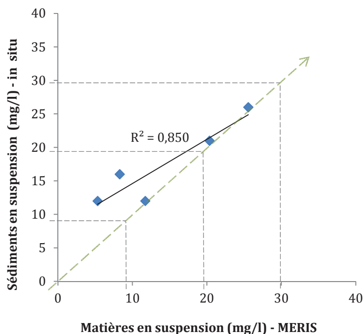
Figure 79 : Sédiments en suspension (in situ) versus matières en suspension (satellite) à l'embouchure du bras de Sf. Gheorghe. Données satellitaires à moyenne résolution spatiale issues du capteur MERIS.
