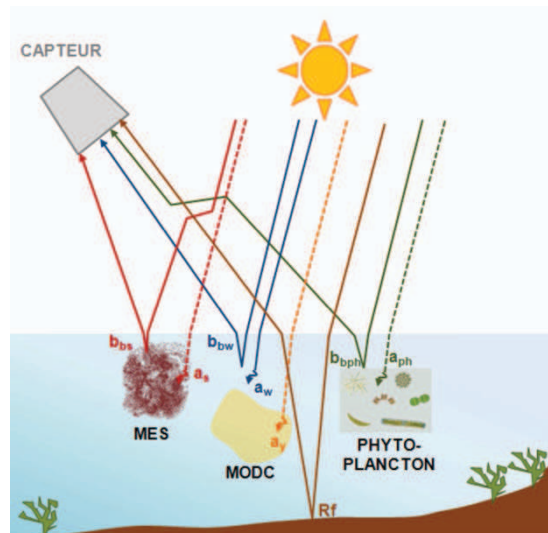
Figure 54 : Composants influençant la lumière émergeant de la surface de l'eau. Source : Petus (2009)
