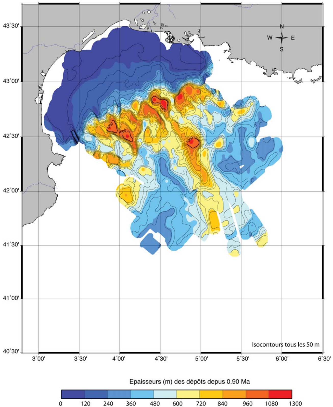
FIGURE 10.21 – Epaisseurs (m) des dépôts depuis 0.90 Ma.
