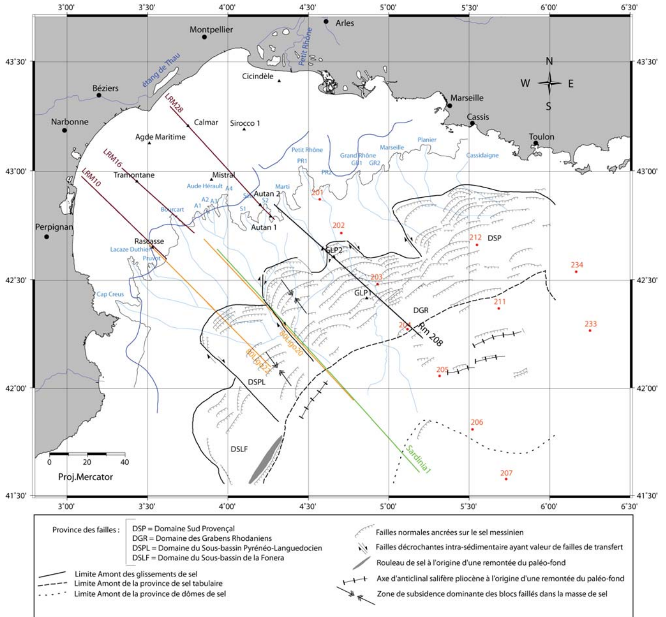
FIGURE 5.19 – Plan de position des profils de la fig. 5.20 perpendiculaires à la marge. Les éléments de tectonique salifère de [DosReis, 2001] sont indiqués. La limite entre la surface d'érosion messinienne rugueuse et la surface d'abrasion lisse de [Bache, 2008] est tracée en bleu foncé. Le rebord de plateau et les talwegs des canyons actuels sont repérés en bleu clair.
