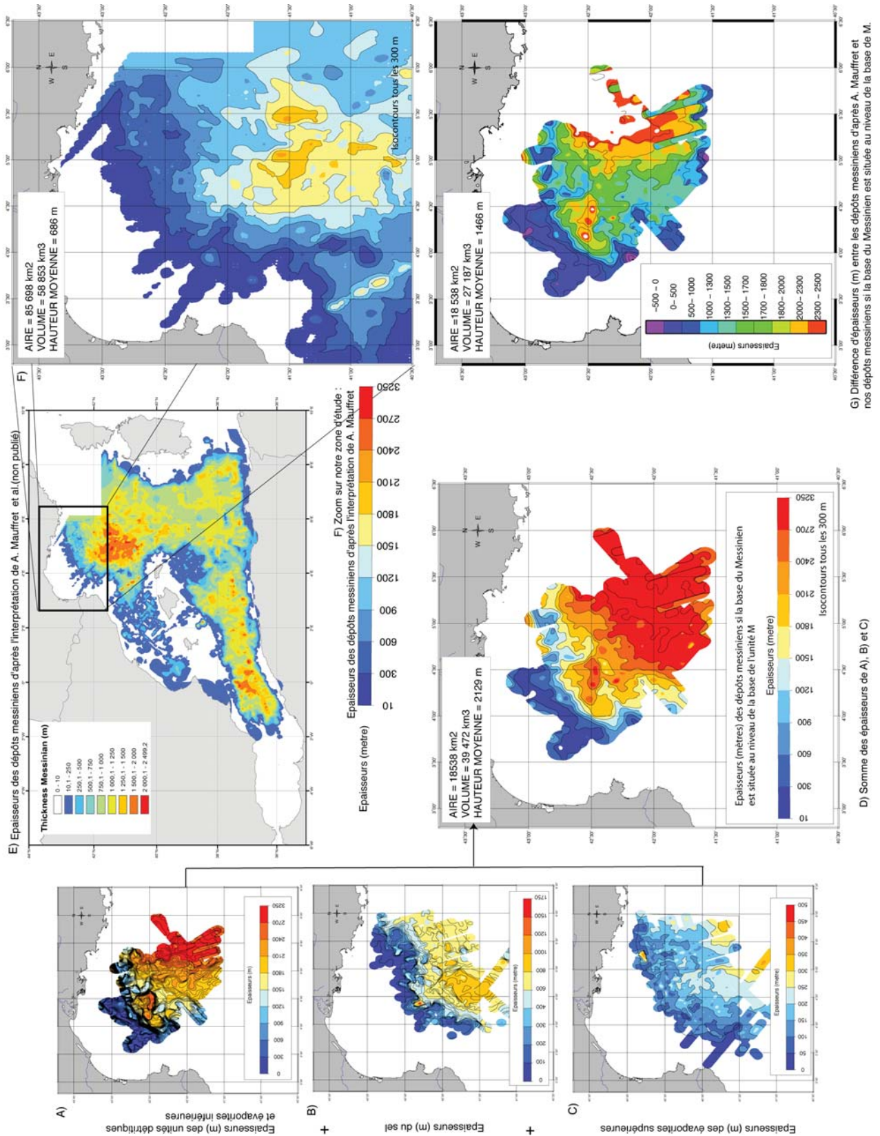
FIGURE 6.21 – Comparaison de nos cartes d'épaisseurs et volumes Messiniens avec les données de A. Mauffret (non publiées). A) Isoques (m) des séries détritiques (unités M0, M1, Ma) et évaporites inférieures (Mb) ; B) Isoques (m) du sel ; C) Isoques des évaporites supérieures ; D) Epaisseurs (m) des dépôts messiniens (épaisseurs cumulées de A, B et C) ; E) Epaisseurs (m) des dépôts messiniens d'après l'interprétation d'A. Mauffret ; F) Epaisseurs (m) des dépôts messiniens d'après l'interprétation d'A. Mauffret extraites sur notre zone d'étude ; G) Différence d'épaisseurs (m) entre nos dépôts messiniens (si la base de l'unité M correspond à la base de la crise) et les dépôts messiniens d'après A. Mauffret. NB : la même échelle de couleurs est adoptée pour les cartes D) et F).
