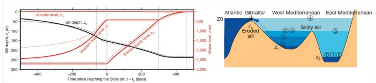
FIGURE 3.10 – Scénario de réennoisement des bassins de Méditerranée. Courbes du niveau marin en Méditerranée et de la profondeur du seuil de Sicile (Gauche). Illustration schématisque du remplissage (Droite) avec (0) niveau marin avant réennoisement, (1) période d'incision maximale du seuil, (2) le niveau marin de la Méditerranée occidentale atteint le seuil de Sicile, (3) le niveau marin de la Méditerranée orientale atteint le seuil de Sicile, (4) l'ensemble de la Méditerranée est rempli. [Garcia-Castellanos et al., 2009].
