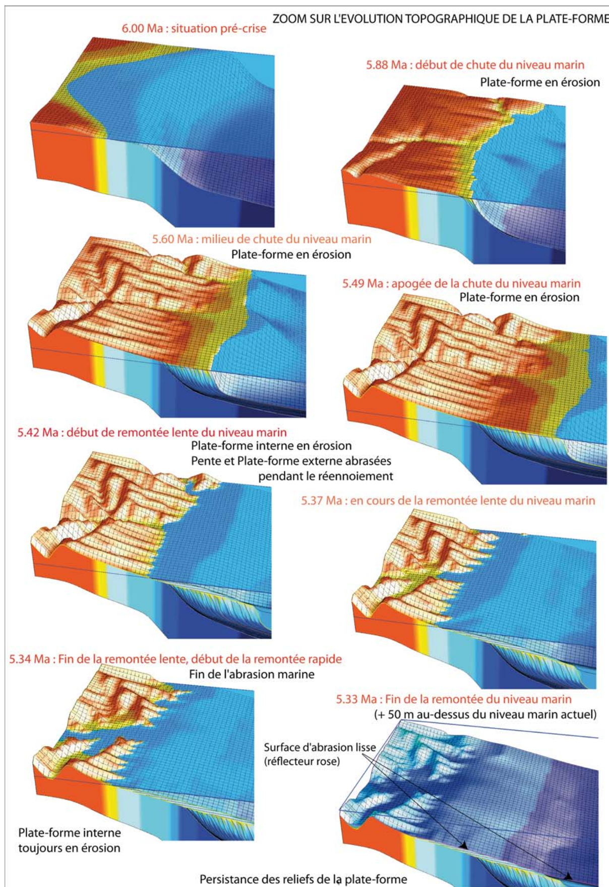
FIGURE 7.26 – Ravinement de la pente et de la plate-forme externe lors de la phase de remontée lente du niveau marin. La remontée rapide du niveau marin conserve la rugosité du paysage sur la plate-forme interne. Le réflecteur rose correspond à la fin de la transgression à 5.33 Ma.
