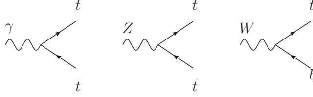
FIGURE 1.9: Vertex faisant intervenir un quark top et un boson de l'interaction faible.
