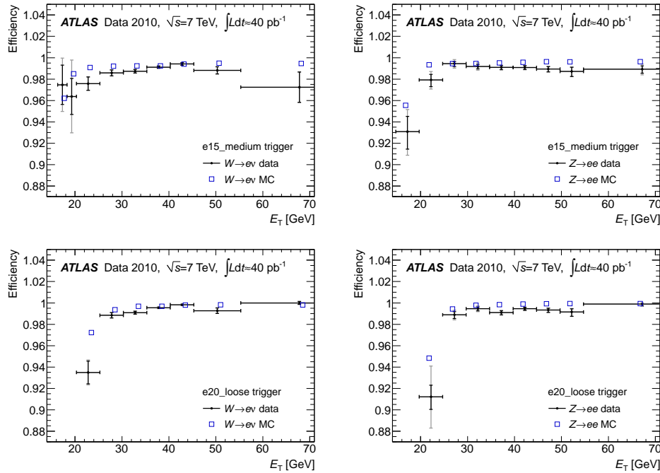
FIGURE 3.6: Comparaison des efficacités de trigger des électrons dans la simulation (carrés bleus) et dans les données (croix noires). En haut : efficacité du déclenchement e_{15\_medium} en fonction de E_T en utilisant des événements W \rightarrow e\nu (à gauche) et Z \rightarrow ee (à droite). En bas : efficacité du déclenchement e_{20\_loose} en fonction de E_T en utilisant des événements W \rightarrow e\nu (à gauche) et Z \rightarrow ee (à droite).
