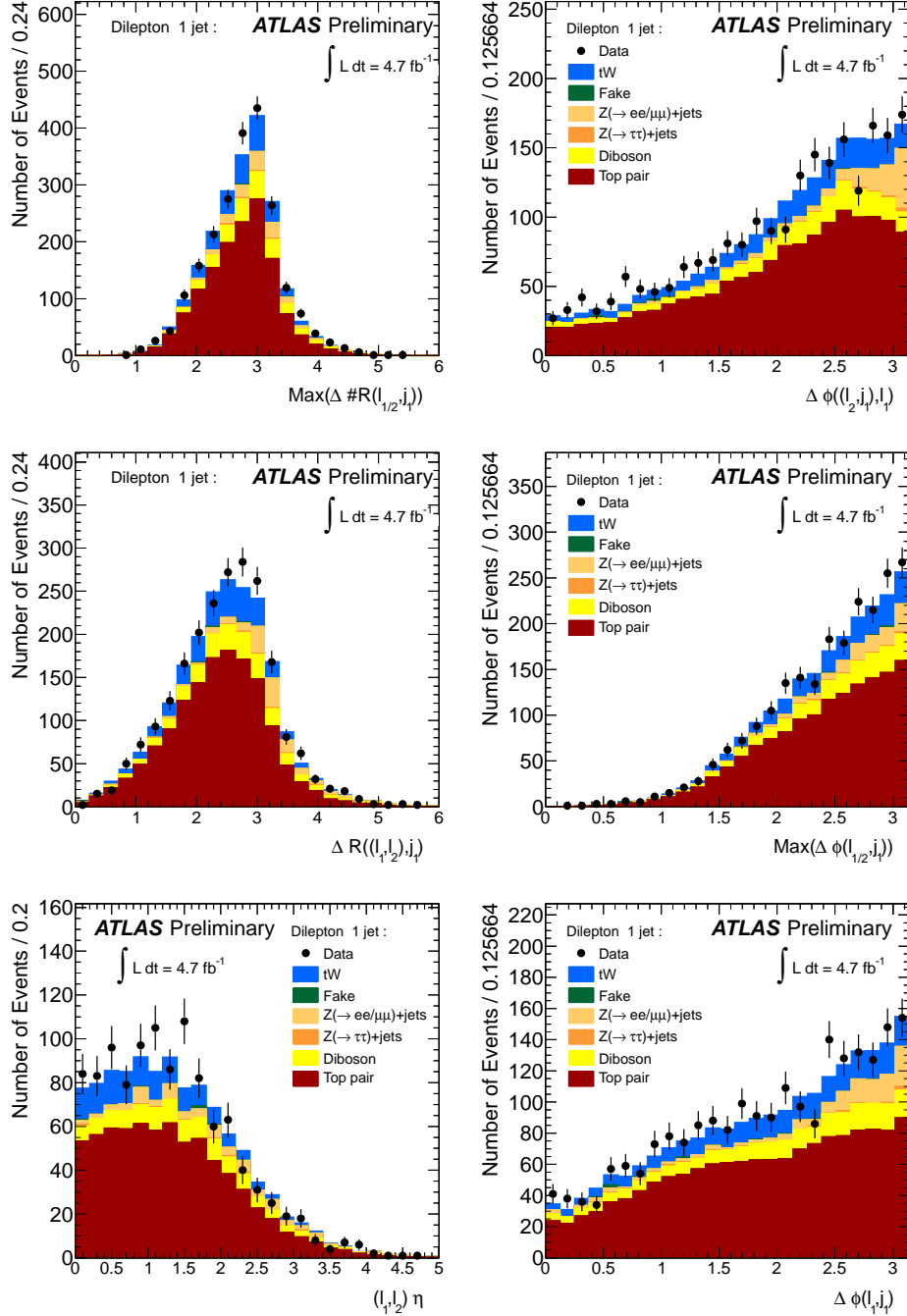
FIGURE B.2: Distribution de \Delta R[(l_1, l_2), j_1] , \text{Max} \Delta \phi(l, j) , \eta(l_1, l_2) , \Delta \phi(l_1, j_1) dans les événements à 1 jet
