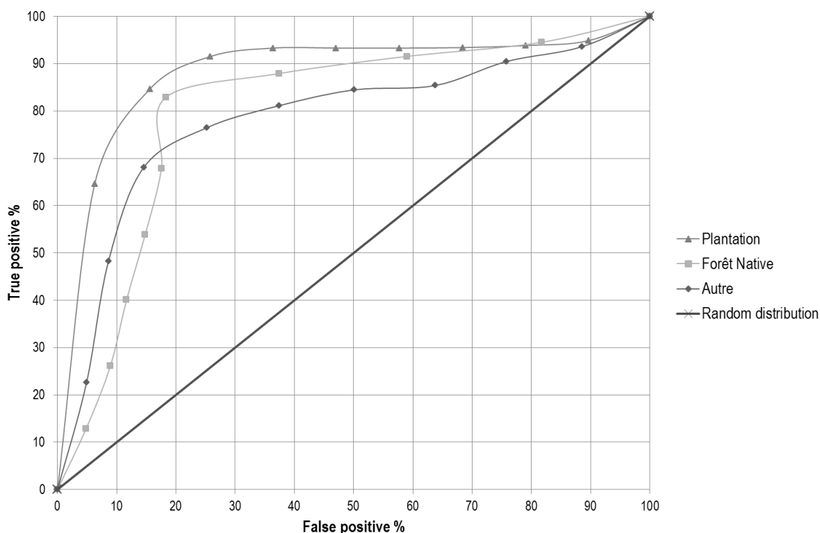
Figure 114 : ROC pour le modèle LCM
