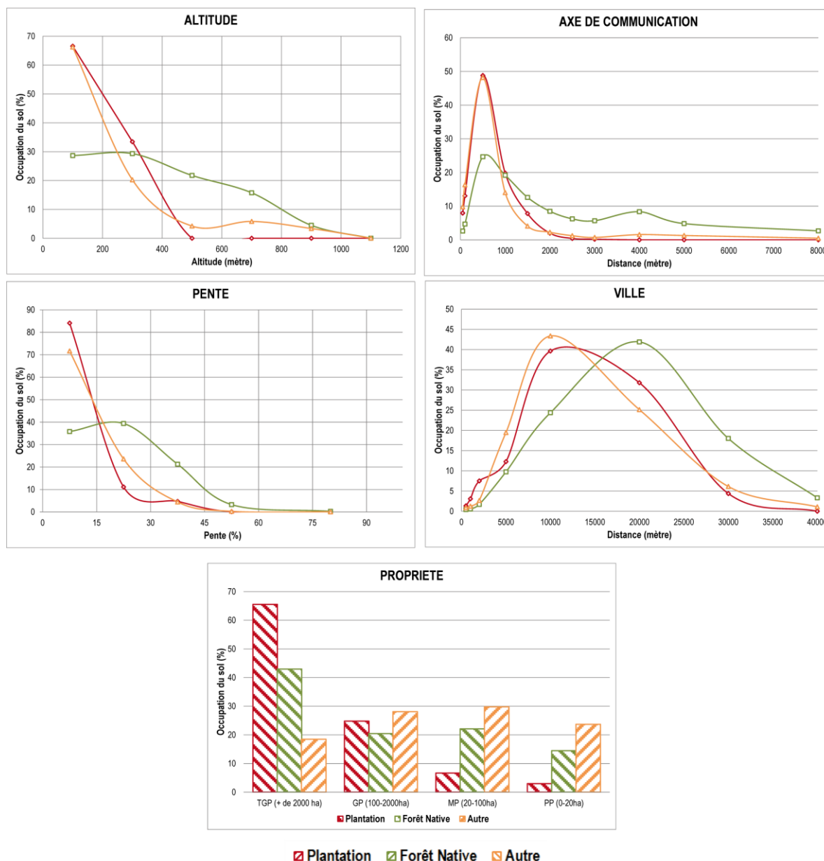
Figure 88 : Relation entre les types d’occupation du sol (1999) et cinq variables explicatives
