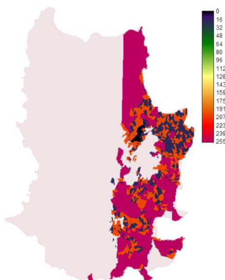
Figure 94 : Standardisation du facteur PROTER
