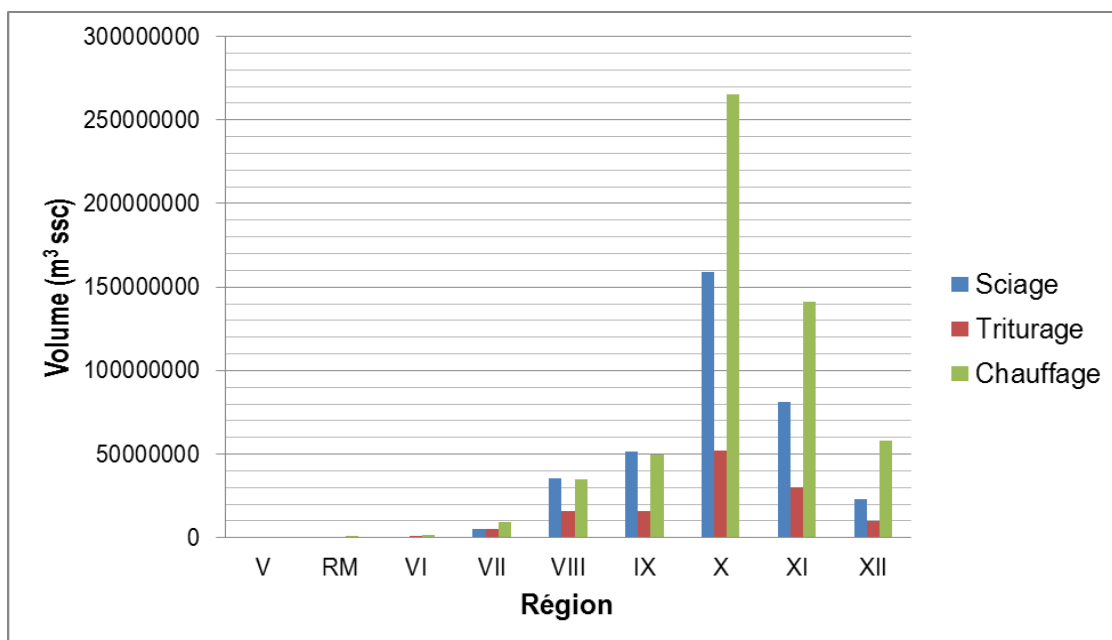
Figure 7 : Volume total (m 3 ssc) de bois natif par Région. Source : CONAF-CONAMA-BIRF, décembre 1999
