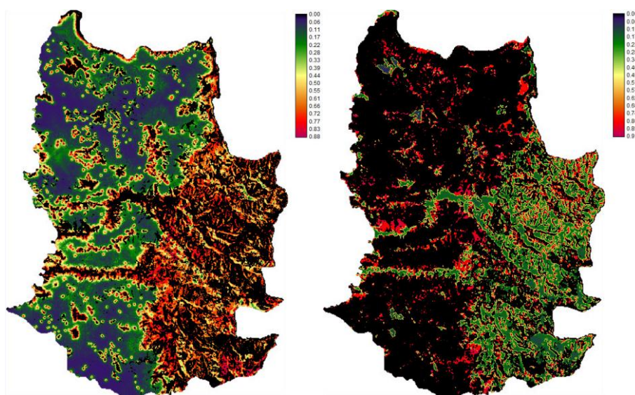
Figure 103 : Cartes de transition potentielle - DEFORESTATION (à gauche) et COLONISATION NATURELLE (à droite)
