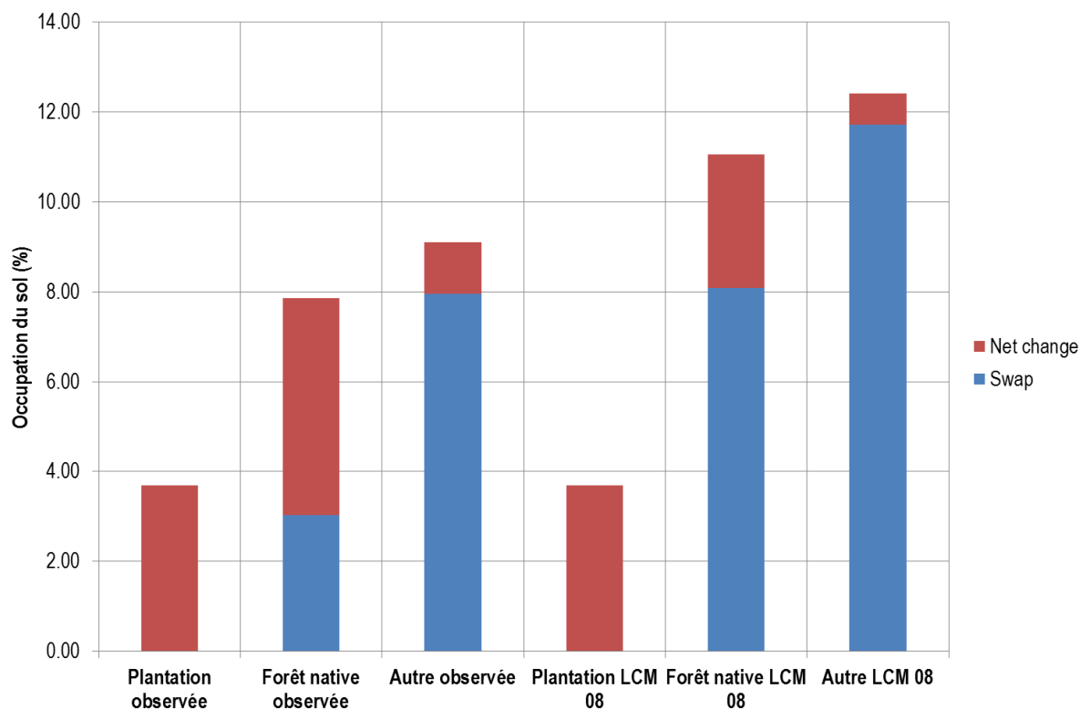
Figure 112 : Comparaison entre le LUC-budget réel (1999-2008) et le LUC-budget simulé (1999 réel – 2008 LCM). La barre totale (net change + swap) représente le % total de changement
