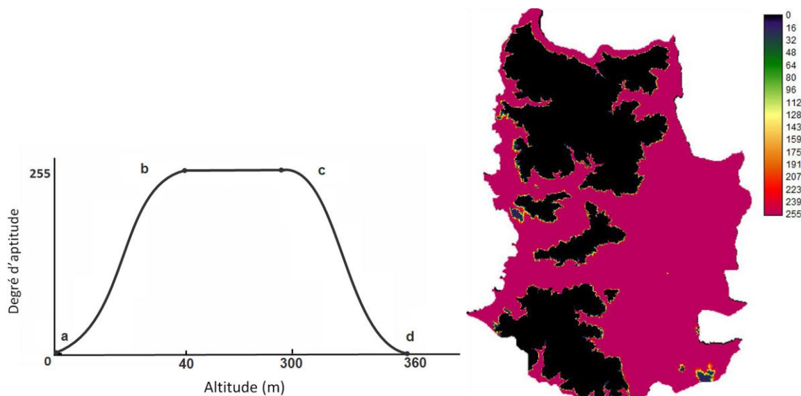
Figure 98 : Standardisation du facteur ALT
