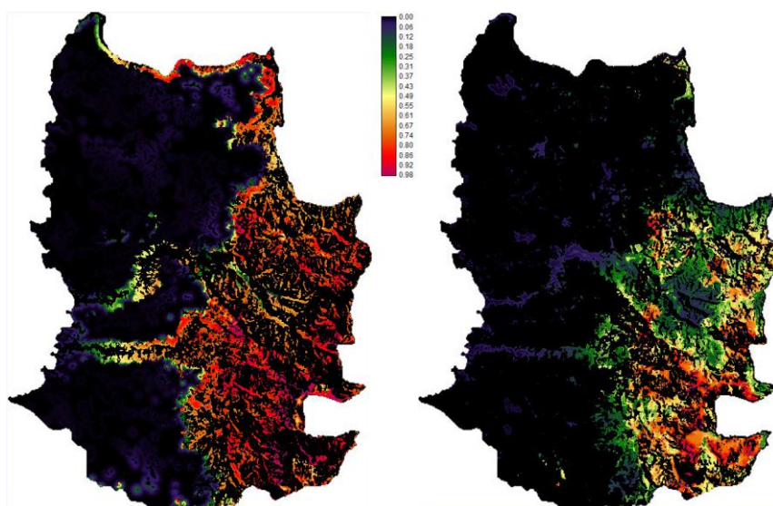
Figure 104 : Cartes de transition potentielle - PLANTATION
