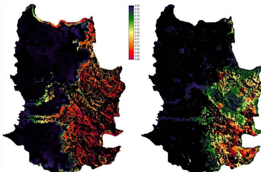
Figure 104 : Cartes de transition potentielle - PLANTATION
