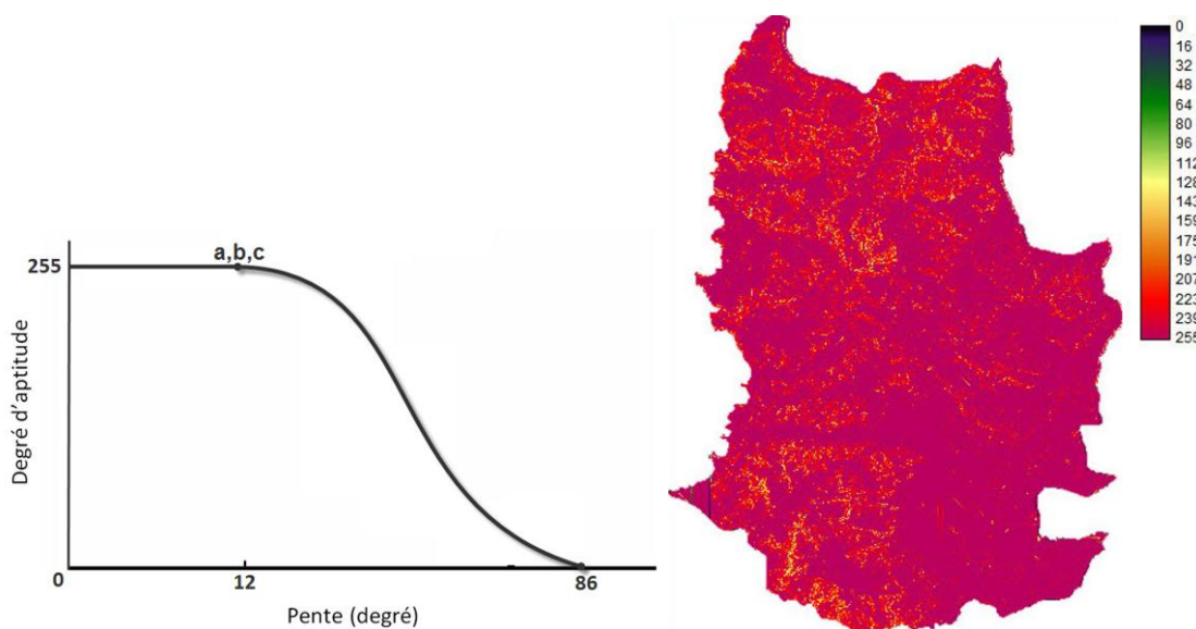
Figure 99 : Standardisation du facteur PTE
