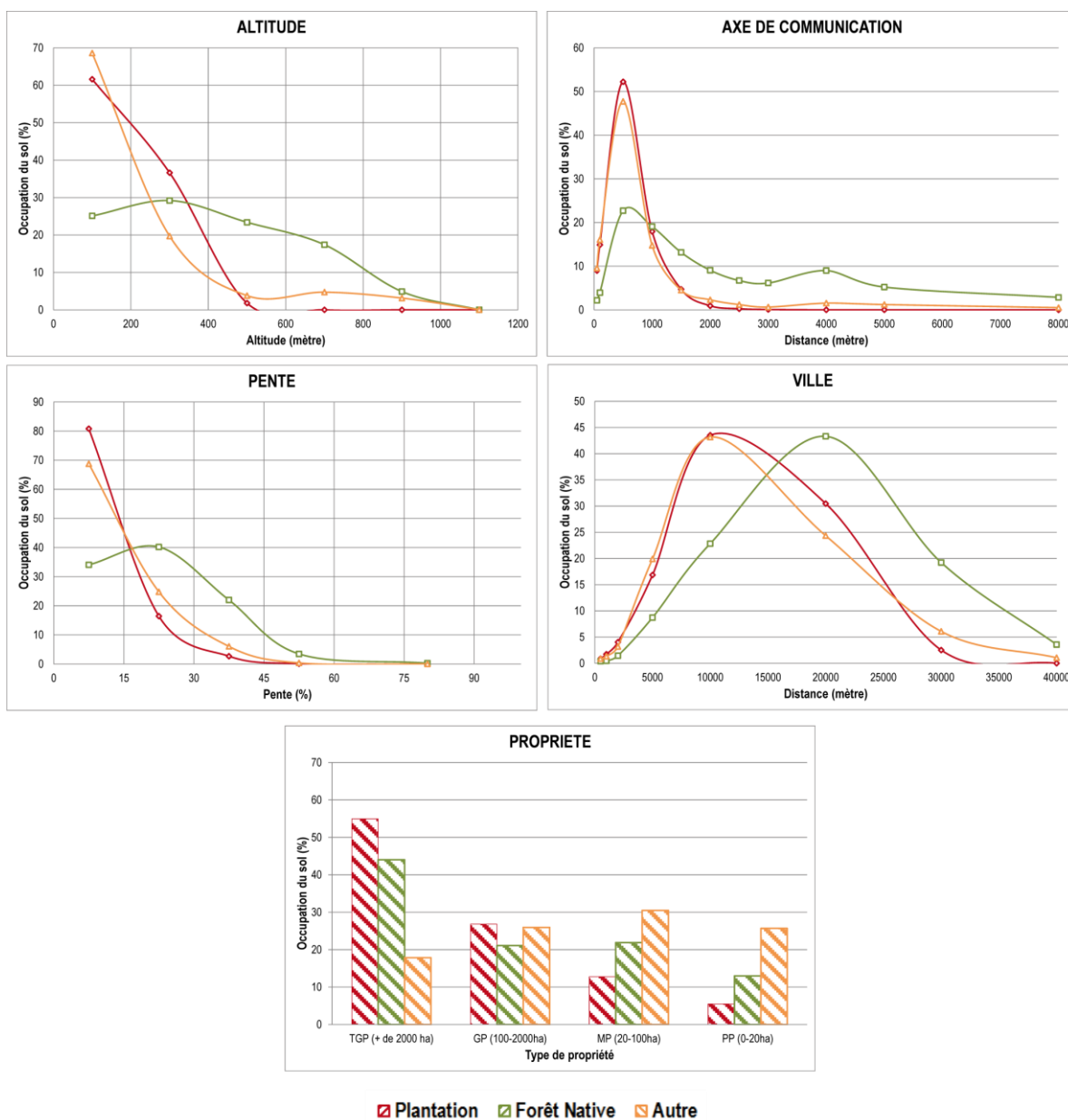
Figure 89 : Relation entre les types d'occupation du sol (2008) et cinq variables explicatives
