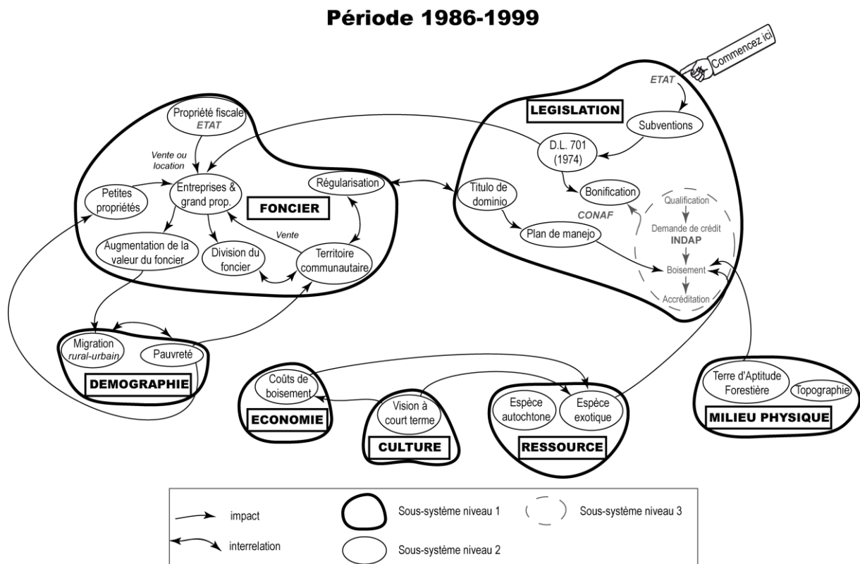
Figure 83 : Représentation systémique pour la période 1986-1999
