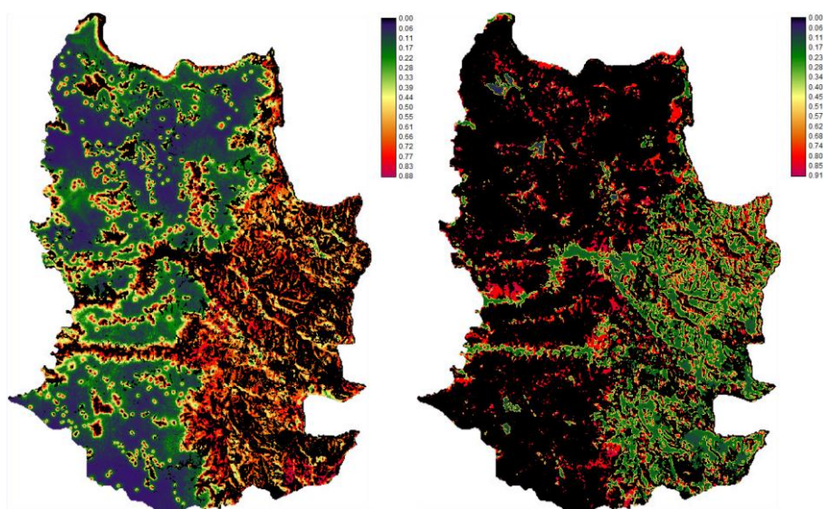
Figure 103 : Cartes de transition potentielle - DEFORESTATION (à gauche) et COLONISATION NATURELLE (à droite)
