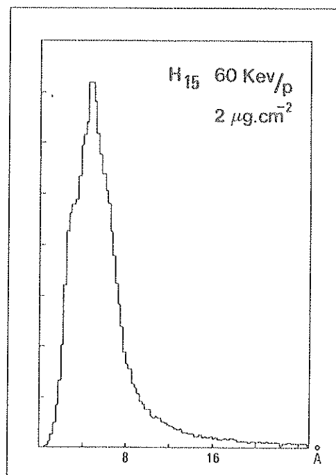
Figure 2.25 : Distributions des distances interprotoniques en sortie de cible de 2\mu\text{g}\cdot\text{cm}^{-2} pour des agrégats \text{H}_5^+ , \text{H}_7^+ , \text{H}_9^+ , \text{H}_{15}^+ incidents de 60 keV/p.
