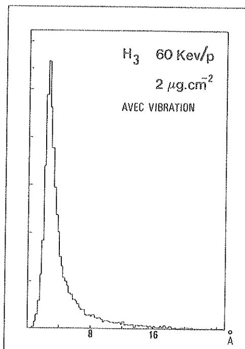
Figure 2.24 : Distributions des distances interprotoniques en sortie d'une cible de 2\mu\text{g}\cdot\text{cm}^{-2} pour des ions \text{H}_2^+ et \text{H}_3^+ incidents de 60 keV/p. En haut sans tenir compte de la répartition des ions incidents dans des états vibrationnels élevés. En bas en prenant en compte cet effet.
