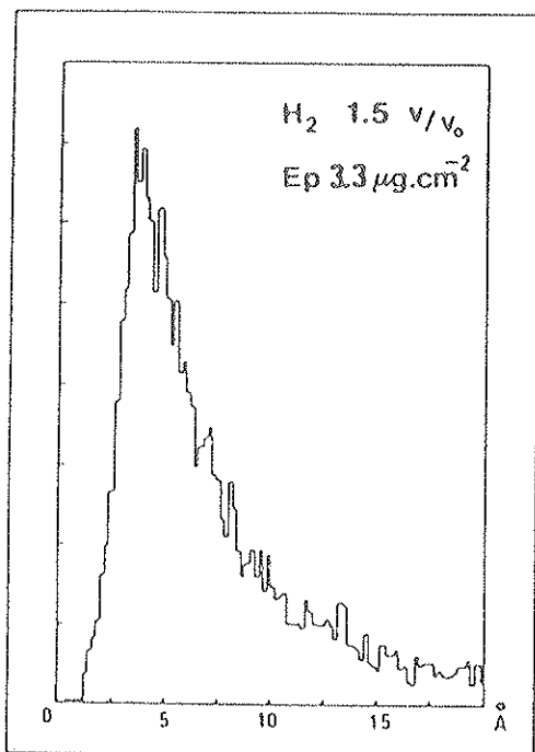
Distance interprotonique
