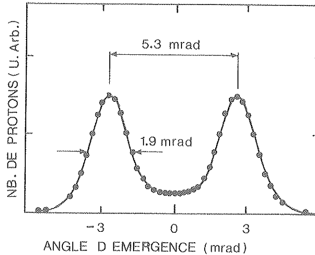
Figure C1 : Distribution angulaire des protons à l'émergence mesurée par D. GEMMEL avec des faisceaux d'ions H_2^+ d'énergie 1.4 MeV/p dans une cible de 1.6\mu g.cm^{-2} .
