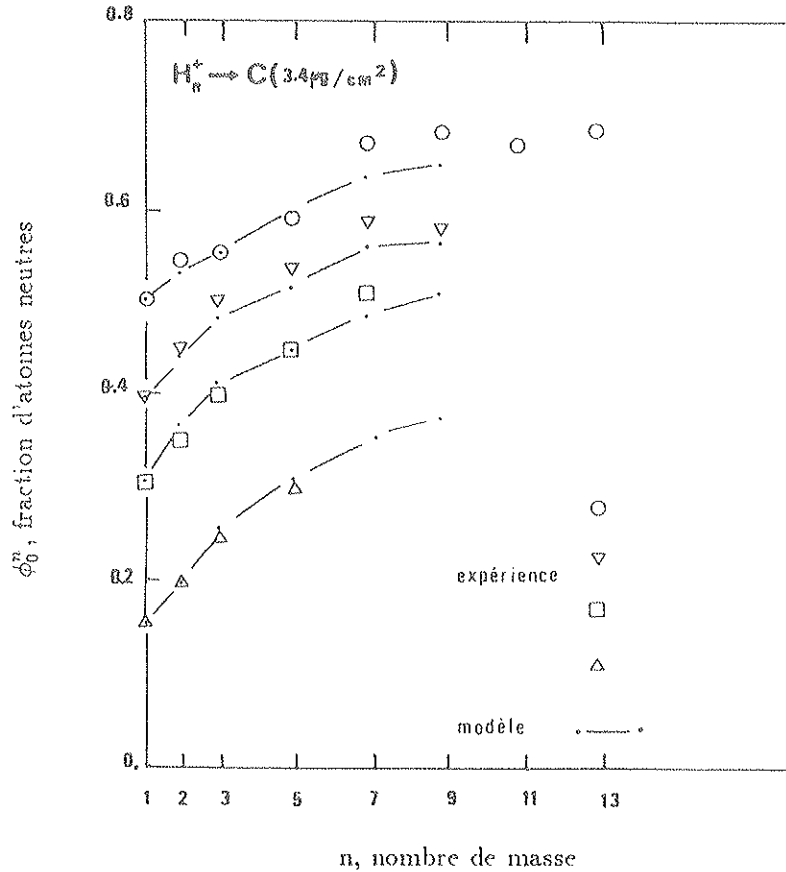
Figure 3.18 : Comparaison des fractions d'atomes neutres calculées avec celles mesurées par B. MAZUY et al. [15].
