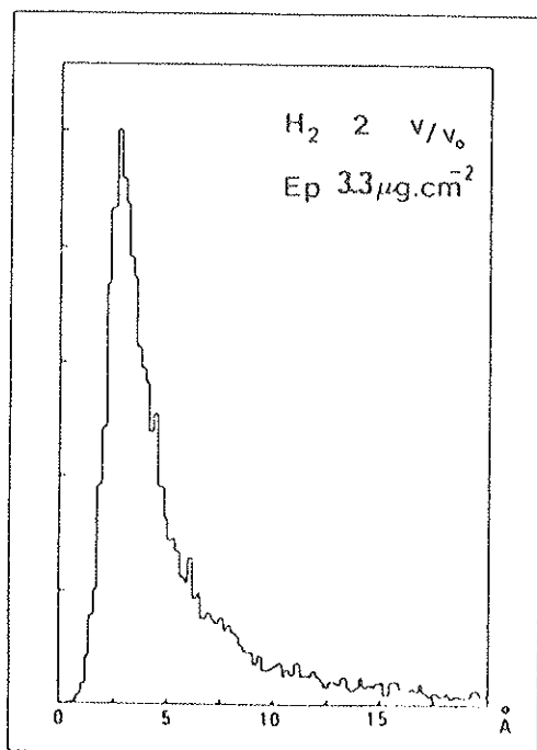
Figure 2.27 : Distributions des distances interprotoniques à la sortie de cibles de 3.3 \mu g \cdot cm^{-2} et de 6 \mu g \cdot cm^{-2} pour des ions H_2^+ incidents de vitesse de 1.5v_0 ( 40 \text{ keV/p} ) à 6v_0 ( 990 \text{ keV/p} ).
