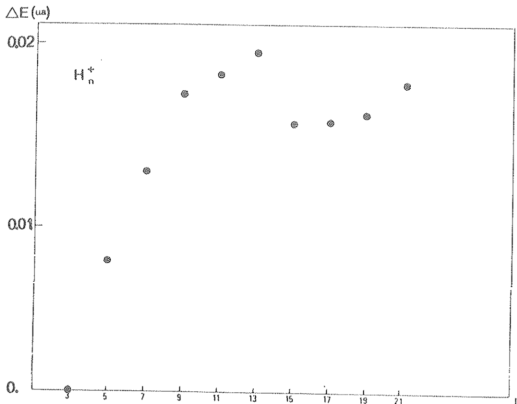
Figure 1.8 : Différence entre l'énergie calculée (HF TZP) pour l'agrégat H_n^+ et l'énergie du système constitué de H_3^+ et de ((n-3)/2) H_2 infiniment éloignés.
