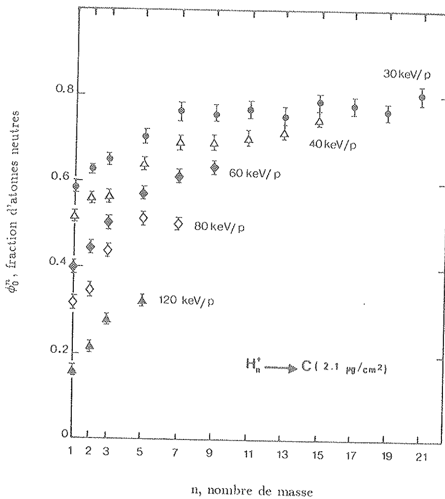
Figure 3.12 : Variation de la fraction d'atomes neutres \phi_0^n par proton incident en fonction du nombre de masse pour différentes vitesses des projectiles [15].
