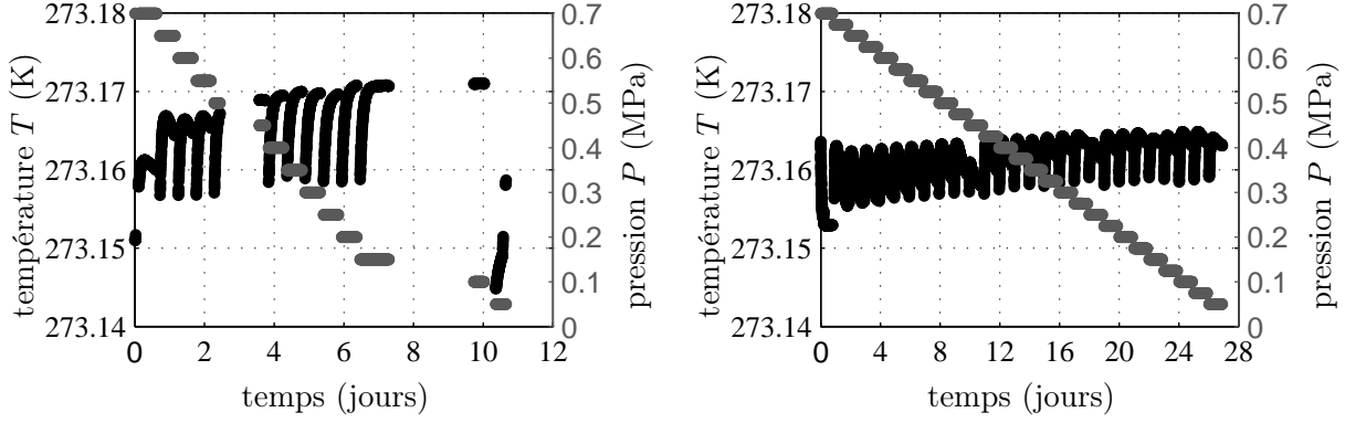
FIG. 4.6 – Variations de la température (points noir) et de la pression (points gris) à l'intérieur du résonateur lors de l'isotherme réalisée en mai 2009 (gauche) et celle réalisée en juillet 2009 (droite)
