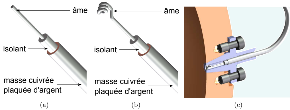
FIG. 4.39 – Dessins représentant (a) schématiquement une antenne micro-onde droite , une antenne micro-onde bobine et (c) leur position en paroi du résonateur.
