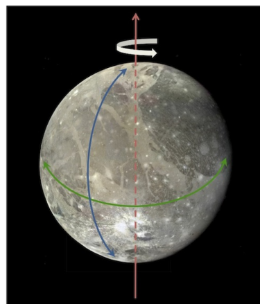
FIGURE 1.14 – Représentation schématique des mouvement de librations en longitude (flèches vertes) et latitude (flèches bleues) de Ganymède. Le satellite tourne autour de son axe (représenté en rouge).
