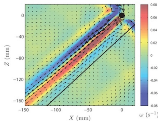
FIGURE 1.6 – Visualisation expérimentale du champ de vitesses (flèches) et de vorticit  ( chelle de couleurs) de l'onde inertielle g n r e par l'ocillation d'un cylindre. (extrait de Cortet et al. (2010)).
