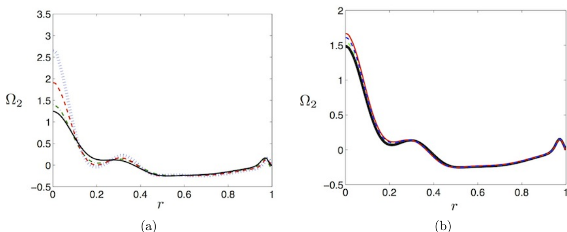
FIGURE 7.4 – Vitesse angulaire associée à l’écoulement zonal, \Omega_2 = \overline{u_\theta}/(r\varepsilon^2) , dans un cylindre de rapport d’aspect \alpha = 2 pour \omega = 1,27 , (a) avec \varepsilon = 0,05 et différentes valeurs du nombre d’Ekman : E = 10^{-4} (courbe noire continue), E = 8 \times 10^{-5} (courbe tirets-pointillés verts), E = 6 \times 10^{-5} (courbe en tirets rouges), E = 4 \times 10^{-5} (courbe en pointillés bleus); (b) pour E = 8 \times 10^{-5} et différentes amplitudes de libration : \varepsilon = 0,1 (courbe noire en gras), \varepsilon = 0,08 (courbe tirets-pointillés verts), \varepsilon = 0,02 (courbe en tirets bleus), \varepsilon = 0,01 (courbe rouge continue).
