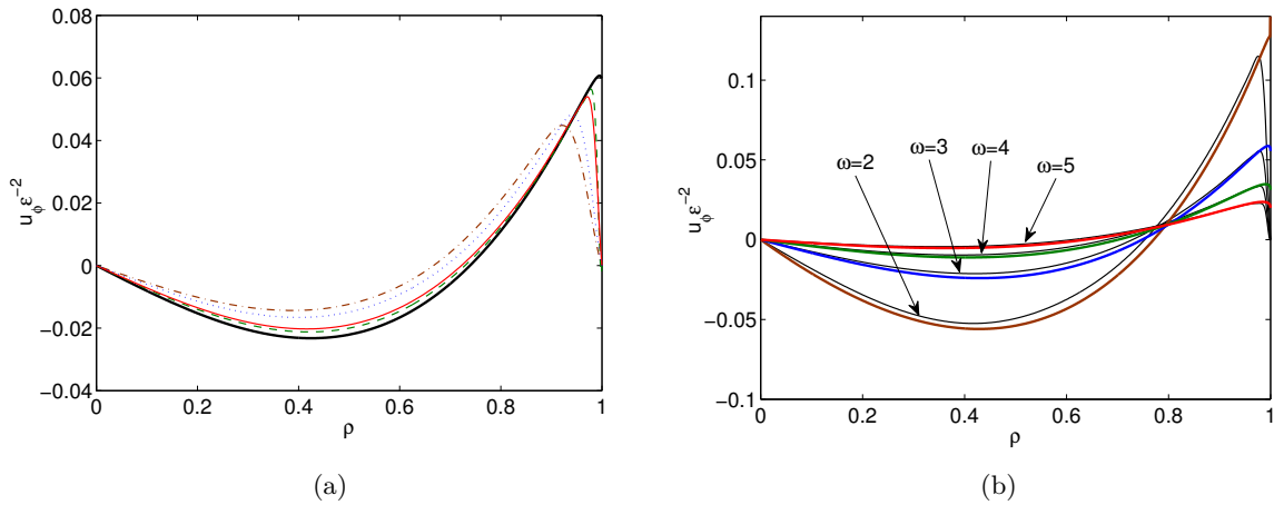
FIGURE 4.5 – Écoulement stationnaire azimutal u_{\phi_2} = u_\phi \varepsilon^{-2} dans une sphère. Comparaison des résultats numériques obtenus dans le plan équatorial ( z = 0 ) avec les résultats théoriques (courbe noire). (a) Pour une fréquence et une amplitude de libration fixes ( \omega = 3 ; \varepsilon = 0,1 ) et différents nombres d'Ekman (courbe marron en tirets-pointillés : E = 10^{-3} ; courbe bleue en pointillés : E = 5 \times 10^{-4} ; courbe rouge continue : E = 10^{-4} ; courbe verte en tirets : E = 4 \times 10^{-5} ); (b) pour un nombre d'Ekman et une amplitude fixes ( E = 5 \times 10^{-5} , \varepsilon = 0,01 ) et différentes fréquences de libration. Les courbes noires représentent les profils obtenus numériquement et les courbes en couleurs sont les solutions théoriques correspondantes.
