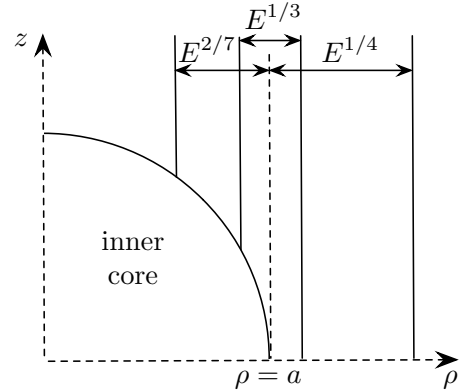
FIGURE 3.6 – Structure des couches de Stewartson. La couche interne a une épaisseur E^{1/3} et les couches externes ont une épaisseur E^{1/4} et E^{2/7} .
