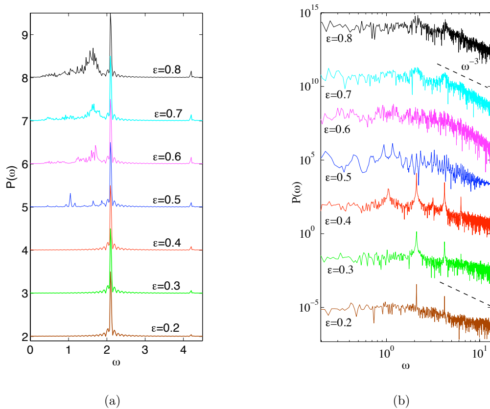
FIGURE 6.8 – (a) Moyenne axiale du spectre temporel de la vitesse radiale u_r en r = 0,2 pour \omega = 2,1 , E = 4 \times 10^{-5} et différentes amplitudes de libration longitudinale \epsilon . (b) Spectre temporel de la vitesse axiale mesurée au voisinage de la paroi extérieure au point (r = 0,99 ; z = 0,1) pour les mêmes paramètres que la figure (a).
