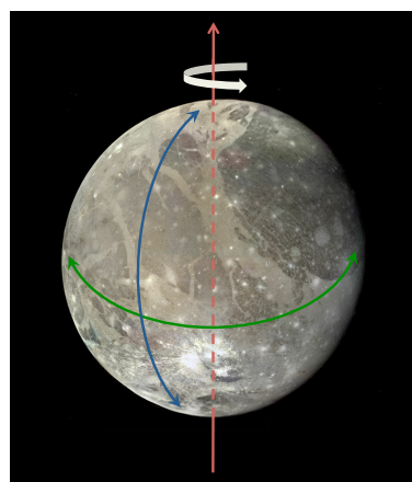
FIGURE 1.14 – Représentation schématisée des mouvement de libration en longitude (flèches vertes) et latitude (flèches bleues) de 18 Ganymède. Le satellite tourne autour de son axe (représenté en rouge).
