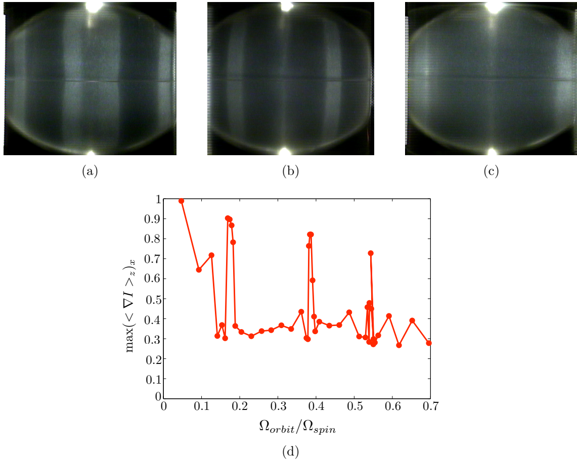
FIGURE 7.8 – Détermination des modes résonants par visualisation directe (particules de Kalliroscope) pour E = 1,45 \times 10^{-5} , \beta = 0,04 et (a) \Omega_R = 0,178 , (b) \Omega_R = 0,384 et (c) \Omega_R = 0,55 . (d) Gradient d'intensité lumineuse en fonction de \Omega_R pour E = 1,45 \times 10^{-5} et \beta = 0,04 .
