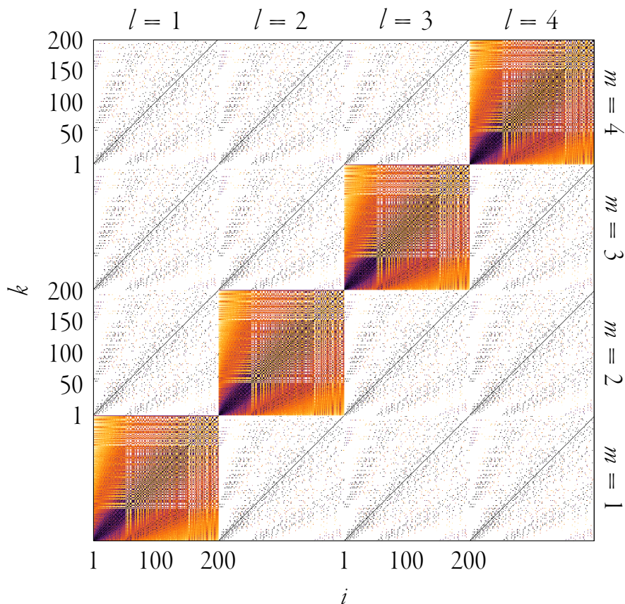
FIGURE III.2 – « Pattern » de la matrice Jacobiennne calculée pour N = 200 et P = 4 . Les couplages locaux entre niveaux expliquent les blocs diagonaux pleins car chacun des états est couplé aux autres par les collisions. En revanche les couplages non locaux ne peuvent être que radiatifs, d'où les autres blocs creux.
