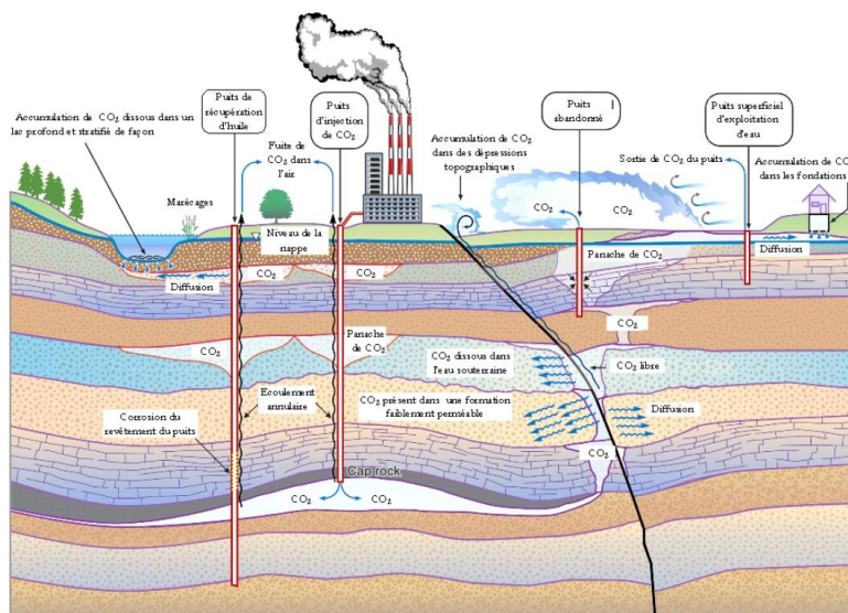
Figure 18 : Schématisation des risques associés au stockage géologique du CO 2 . Graphique : INERIS, source : Hovorka et al (2004).
