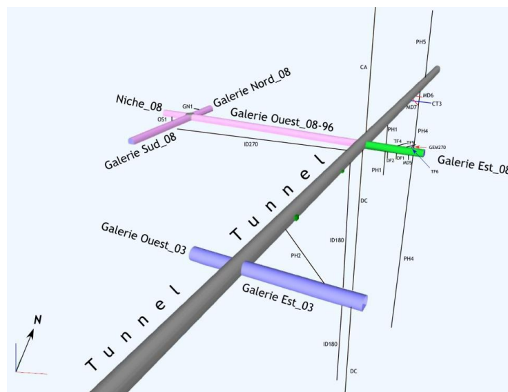
Figure 29 : Plan du laboratoire souterrain IRSN de Tournemire
