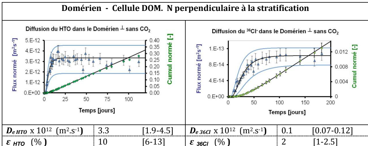
Figure 50 : Courbes de flux et de cumul avec les valeurs des paramètres diffusifs correspondants ( D_e et \epsilon ) des traceurs HTO, 36 Cl obtenues dans la cellule DOM.N (Domérien testé à l'équilibre, perpendiculairement à la stratification)
