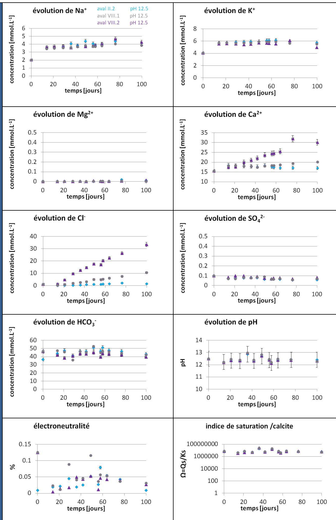
Figure 105 : Superposition des évolutions chimiques enregistrées dans les réservoirs avals de chaque configuration expérimentale appliquée aux pâtes de ciment (cellule II.2 ;VIII.1 et VIII.2).
