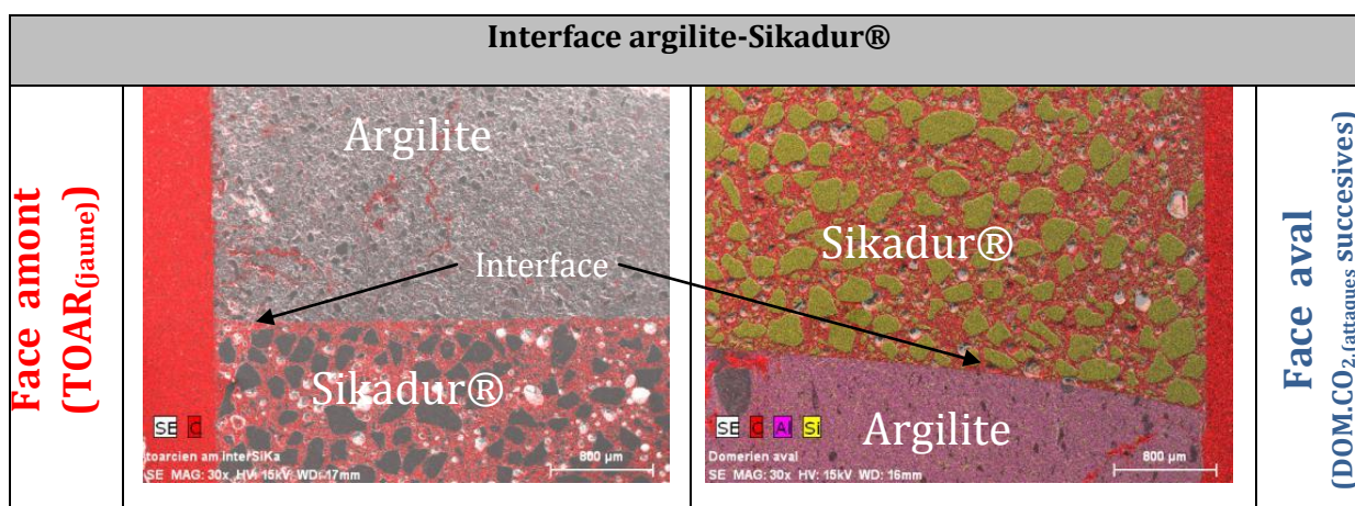
Figure 63 : Observations MEB de l'interface argilite-Sikadur® après l'attaque acide sur deux échantillons en amont (TOAR(jaune) ) et en aval (DOM \text{CO}_2 attaques successives). Photographie de la zone étudiée (SE : Secondary electron) avec cartographie Carbone (C, rouge), silicium (Si, jaune) et aluminium (Al, mauve).
