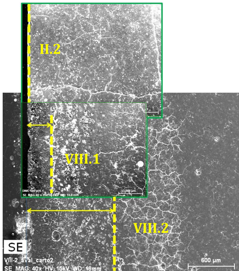
Figure 118 : Comparaison des fronts de pénétration pour les trois cellules (II.2, VIII.1 et VIII.2) testant les pâtes de ciment à pH=8 et pH=5.
