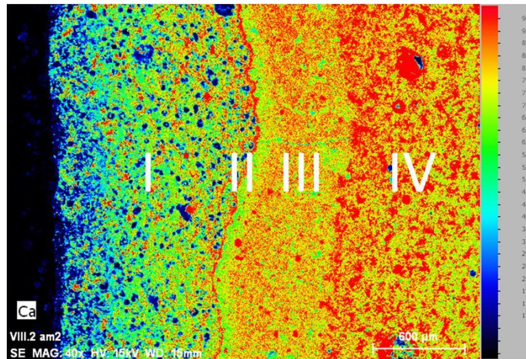
Figure 112 : Localisation des zones altérées sur l'échantillon VIII.2
