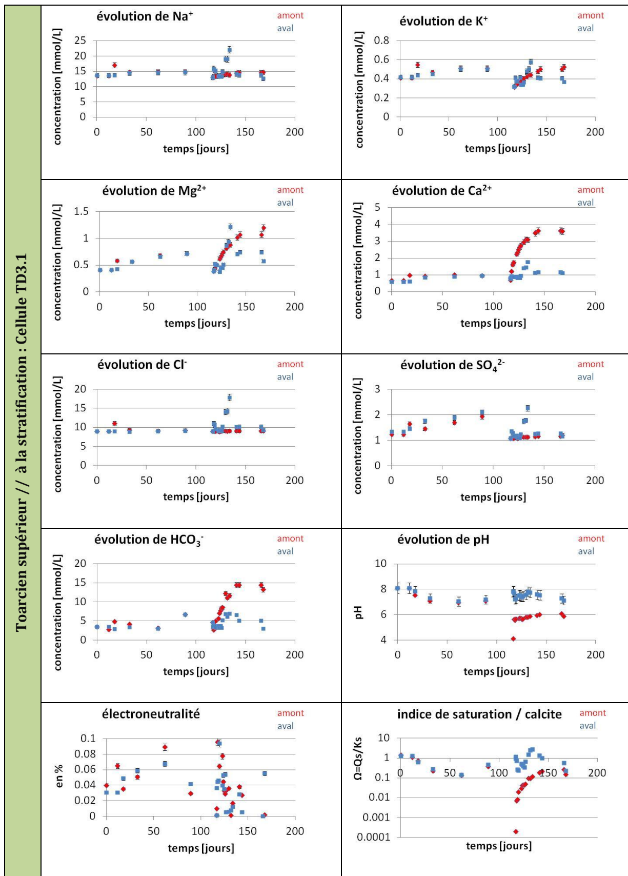
Annexe 14 : Monitoring chimique des réservoirs amont et aval de la cellule PEEK TD3.1 (échantillon de Toarcien Supérieur prélevé proche de la fissure).
