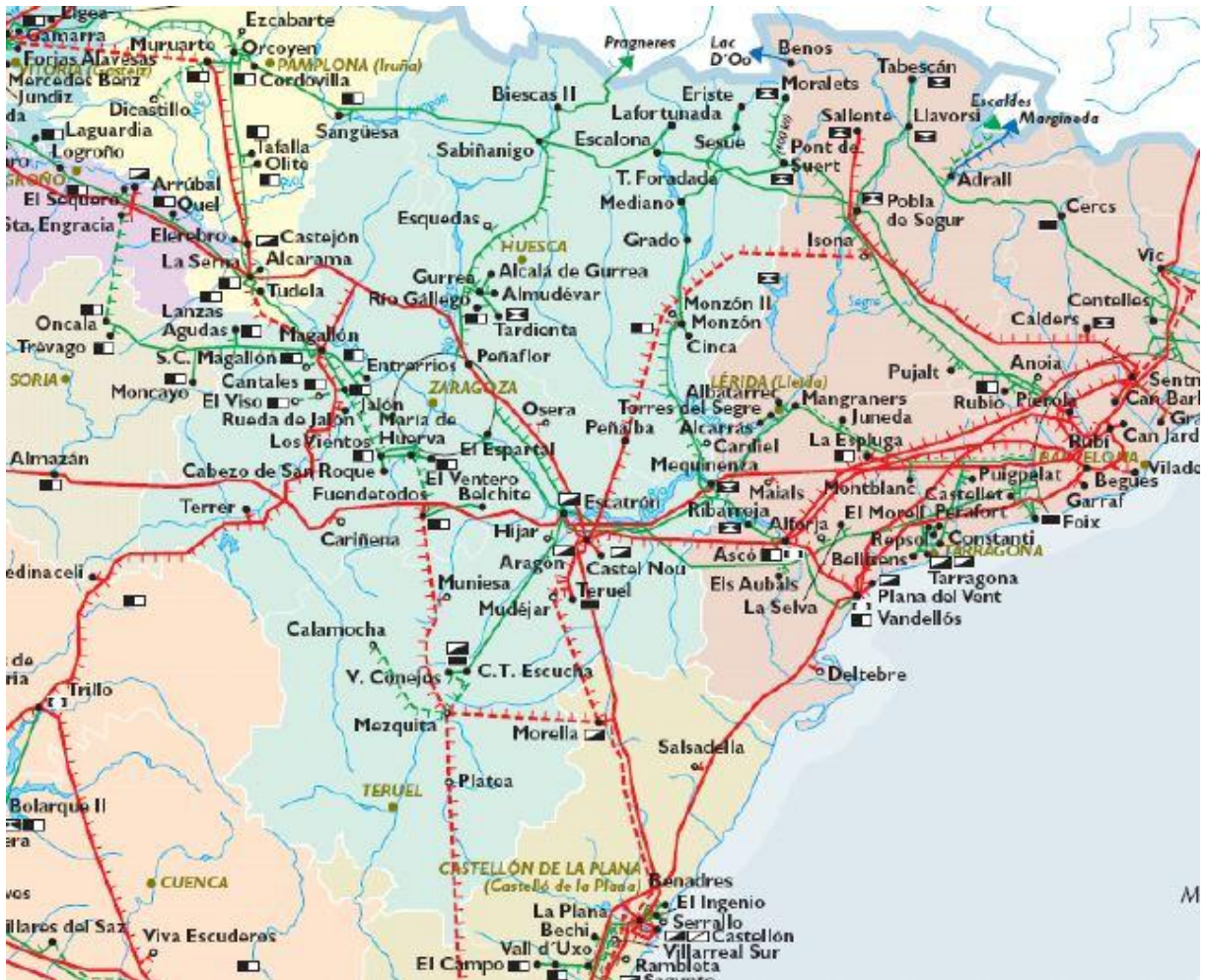
Carte des centrales électriques, dans http://imageshack.us/f/808/71541264.png/
