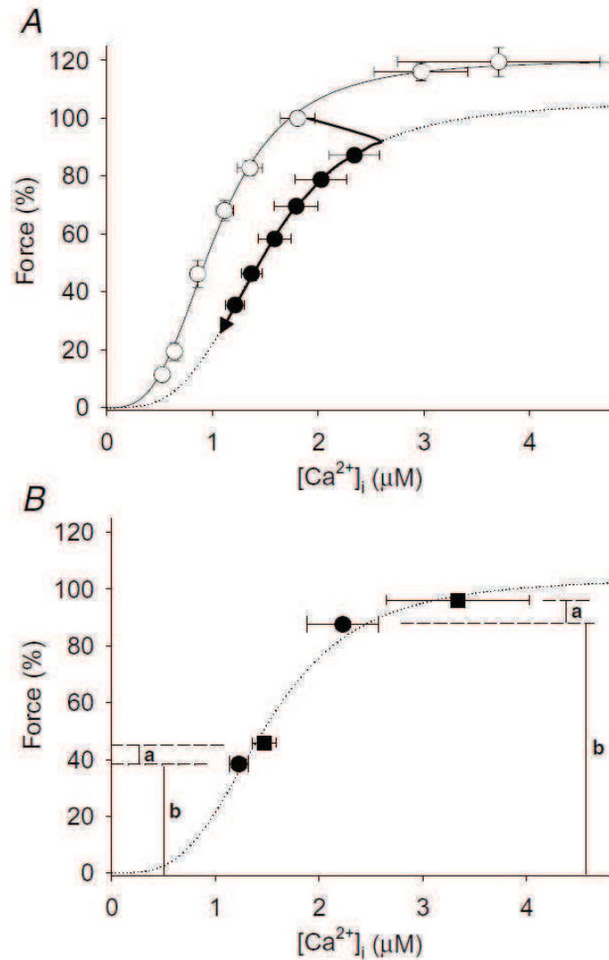
Figure 10. Relation force- [Ca^{2+}]_i sur le muscle flexor digitorum brevis de souris obtenue A) avant l'exercice (cercle blanc) fatigant par des stimulations tétaniques de 350ms pour une fréquence de 15 à 150 Hz, et après la fatigue (cercle noir) pour des contractions tétaniques de 350ms à 70 Hz correspondant à 90, 80, 70, 60, 50 et 40% de la force initiale. B) La relation force- [Ca^{2+}]_i venant du point A obtenu pendant la fatigue avec la stimulation standard (cercle noir) et interpolée (carré noir) correspondant à 90 et 40% de la force initiale. (figure tirée de Place et al., 2008).
