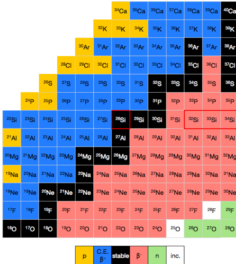
FIGURE 2.4: Noyaux de la couche sd
