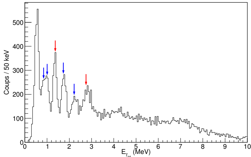
FIGURE 4.22 : Spectre \gamma mesuré à E_{c.m.} = 6,6 MeV en imposant une coïncidence entre les BGO et le DSSD. Les flèches indiquent les transitions provenant des voies de fusion-évaporation ^{12}\text{C}(^{16}\text{O},\alpha)^{24}\text{Mg} (en rouge) et ^{12}\text{C}(^{16}\text{O},p)^{27}\text{Al} (en bleu).
