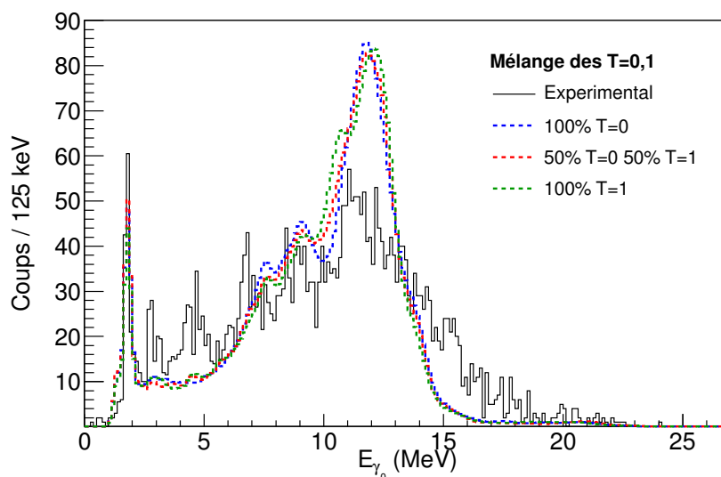
FIGURE 4.35: Simulations numériques pour E_{c.m.} = 6,6 MeV n'incluant que des états T = 1 , différents mélanges d'isospin ont été testé pour les états T = 0,1 et sont comparés aux données expérimentales.
