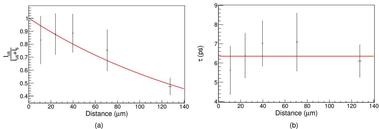
FIGURE 3.44: (a) Évolution du rapport des intensités des composantes lente et rapide en fonction de la distance entre la cible et le ralentisseur pour la transition 1/2^+ \rightarrow 3/2^+ du ^{33}\text{Si} . La courbe en rouge est un ajustement exponentiel des données. (b) Temps de vie extrait pour chaque distance en utilisant l'ajustement du panneau de gauche. Un ajustement constant des différents points nous donne le temps de vie de l'état 1/2^+ à 1,010 MeV.
