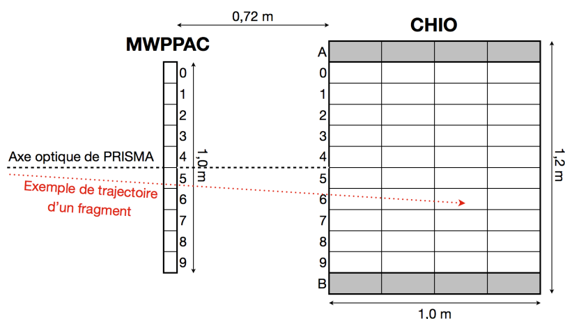
FIGURE 3.25: Schéma des détecteurs autour du plan focal de PRISMA. La segmentation des détecteurs permet une bonne reconstruction de la trajectoire des ions (flèche rouge).
