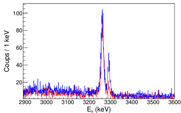
(b) ^{36}\text{S} : 2_1^+ \rightarrow 0_1^+
