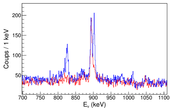
(a) ^{36}\text{S} : 4_1^- \rightarrow 3_1^-, 3_1^- \rightarrow 2_1^+
