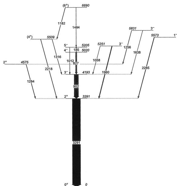
FIGURE 3.34: États du ^{36}\text{S} observés lors de l'expérience ^{36}\text{S}+^{208}\text{Pb} [53] avec les prédictions sur les durées de vie obtenues avec l'interaction PSDPF. La largeur des flèches sur le panneau de gauche est proportionnelle à l'intensité relative des transitions. Toutes les énergies sont en keV sur le spectre.
