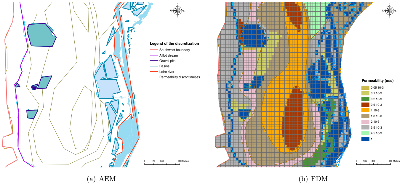
FIGURE 2.14 – Discrétisation du domaine pour chacune des méthodes AEM et FDM avec une résolution de 50 m. Les AEM utilisent l’algorithme de Douglas-Peucker avec une tolérance de 50 mètres. Les FDM utilisent une taille de grille de 50 mètres.
