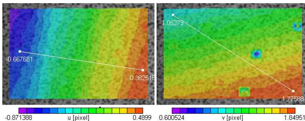
FIG. 4.15 – Déplacement calculé entre une image de référence sans filtre et une image acquise pour le filtre centré à 1.310\mu m .
