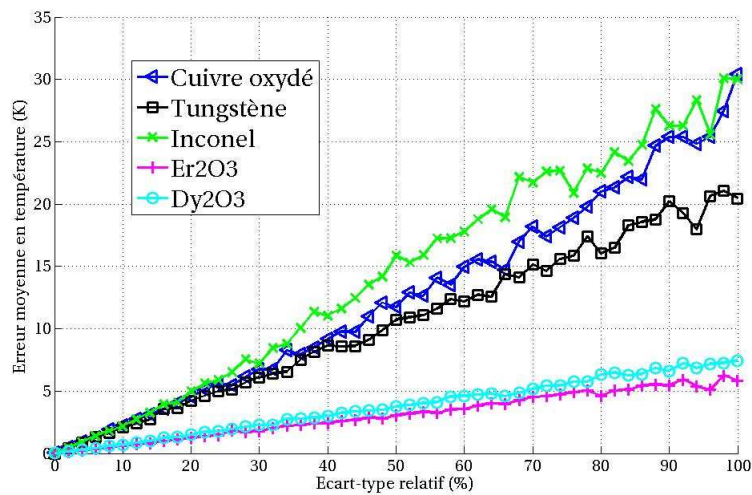
FIG. 2.20 – Moyenne de l’erreur en température \bar{\varepsilon}(T) en fonction de l’écart-type normalisé (ie 100% représente 5^{\circ}C pour la température de luminance et 0.01sr^{-1} pour la réflectivité bidirectionnelle).
