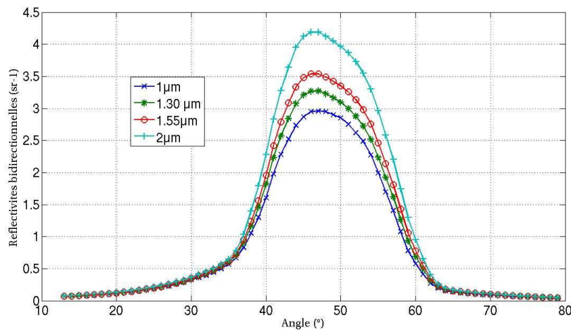
FIG. 1.9 – BRDF dans le plan d'incidence, avec un angle d'incidence de 45°, pour un échantillon de Tungstène et pour quatre longueurs d'onde proche infrarouge.
