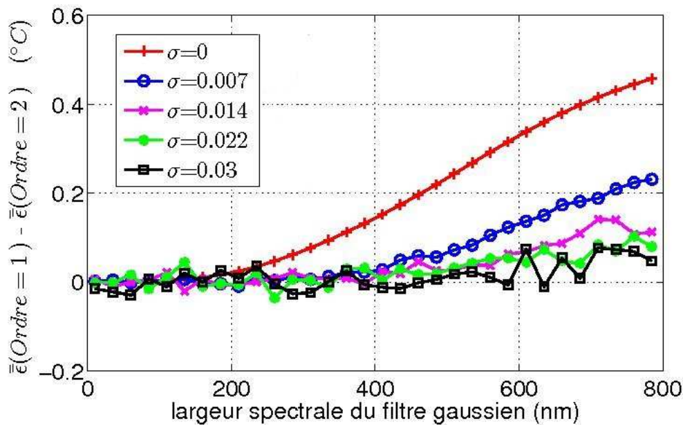
FIG. 3.5 – Écarts des paramétrages aux ordres 1 et 2 sur les erreurs moyennes des températures estimées en fonction de la largeur spectrale du filtre pour un signal détecteur généré avec un filtre gaussien et pour quatre niveaux de bruit de 0 à 3%.
