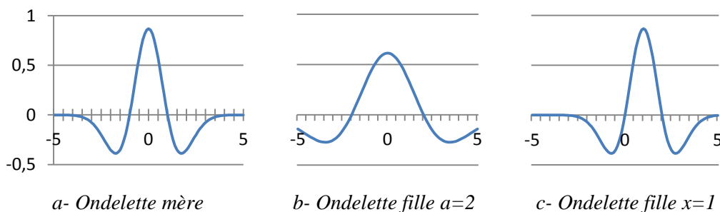
Figure 2.21 – Paramétrisation des ondelettes (chapeau mexicain)
