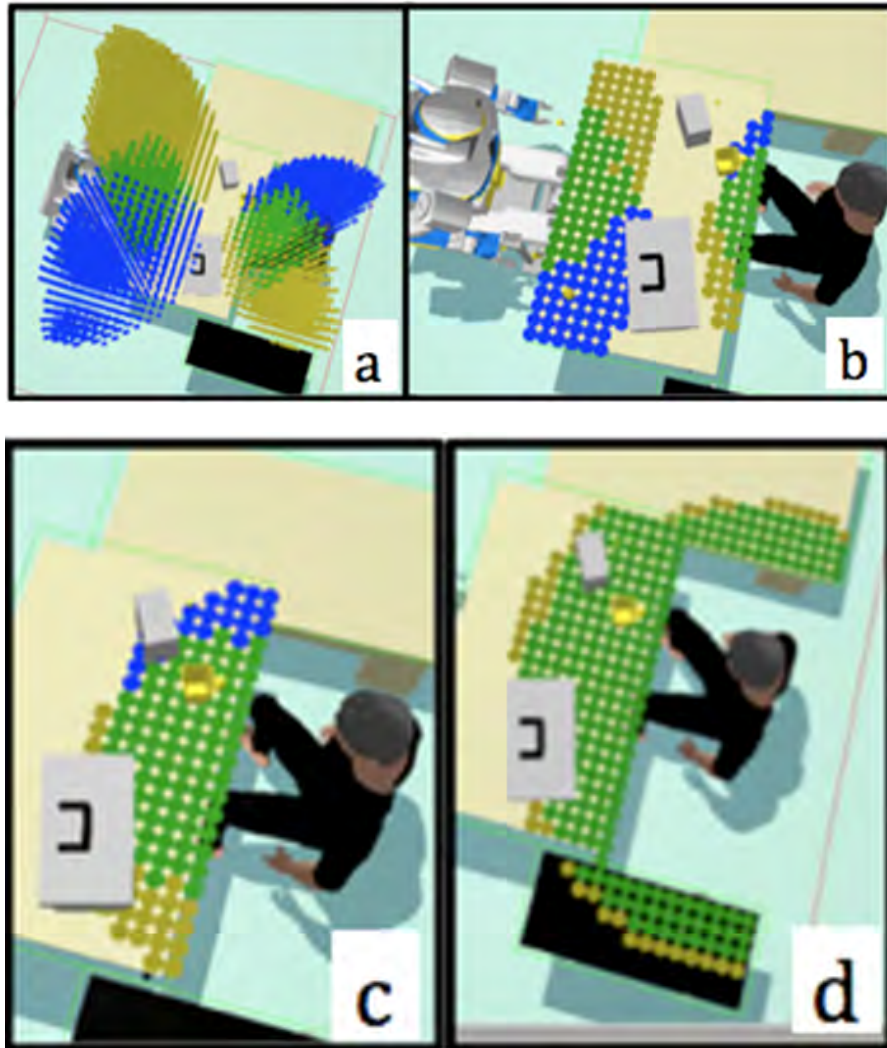
Figure E.4: Carte d'atteignabilité pour un Homme et HRP2 à partir de leur état courant: (a) en 3D et (b) sur le plan de la table. On voit ce qui est atteignable uniquement par la main gauche (jaune), par la main droite (bleu) et par les deux mains (vert). Dans le cas présent, il n'y a pas d'espace commun si aucun des agents ne s'implique et réalise un effort. (c) montre ce qui est atteignable par l'homme si il tend les bras (d) montre ce qui est atteignable par l'homme si il lui est possible de tendre les bras et de se tourner.
