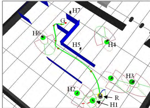
Figure E.10: Le robot Jido (R) doit guider l'homme (H1) vers le but (G). La trajectoire en vert montre le plan calculé par notre planificateur.
