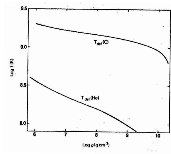
FIG. 4.1 – Valeur de T_{\text{def}} pour l'hélium et le carbone en fonction de la pression ((Nomoto 1982a))
