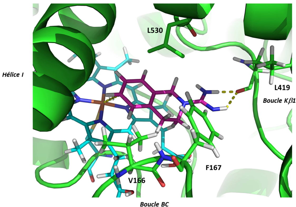
Figure IV-14 : Positionnement majoritaire de la débrisoquine au sein du site actif du CYP2U1 (cluster 1) propice à la formation de la 6-hydroxydébrisoquine. L'apoprotéine est en vert, l'hème en bleu et la débrisoquine en violet.
