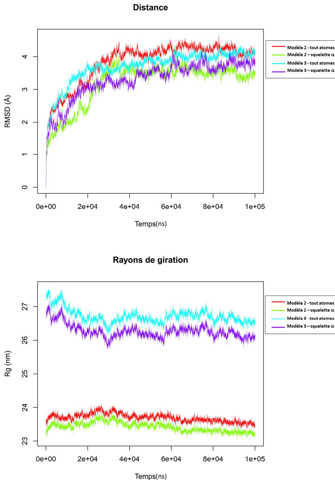
Figure II. 16 : Evolution du RMSD et du rayon de giration lors de la dynamique effectuée sous NAMD/CHARMm pour les deux modèles de CYP2U1 (modèles 2 et 3 - calcul Ptraj) à une température de 300K. Les données sont obtenues soit en considérant tous les atomes soit seulement le squelette alpha.
