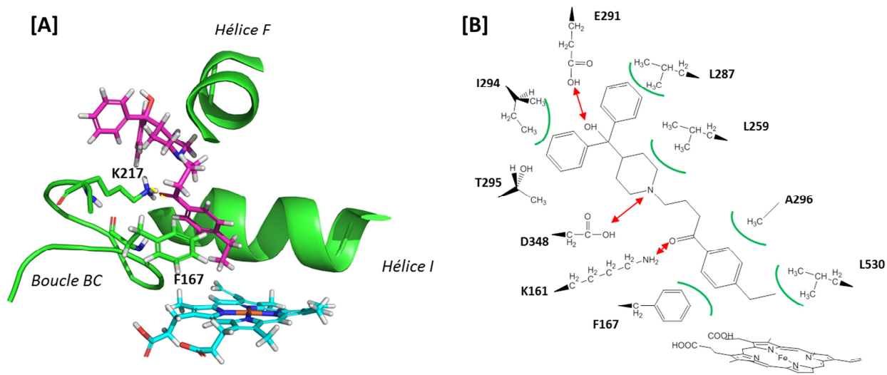
Figure IV-24 : [A] : Positionnement de l'éthylterféfadone au sein du site actif du CYP2U1 pour une entrée du substrat par le canal 2ac. L'apoprotéine est en vert, l'hème en bleu et l'éthylterféfadone en violet, [B] : Interactions relevées dans les complexes. Les liaisons hydrogènes et électrostatiques sont représentées par des flèches rouges, les interactions de Van der Waals sont indiquées en vert.
