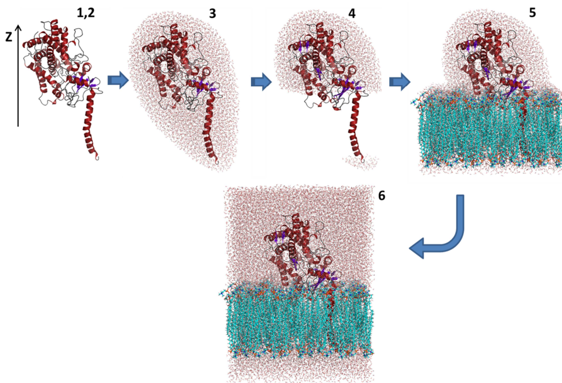
Figure VI-1 : Les étapes de la construction d'un modèle en membrane. La protéine est représentée en cartoon, les molécules d'eau et les phospholipides en bâtons.
