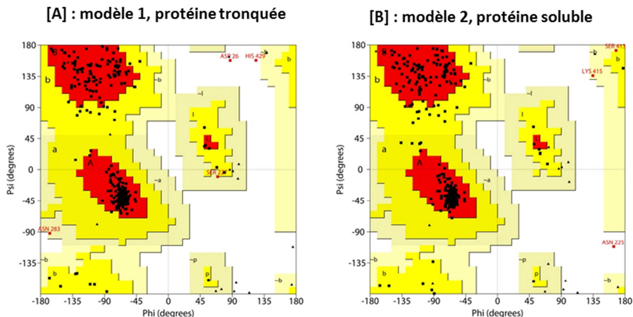
Figure II. 7 : Diagramme de Ramachandran des modèles du CYP2U1. Les triangles correspondent aux glycines et aux prolines de la protéine, les carrés aux autres résidus. Pour le modèle de protéine tronquée [A], 92% des résidus sont situés dans une zone favorable, 6.9% dans des zones défavorables, 0.1% dans des zones interdites. Pour le modèle de protéine tronquée [B], 90.5% des résidus sont situés dans une zone favorable, 9% dans des zones défavorables, 0.5% dans des zones interdites.
