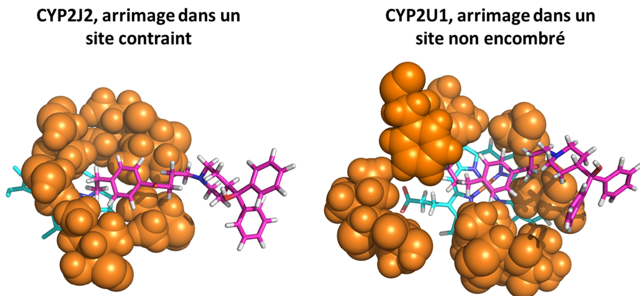
Figure IV-25 : Les résidus de la première couronne lors de l'arrimage de l'éthylterfénadone Les résidus de la première couronne sont représentés en sphères de Van der Waals orange, l'analogue de terfénadone et l'hème en bâton.
