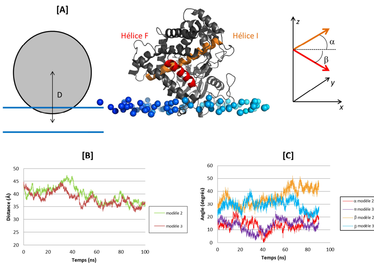
Figure II. 17 : Orientation de la membrane au cours de la dynamique. [A] gauche : Illustration de la distance D mesurée entre les centres de masses des C1 des lipides et C\alpha du CYP2U1. centre et droite : Orientation des hélices I et F du CYP2U1 par rapport à la membrane (l'hélice I est en orange, l'hélice J en rouge, un plan représentant la membrane est illustré par des sphères bleues). [B] Evolution de la distance D au cours de la dynamique. [C] : Evolution des angles \alpha et \beta au cours de la dynamique.
