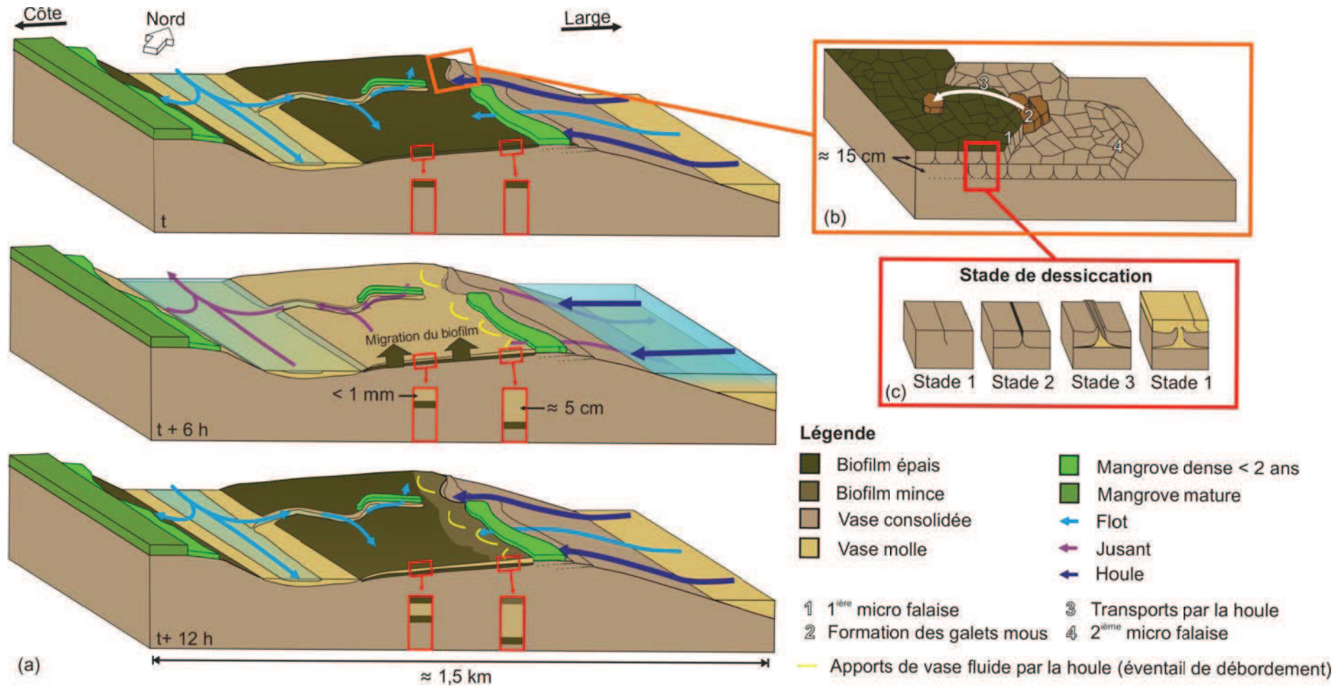
Figure 5.24: Evolution morphologique de la partie intertidale d'une vasière. (a) Sédimentation sur la vasière engendrée par la marée et la houle, au cours d'un cycle de marée ; (b) Faciès d'érosion et création des galets mous par la houle en front de mer; (c) Stades de dessiccation de la surface de la vasière.
