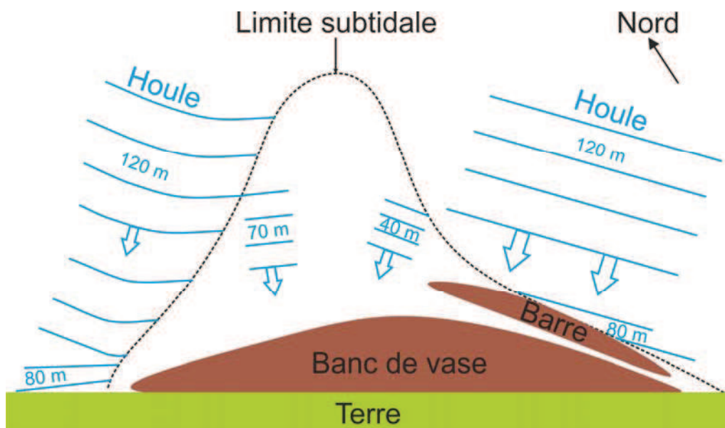
Figure 3.4 : Schéma synthétique des variations des longueurs d'ondes des houles et de leurs réorientations, lors de leurs interactions avec la partie subtidale d'un banc de vase. L'amortissement des houles varie en fonction de leur position par rapport au banc mais ne change pas lors de leur propagation vers la côte. Le transport sédimentaire qui suit l'orientation des houles est concentré vers le centre du banc.
