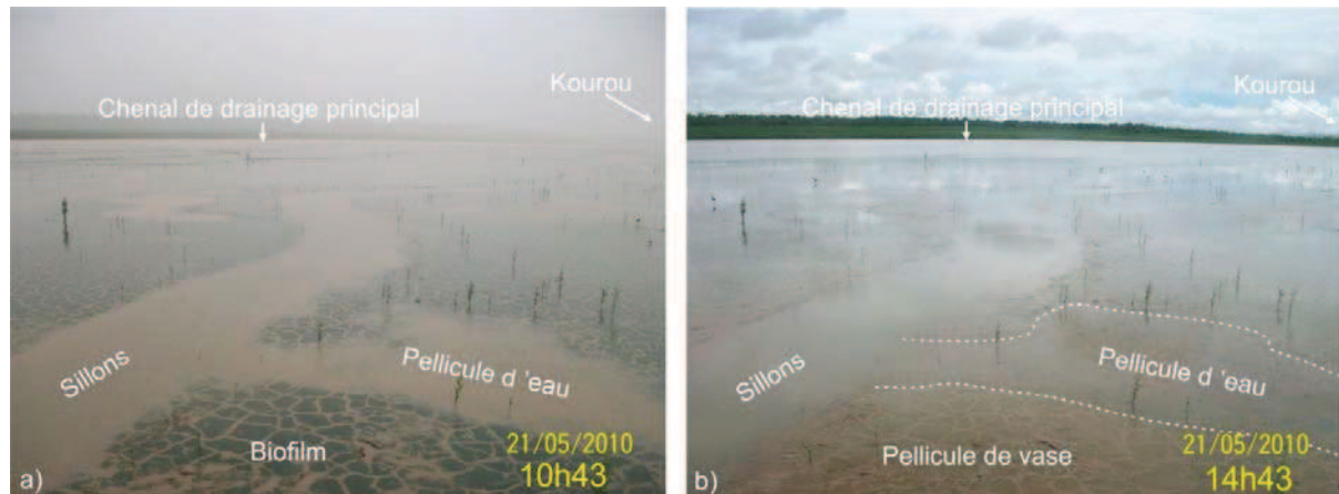
Figure 5.9 : Matière en suspension au flot et au jusant. Photos prises par la station d'observation sur la vasière de Kourou SE au flot (a) et au jusant (b).
