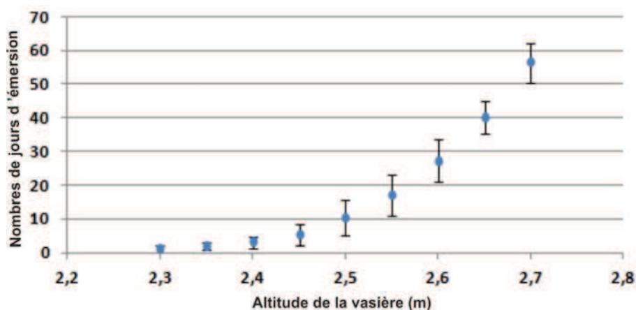
Figure 5.3 : Moyenne du nombre de jours d'émergence de la vase à Kourou, en fonction de l'altitude par rapport au zéro hydrographique, pour la période 1950-2008. Le nombre de jours d'émergence par an augmente rapidement pour les altitudes supérieures à 2,4 m.
