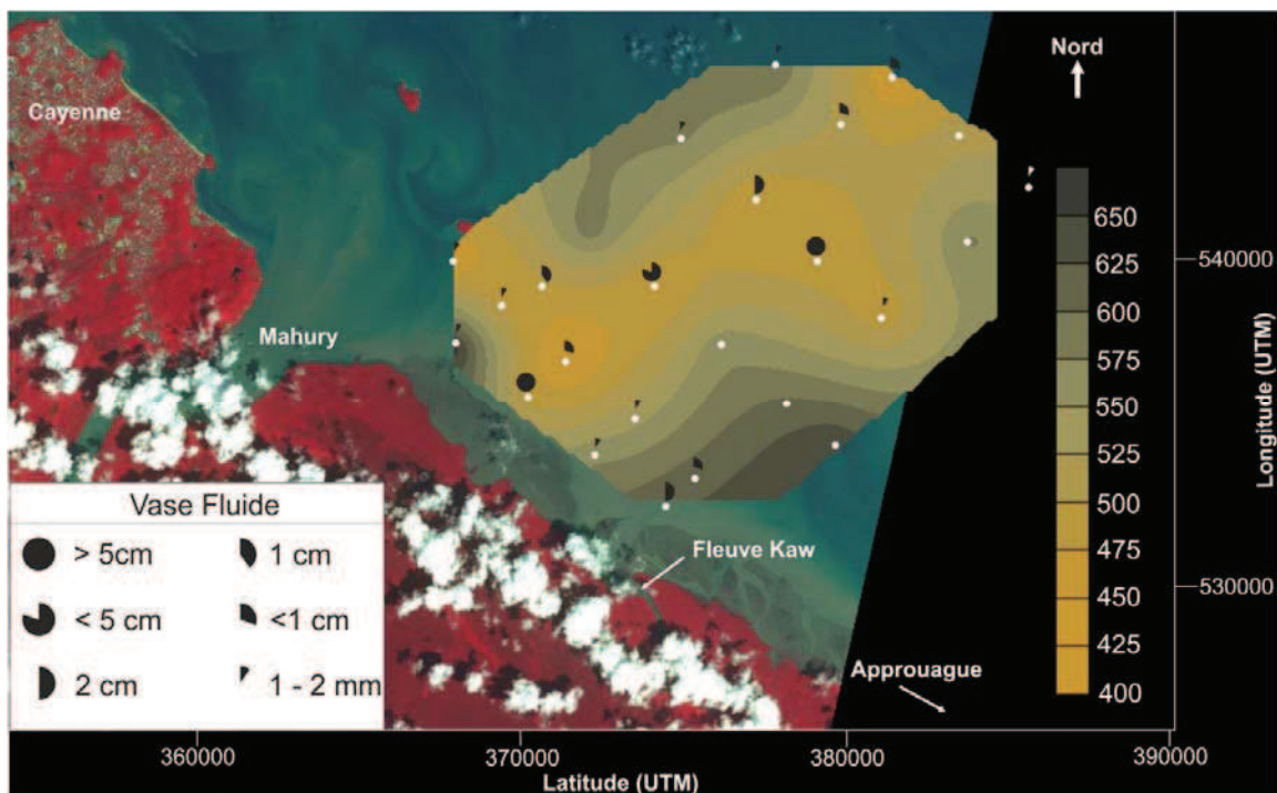
Figure 4.8 : Concentration des vases subtidales pour le banc de Kaw le 26/10/2011. Les points blancs correspondent à la position des prélèvements des sédiments de surface. Les informations sur la vase fluide correspondent à l'épaisseur des dépôts à la surface du sédiment prélevé. Extrait d'une image satellite SPOT 5.
