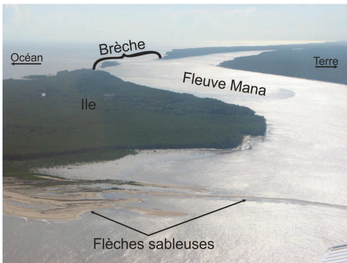
Figure 3.15 : Photo aérienne de l'embouchure du fleuve Mana en 2003, prise par C.Proisy.
