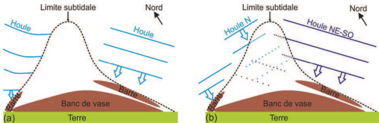
Figure 4.15 : Schémas des différentes hypothèses d'orientation des barres vaseuses par la diffraction (a) ou la filtration (b) des houles.
