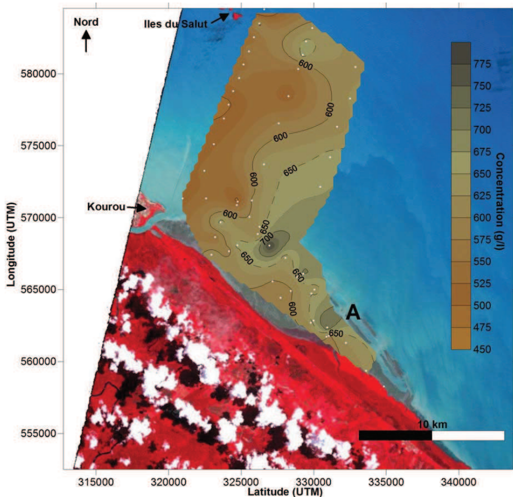
Figure 4.6 : Concentration des sédiments de surface pour le banc de Kourou le 15/04/2003 (Gardel et Gratiot, 2004). Les points blancs correspondent à la position des prélèvements des sédiments de surface. Extrait d'une image satellite SPOT 5.
