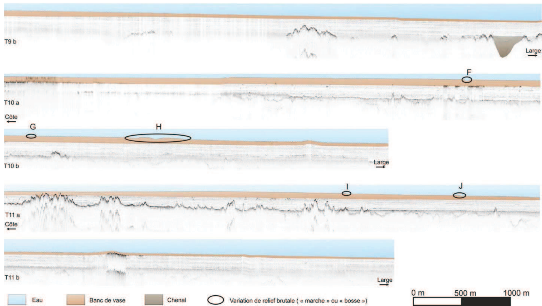
Figure 4.5: Profils sismiques interprétés. Mesure le 16/10/10 au large de Kourou. Certains ont été coupés en deux parties (a et b) pour plus de commodité.
