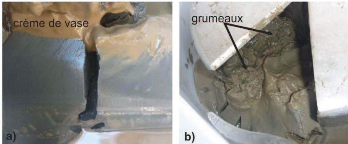
Figure 4.9: Photo de prélèvements effectués avec une benne de type Van Veen le 26/10/2011. a) dépôt de crème de vase sur de la vase plus consolidée ; b) vase molle avec un faciès grumeleux à sa surface.
