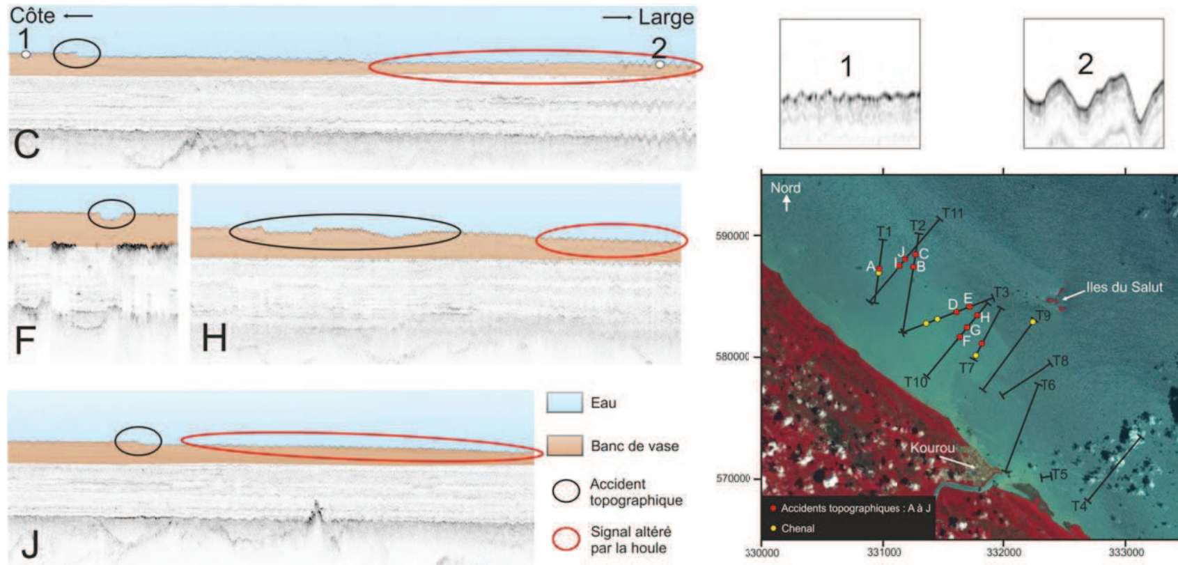
Figure 4.4 : Accidents topographiques de la surface subtidale du banc de vase de Kourou entre le 14/10/2010 et le 18/10/2010. Image satellite SPOT5 acquise le 16/10/2010.
