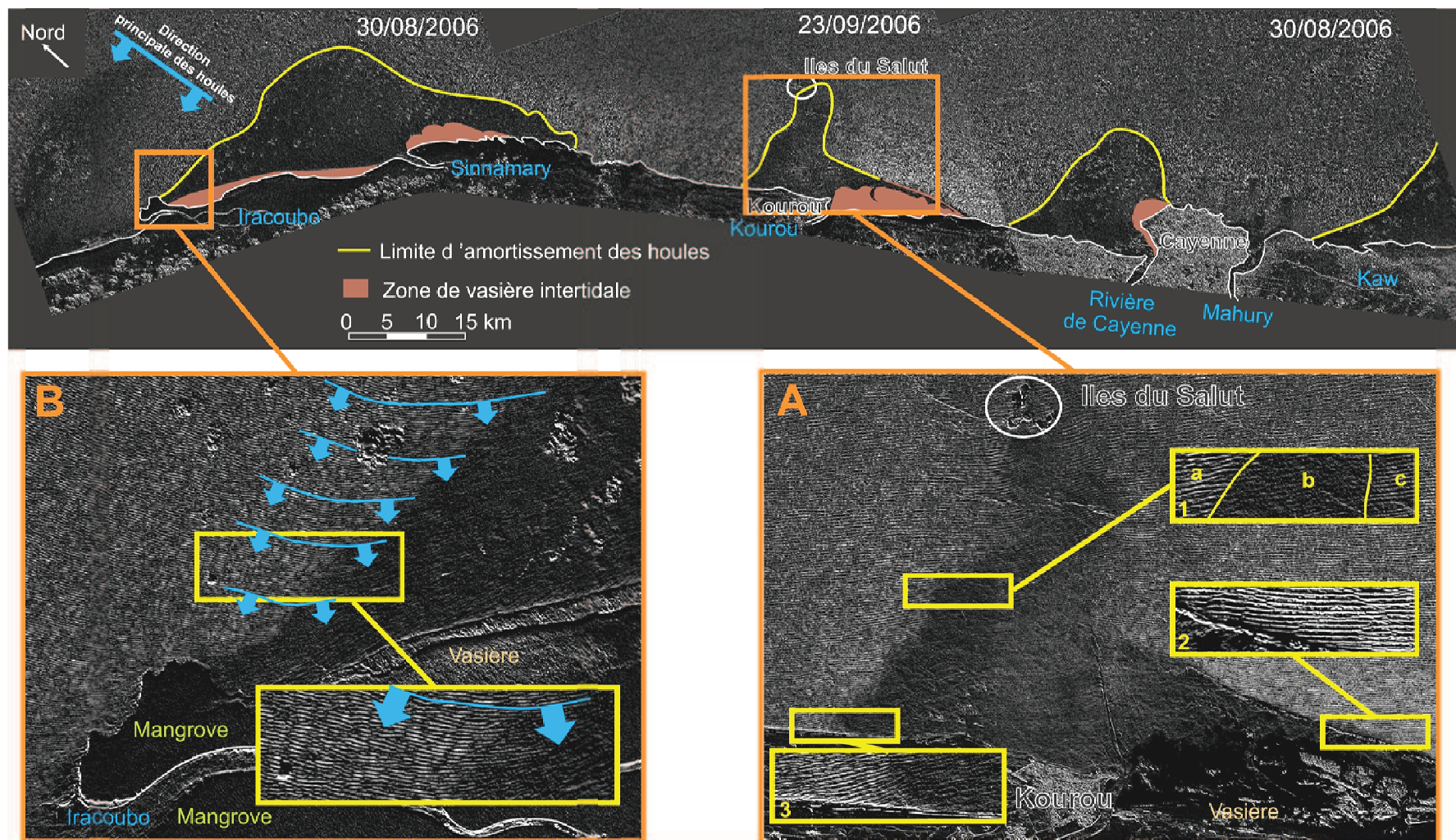
Figure 3.3 : Amortissement des houles le long de la côte de la Guyane française entre Iracoubo et Kaw en 2006. A : Zoom sur la région de Kourou. La variation spatiale de l'amortissement des houles est visible dans l'encadré 1 : (a) houle non amortie, (b) fortement amortie, (c) peu amortie. Les zones encadrées 2 et 3 sont des zoom montrant la différence d'orientation des houles entre l'avant et l'arrière banc ; B : Modification de l'orientation des houles par la partie subtidale du banc de Sinnamary-Iracoubo. Les traits bleus soulignent des crêtes de houles et les flèches correspondent à leur direction de propagation vers la côte. La zone encadrée est un zoom illustrant la diffraction des houles au contact de la vase subtidale. Mosaïque d'images satellites SPOT 5.
