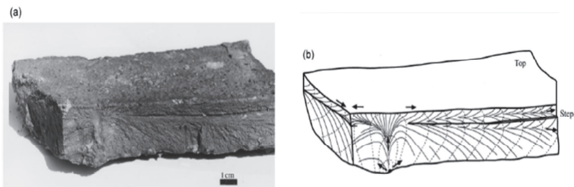
Figure 5.5 : (a) Vue oblique d'un polygone créé par des fentes de dessiccation ; (b) schéma interprétatif de la morphologie de surface associé à la propagation d'une fente. La fente se forme en profondeur puis se développe vers le haut jusqu'à la surface et ensuite latéralement. Weinberger, 1999
