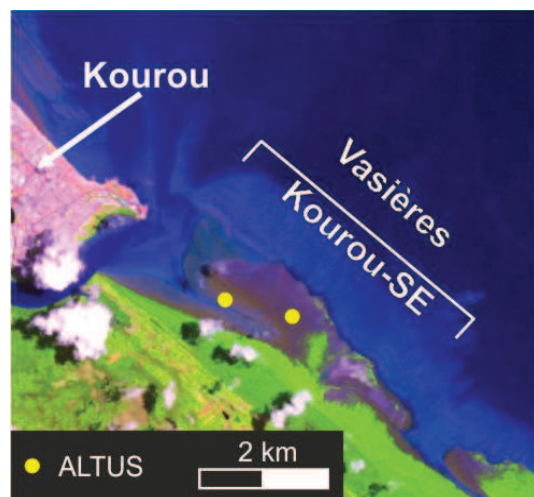
Figure 5.11 : Extrait de la figure position ALTUS et ADCP du chapitre 2.
