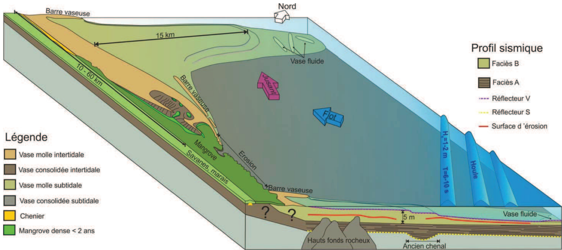
Figure 4.23 : Schéma d'un banc de vase à basse mer dans son ensemble et vue en coupe. Les points d'interrogations marquent l'absence de données concernant la structure en profondeur de la zone intertidale et de la plaine côtière
