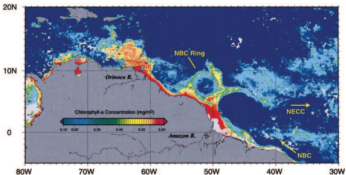
Figure 1.5 : Indice de chlorophylle obtenu à partir de capteurs SeaWiFS (Sea-viewing Wide Field-of-view Sensor) montrant la rétroflexion du NBC et la formation d'un tourbillon (Fratantoni et Glickson, 2002).
