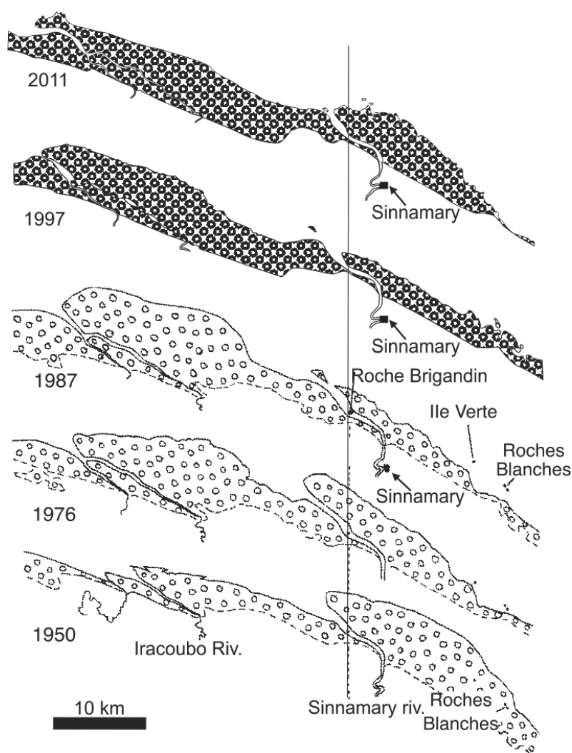
Figure 3.8 : Evolution du littoral et des surfaces de mangrove de la région Sinnamary-Iracoubo, entre 1950 et 2011. Entre 1950 et 1987 la région d'Iracoubo est en accretion puis rentre en érosion au début des années 1990. L'inverse se produit pour la région de Sinnamary. Ce phénomène est provoqué par la migration d'un banc de vase se situant à Sinnamary dans les années 1950 puis vers Iracoubo dans les années 1980. Figure modifiée et actualisée de (Plaziat et Augustinus, 2004).
