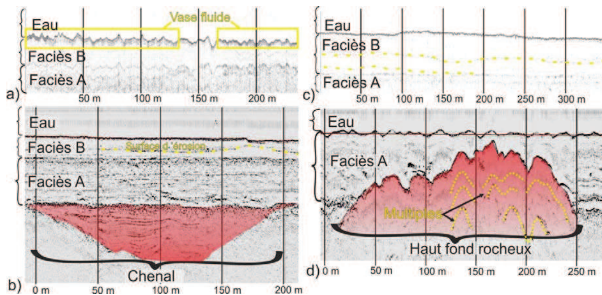
Figure 4.3 : Extraits de profils sismiques représentant les faciès types de la vase fluide (a), d'un chenal (b), de surfaces d'érosion (c) et d'un haut fond rocheux (d).
