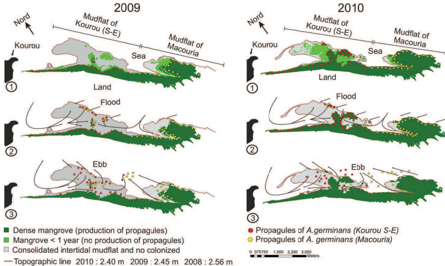
Figure 4.18 : Zone de production des propagules sur les vasières de Macouria et Kourou-SE entre 2008 et 2010 (1) ainsi que leur dispersion en situation de flot (2) et de jusant (3). Les courants ont été établis à partir des résultats d'une étude qui a eu lieu sur la zone de Macouria (zone B) du banc de Kourou en 2006 (Dissaux, 2009), grâce à de nombreuses observations et réflexions sur le terrain et à des mesures ADCP.
