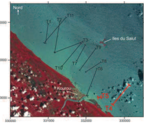
Figure 4.2 : Miniature modifiée de la figure 2.7.
