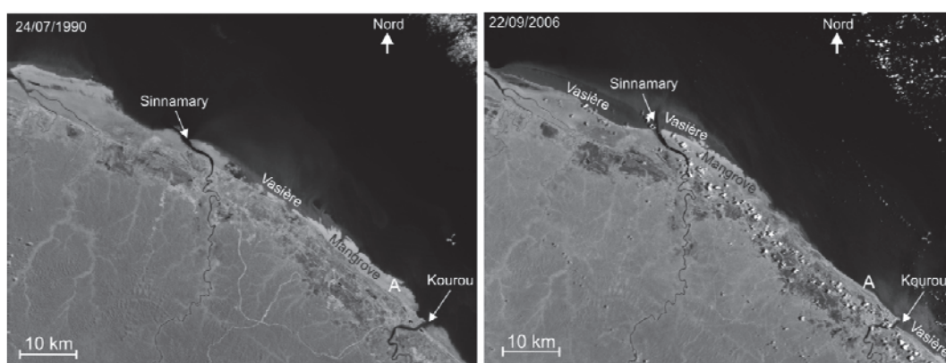
Figure 3.12 : Evolution du littoral dans la région de Sinnamary entre 1990 et 2006. La zone A est composée d'une large mangrove en 1990. En 2006, la mangrove a été érodée, le chenal sableux est réactivé. Le secteur au Sud-Est de l'embouchure de Sinnamary est en colonisation. Images Landsat 5.
