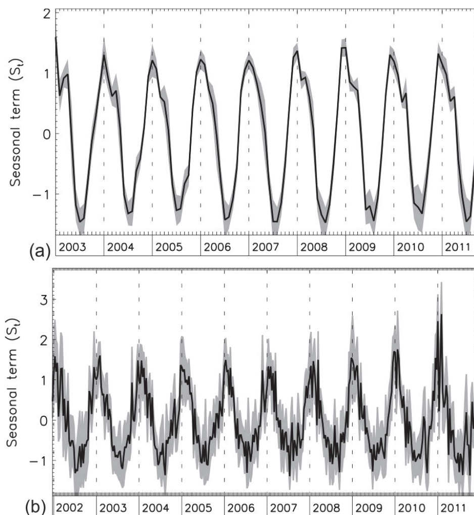
Figure 3.1 : Analyse saisonnière de la force des vents (a) et de la hauteur significative des houles (b), à proximité de la côte des Guyanes, par la méthode Census X11 (expliquée dans le chapitre 2, partie 1).
