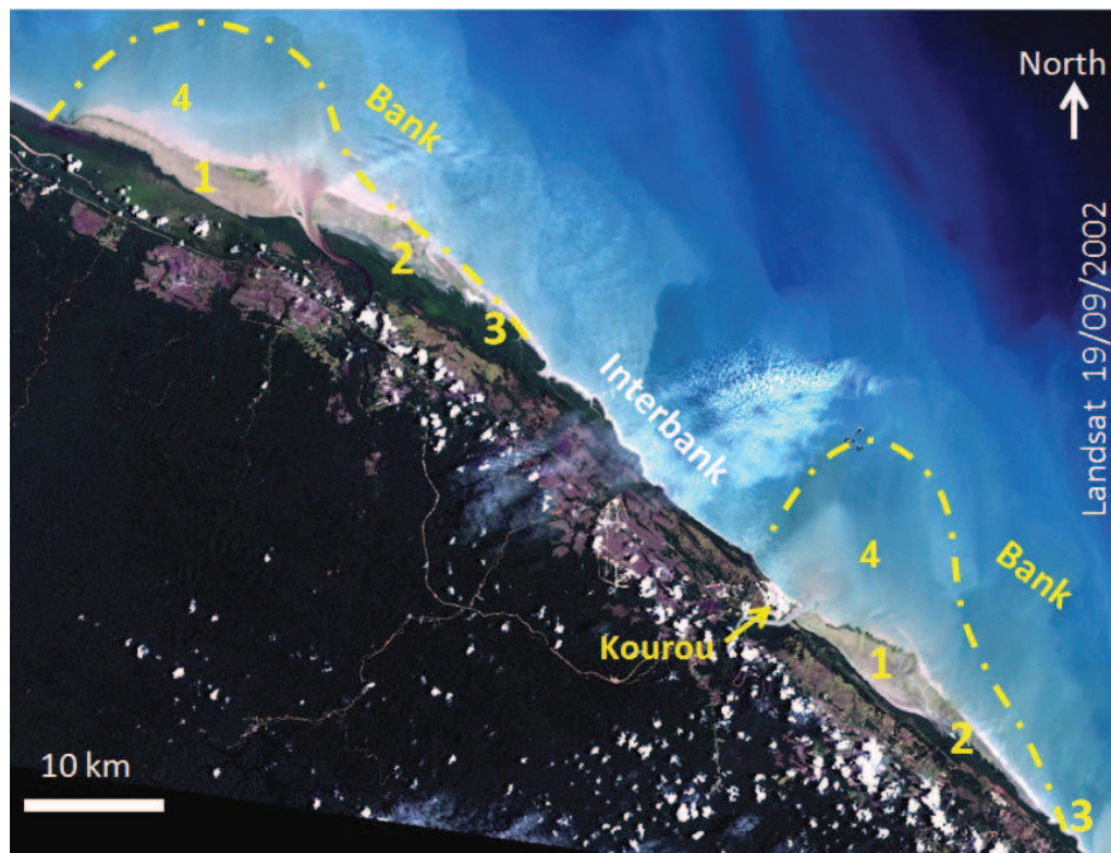
Figure 1.8: Image satellite Landsat 5 de la région de Kourou. Les numéros correspondent aux différentes parties des bancs de vase : 1 Zone en accréation ; 2 Zone en colonisation ; 3 Zone en érosion ; 4 Zone subtidale.
