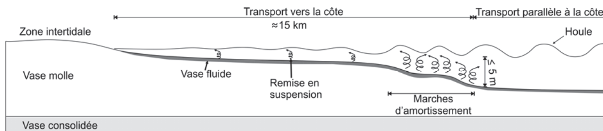
Figure 6.1 : Schéma de l'amortissement des houles sur la zone subtidale d'un banc par la remise en suspension de la vase et son transport vers la côte. La zone d'amortissement maximale est marquée par deux « marches ». En dessous de 5 m de bathymétrie, la houle n'a plus d'effet, le transport sédimentaire s'effectue par les courants, parallèlement à la côte.
