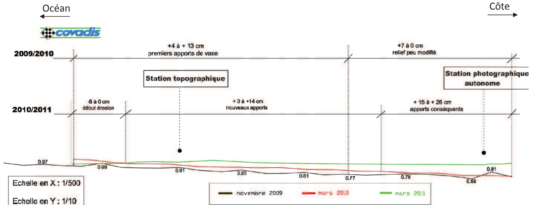
Figure 5.15: Evolution d'un profil topographique sur la zone atelier entre novembre 2009 et mars 2011. La station topographique se situe près du front de mer alors que la station d'observation est dans la zone interne, soumise uniquement à la marée. Les profils ont été réalisés par des relevés au tachéomètre (station topographique) sur le site atelier. Modifiée de Chatelet, 2011.
