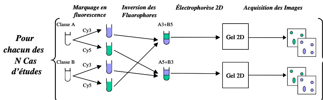
Figure 37 : Principe du Schéma expérimental en « Dye-Swap » . Pour chacun des cas d'étude on réalise deux gels. Ces deux gels ne se distinguent que par l'inversion du marquage en fluorescence sur les deux classes étudiées.
