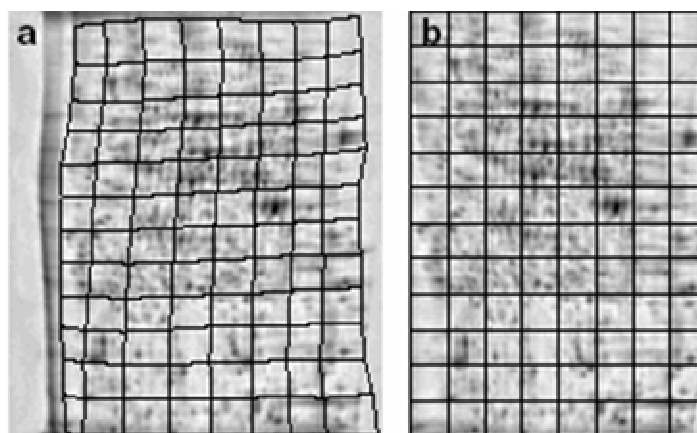
Figure 29: Aligement d'un gel (l'image a correspond au gel avant déformation, l'image b est le résultat de l'alignement avec un gel de référence)
